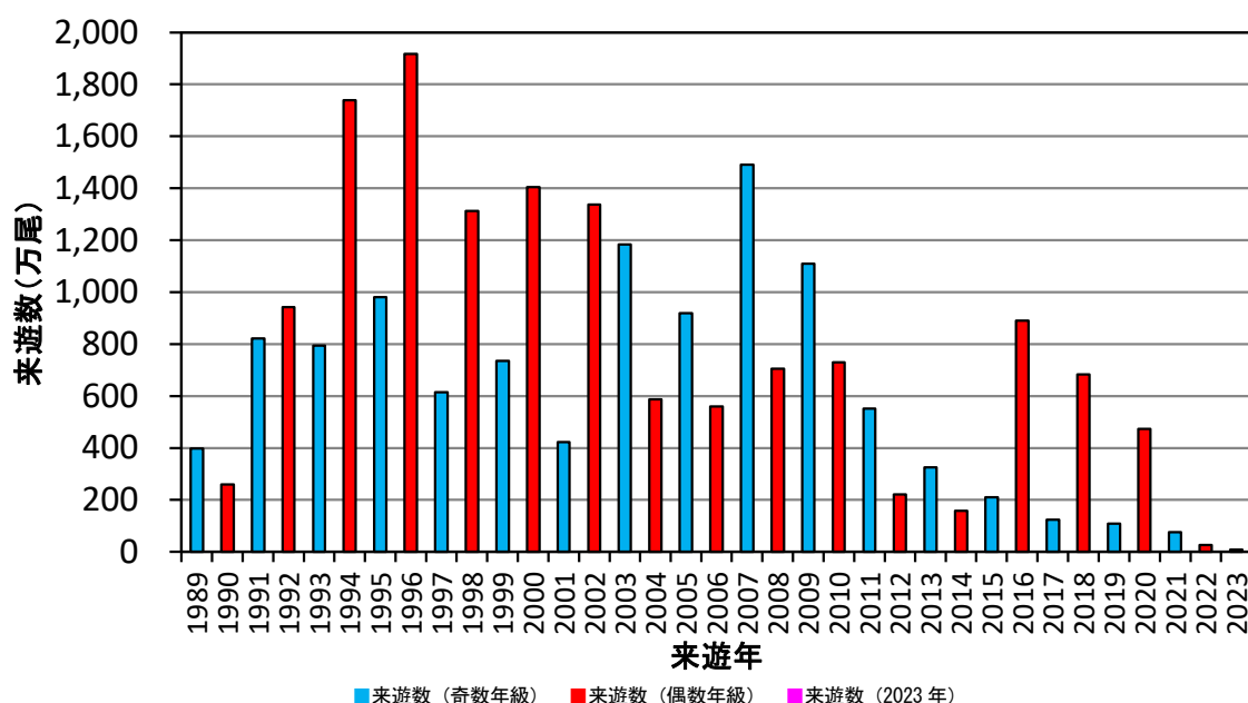
図1. 7月1日～10月31日までのカラフトマス来遊数（累計値）。2023年は速報値。
