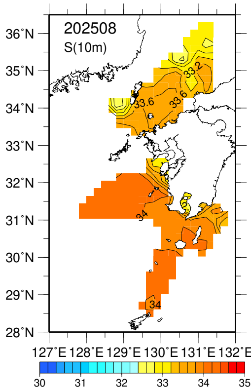
塩分(10m深).
