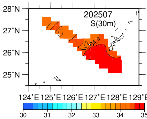
塩分(30m深).
