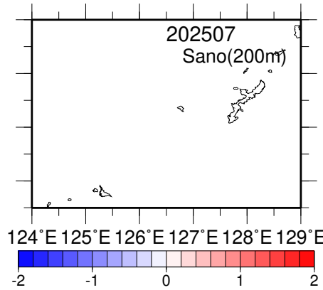
塩分平年偏差(200m深).
