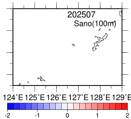
塩分平年偏差(100m深).
