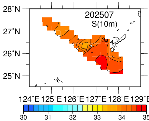
塩分(10m深).
