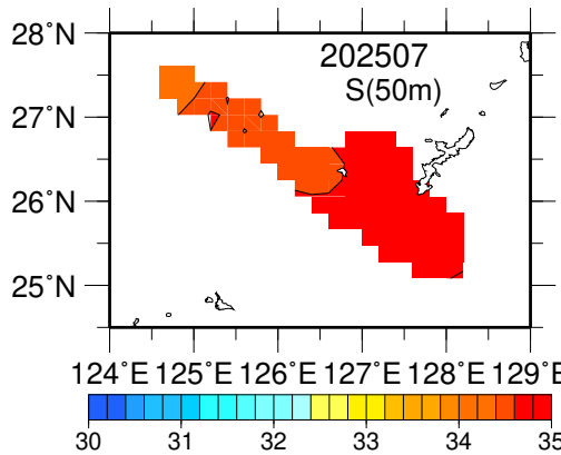
塩分(50m深).
