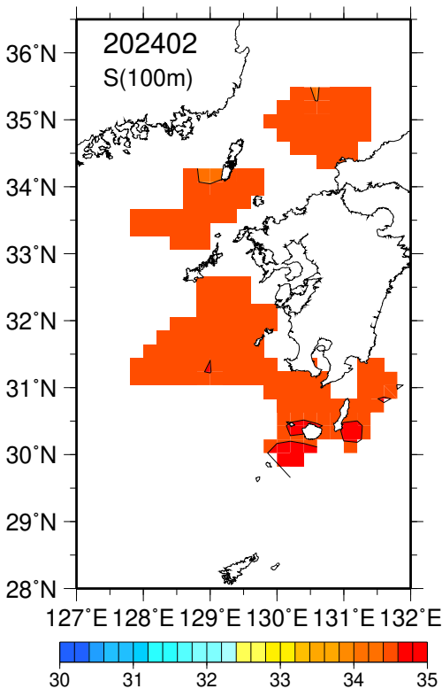
塩分(100m深).
