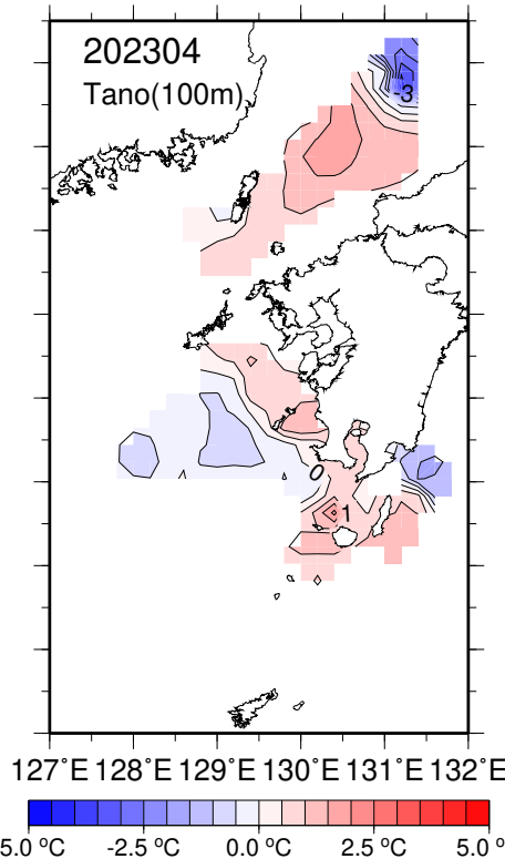
水温平年偏差(100m深).
