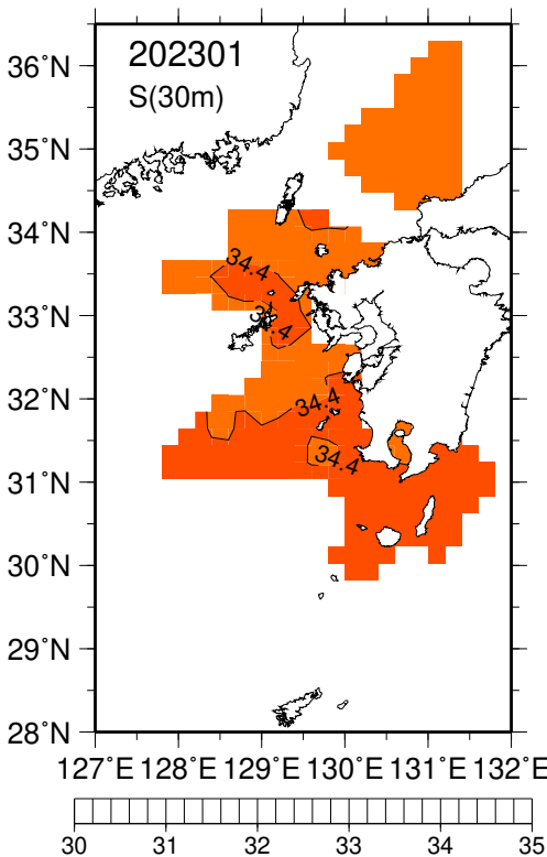
塩分(30m深).
