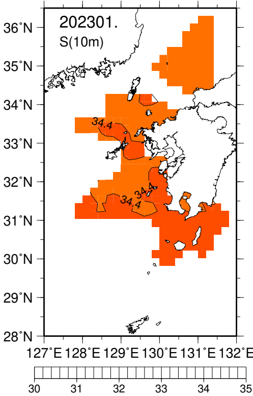
塩分(10m深).
