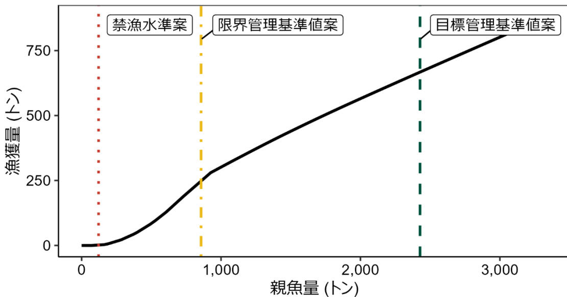
補足図 4-1. 漁獲管理規則案 目標管理基準値案 (SBtarget) は HS 再生産関係に基づき算出した SB_{msy} である。限界管理基準値案 (SBlimit) および禁漁水準案 (SBban) には、それぞれ標準値を用いている。調整係数 \beta には標準値である 0.8 を用いた。黒破線は F_{msy} 、灰色破線は 0.8F_{msy} 、黒太線は HCR、赤破線は禁漁水準案、黄破線は限界管理基準値案、緑破線は目標管理基準値案を示す。a) は縦軸を漁獲圧にした場合、b) は縦軸を漁獲量で表した場合である。b) については、漁獲する年の年齢組成によって漁獲量は若干異なるが、ここでは平衡状態における平均的な年齢組成の場合の漁獲量を示した。
