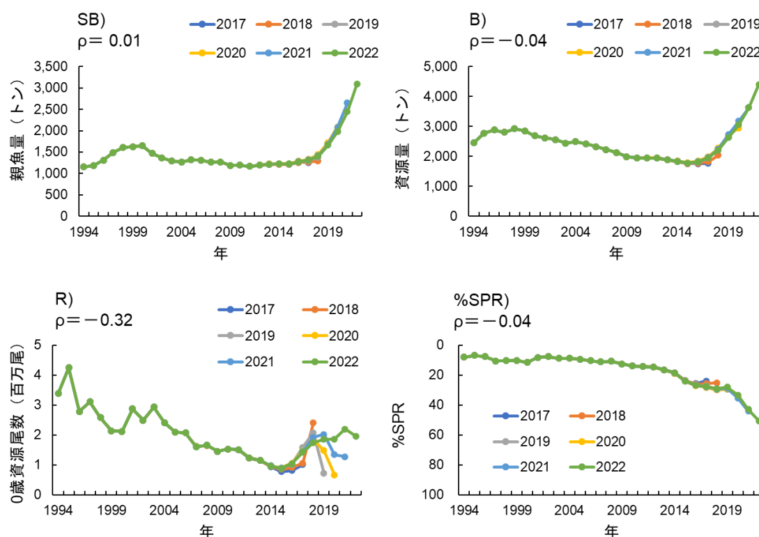
補足図 2-2. 親魚量 (SB)、資源量 (B)、0 歳資源尾数 (R)、%SPR のレトロスペクティブ解析結果 凡例の数字は VPA 最終年を示す。
