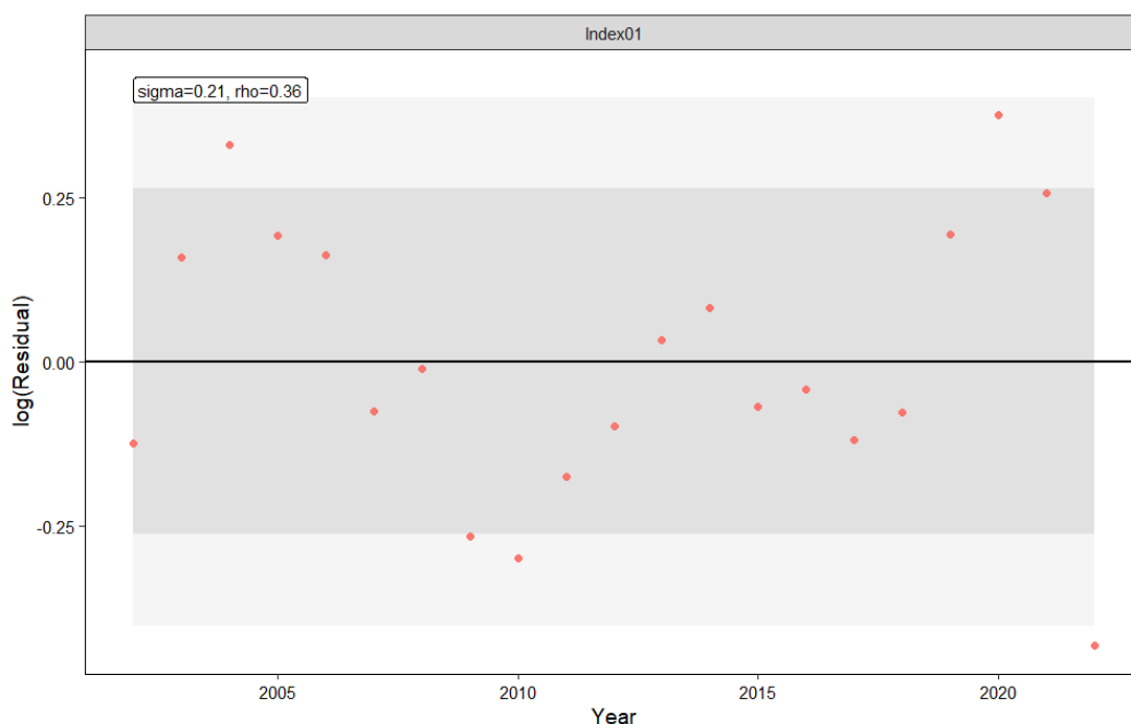
補足図 2-1. チューニング VPA における残差プロット
