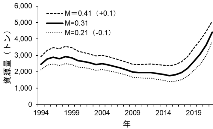
図 4-9. 自然死亡係数 M の値による資源量の感度解析 (チューニングの非線形係数 b を 1.23 に固定した場合)
