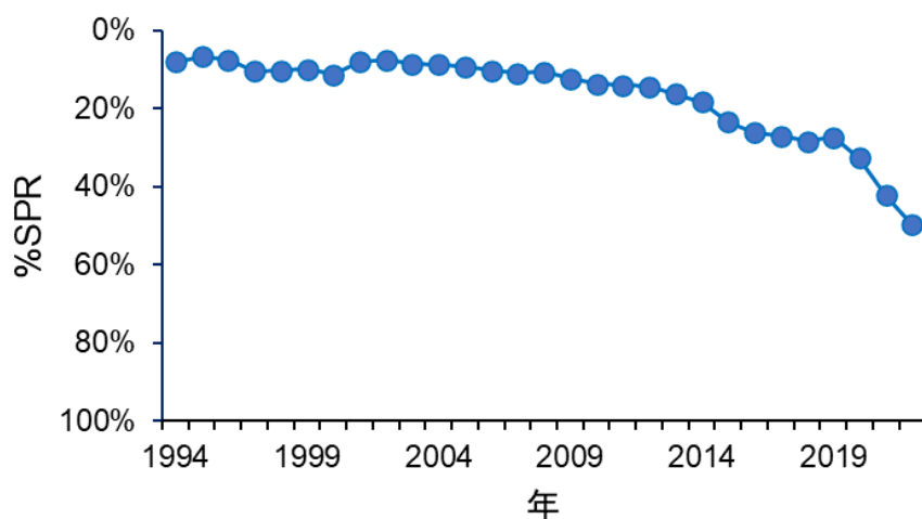
図 4-15. 各年における%SPR 値の経年推移 %SPR は漁獲がないときの親魚量に対する漁獲があるときの親魚量の割合を示し、F が高い（低い）と%SPR は小さく（大きく）なる。
