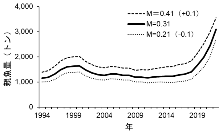
図 4-10. 自然死亡係数 M の値による親魚量の感度解析 (チューニングの非線形係数 b を 1.23 に固定した場合)
