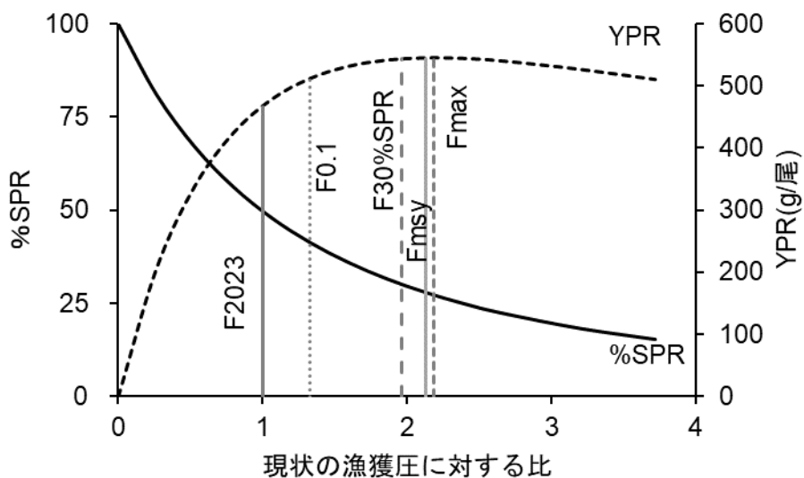
図 4-16. 現状の漁獲圧 (F2023) に対する YPR、%SPR の関係
