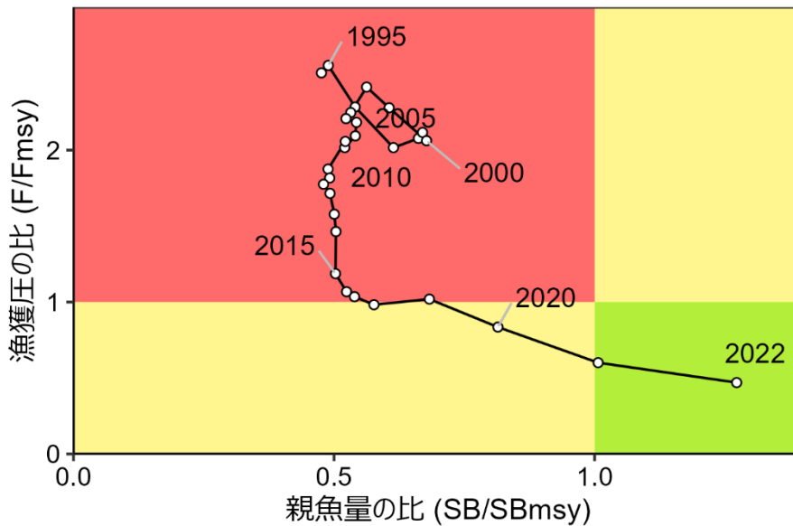
図 4-18. 神戸プロット
