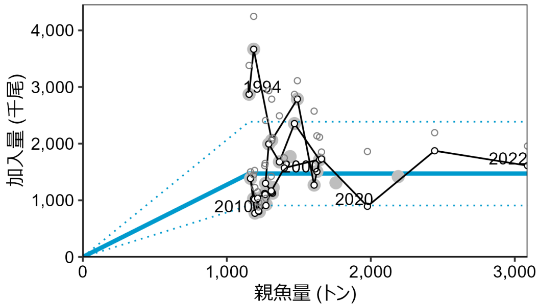
図 4-17. 親魚量と加入量の関係 青実線は本系群で適用した再生産関係式であり、上下の点線は、仮定されている再生産関係において観察データの 90%が含まれると推定される範囲である。再生産関係式のパラメータは令和 3 年 9 月に開催された「管理基準値等に関する研究機関会議」で示された値（山下ほか 2021）に基づき、塗りつぶしの灰色丸印はこの再生産関係推定時の親魚量と加入量を示す。白抜き丸印は今年度評価において推定された 1994～2022 年の親魚量と加入量を示し、黒色は天然のみ、灰色は種苗放流を加味した加入量である。図中の数字は加入群の年級（生まれ年）を示す。
