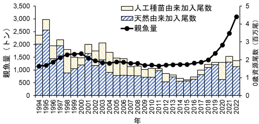
図 4.5. 親魚量および加入尾数の推移
