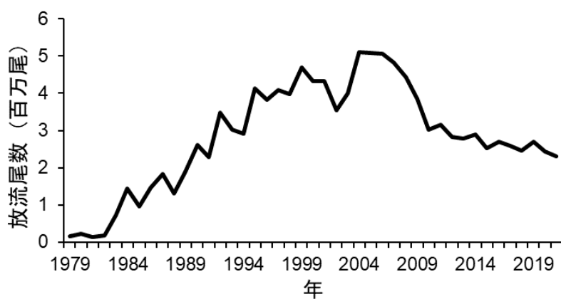
図 4-14. 1979 年以降の人工種苗放流尾数の推移
