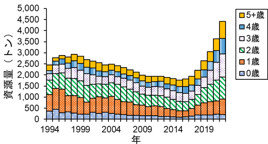
図 4.4. 年齢別資源量の推移
