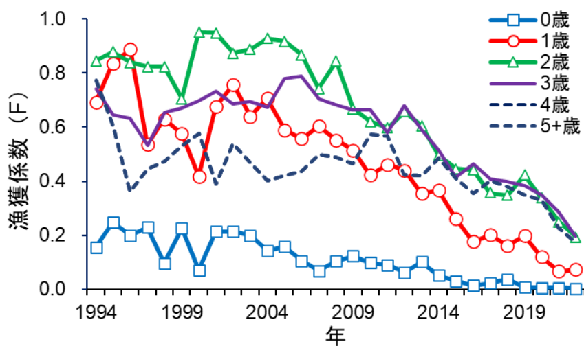
図 4-12. 年齢別漁獲係数 F の推移
