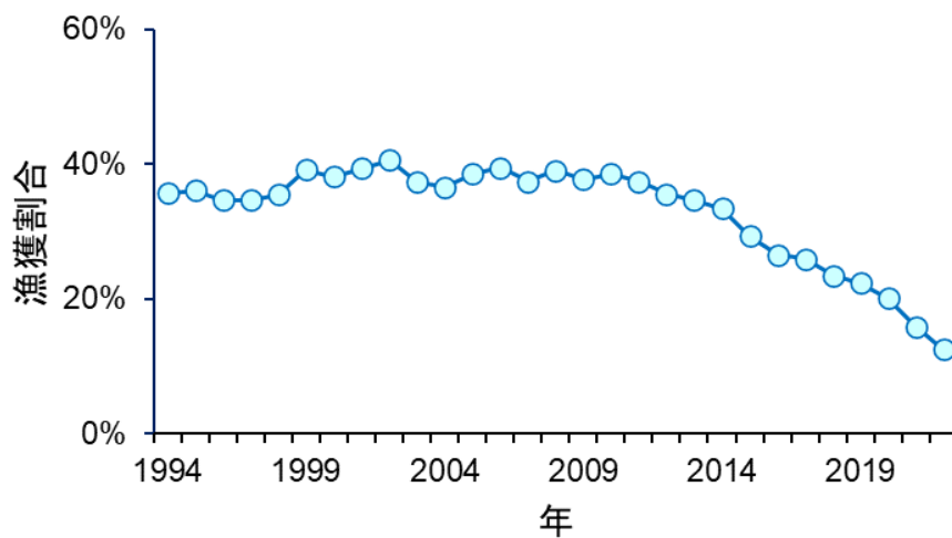
図 4-13. 漁獲割合の推移
