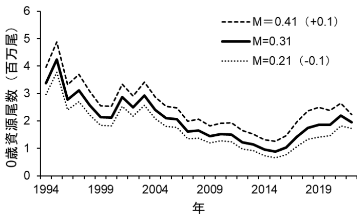
図 4-11. 自然死亡係数 M の値による 0 歳資源尾数の感度 (チューニングの非線形係数 b を 1.23 に固定した場合)
