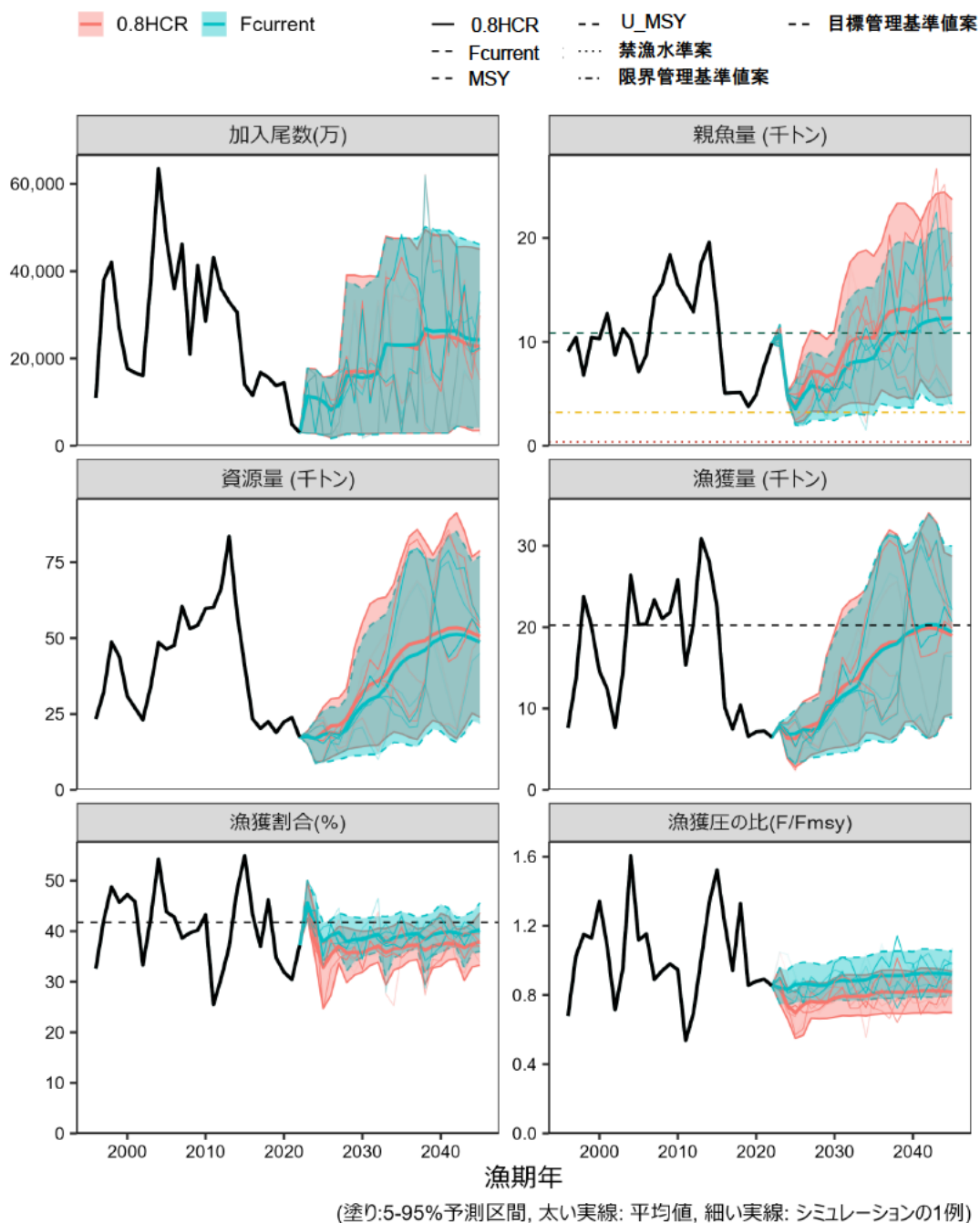
補足図 4-2. 漁獲管理規則 (HCR) 案を用いた将来予測 (赤線) と現状の漁獲圧で漁獲を続けた場合の将来予測 (青線)
