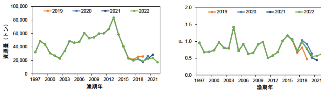
補足図 2-2. 資源量 (左) および F (右) のレトロスペクティブ解析結果
