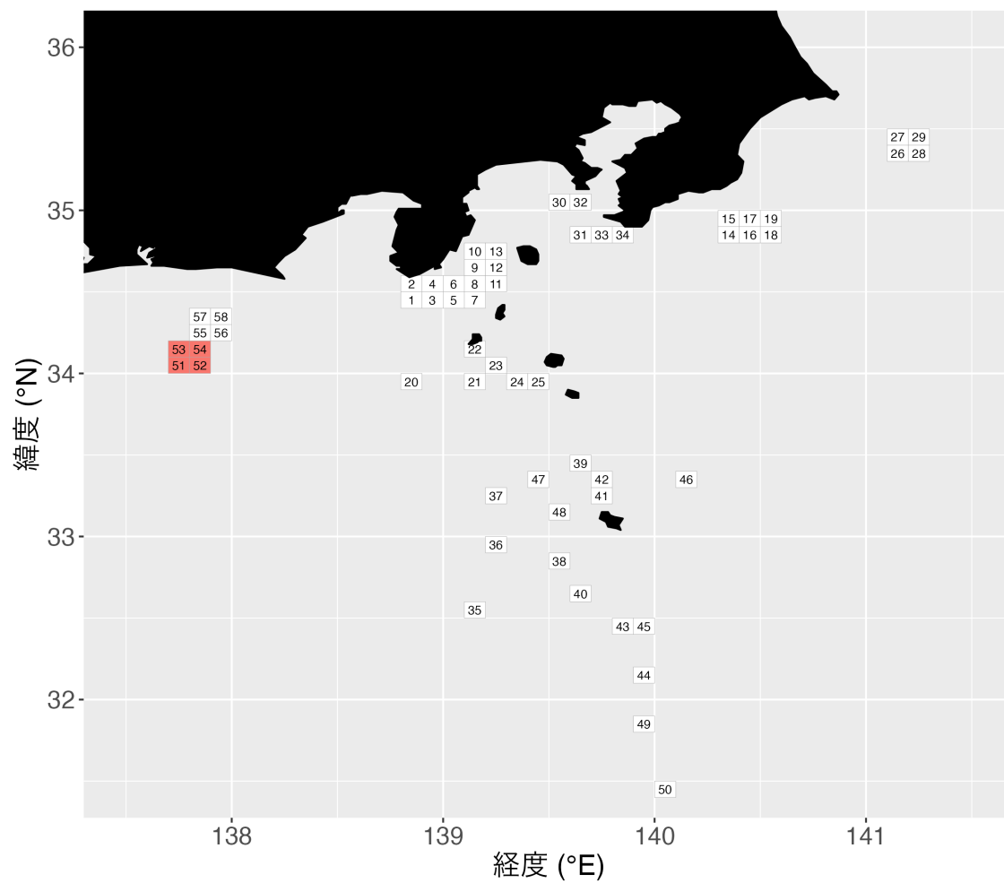
図 1. FRA-ROMS II再解析値の抽出を行う漁場位置の候補 緯度経度 0.1°グリッドごとにデータを抽出。御前崎地区は51～54番のグリッドを使用。
