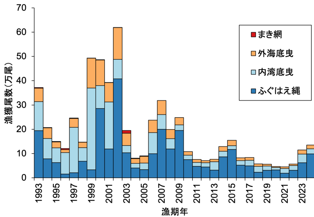
図 3-4. 漁業種類別漁獲尾数の推移
