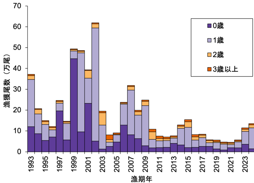
図 3-3. 年齢別漁獲尾数の推移
