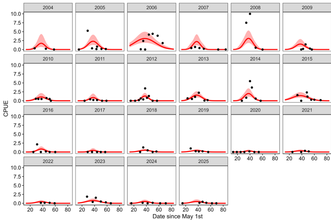
補足図 3-5. サーフネット調査 CPUE の観測値（黒点）と予測値（赤線）の推移（横軸は 5 月 1 日からの日数）
