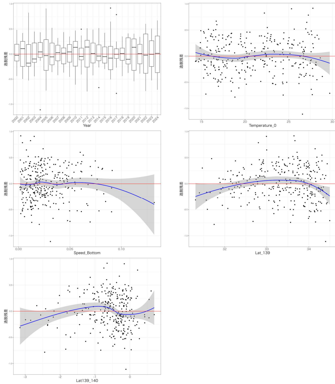
図 6. ベストモデルの層別逸脱残差 Temperature_0、Speed_Bottom、Lat_139、Lat139_140 に関する残差図の青線と灰帯は、残差にフィッティングさせた平滑化曲線 (loess) と、その 95%信頼区間を示す。
