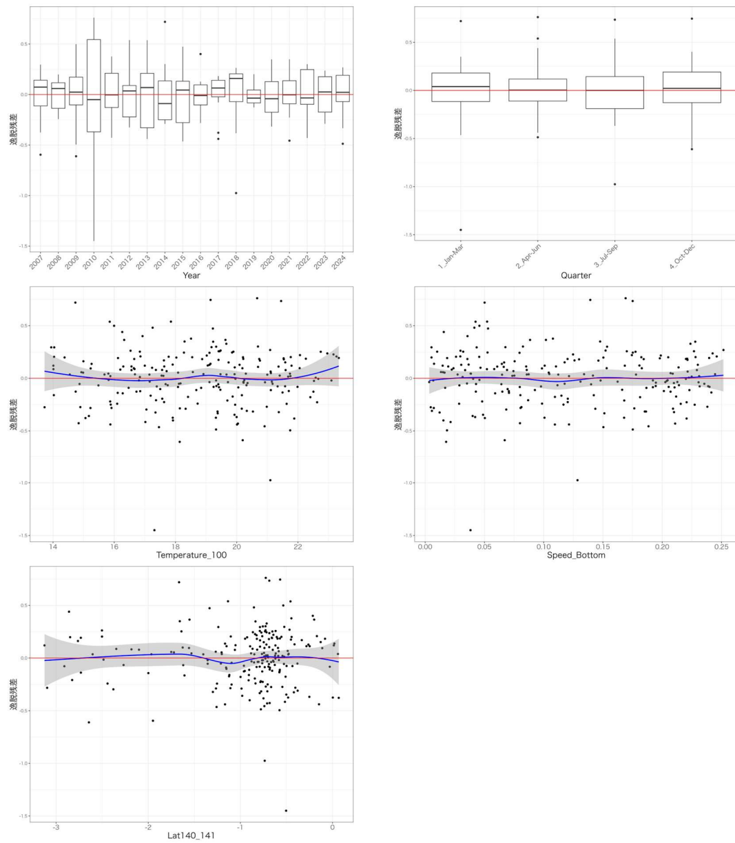
図 6. ベストモデルの層別逸脱残差 Temperature_100、Speed_Bottom、Lat140_141 に関する残差図の青線と灰帯は、残差にフィッティングさせた平滑化曲線 (loess) と、その 95% 信頼区間を示す。
