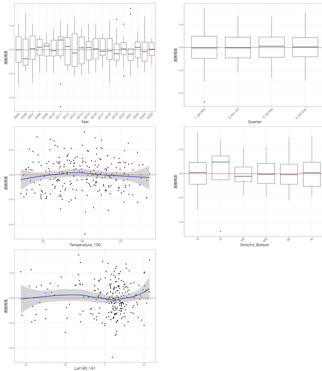
図 6. ベストモデルの層別逸脱残差 Temperature_100、Lat140_141 に関する残差図の青線と灰帯は、残差にフィッティングさせた平滑化曲線 (loess) と、その 95%信頼区間を示す。
