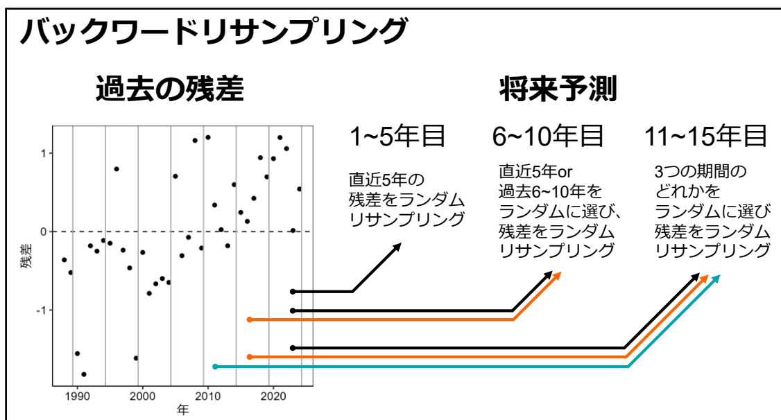
補足図 2-1. バックワードリサンプリングの概念図（SC 補足図 5-1）
