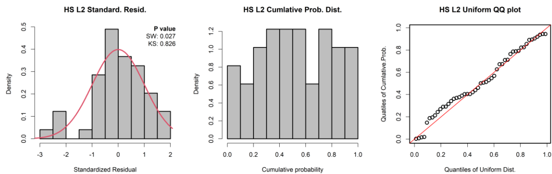
補足図 1-3. ホッケー・スティック型を仮定し再生産関係期間で分けたモデルを最小二乗法で当てはめた場合の標準化残差のヒストグラムと正規性テスト結果（左図）、残差の累積確率密度のヒストグラム（中央図）、および一様分布を仮定した QQ プロット（右図）
