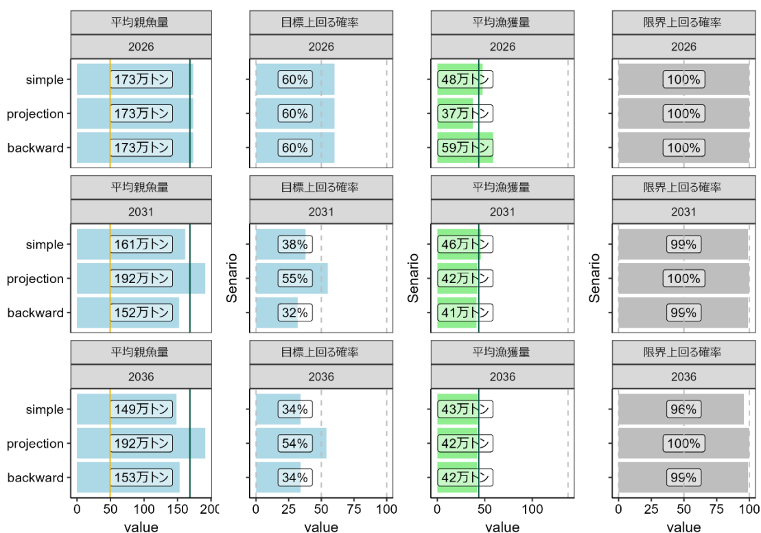
補足図 4-2. 通常加入期において真の再生産関係が RI 型であるときに、HS 型の再生産関係を適用した場合の 2026 年、2031 年、2036 年の平均親魚量、目標管理基準値案を上回る確率、平均漁獲量、限界管理基準値案を上回る確率 目標管理基準値案、限界管理基準値案は真の再生産関係である RI 型の管理基準値案を示す。simple は真の再生産関係が RI 型であるときに、HS 型の再生産関係を適用した場合の将来予測、projection は真の再生産関係が RI 型であるときに、RI 型の再生産関係を適用した場合の将来予測、backward は simple と同じだが ABC 計算時に加入量の誤差に残差のバックワードリサンプリングを適用した場合の将来予測を示す。
