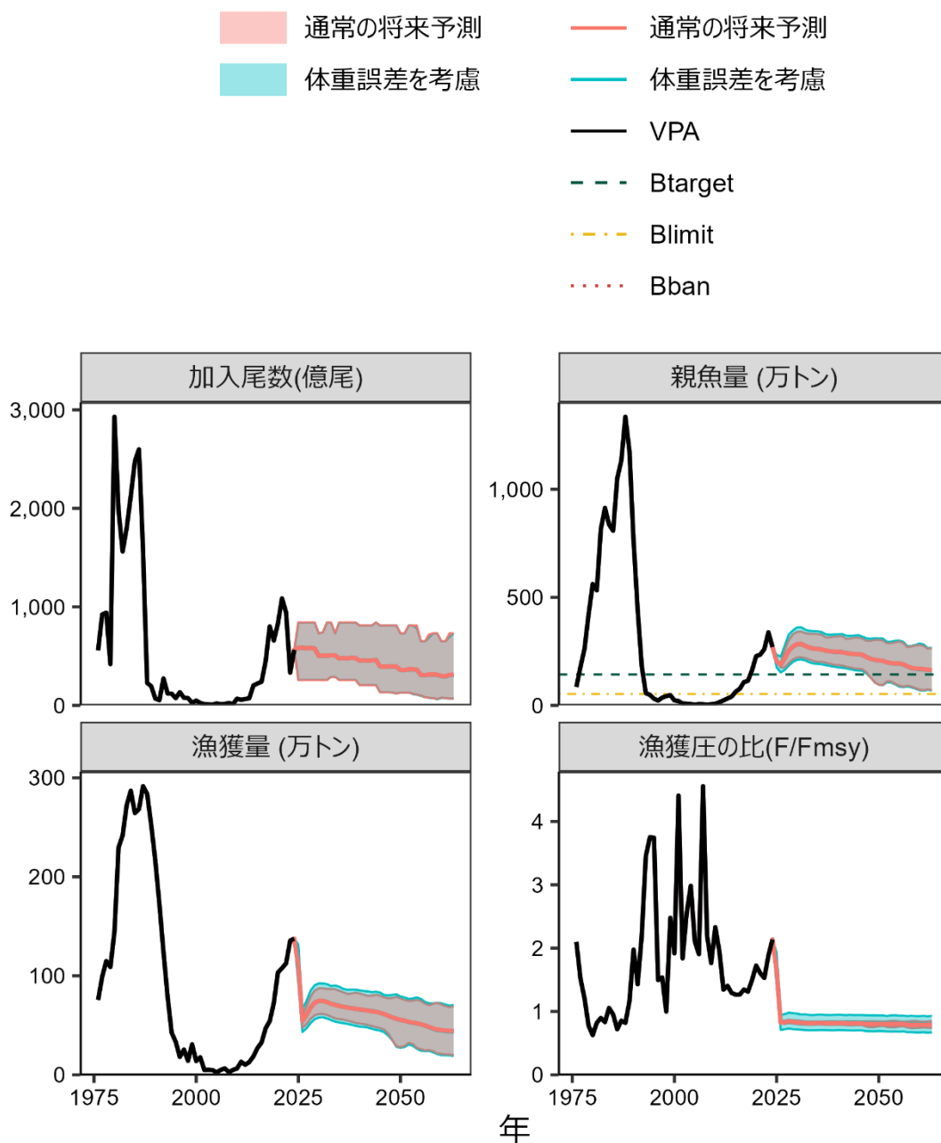
補足図 9-1. 体重の誤差を考慮した将来予測に基づく将来予測
