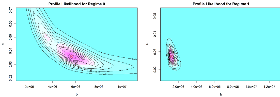
補足図 1-8. ホッケー・スティック型を仮定し再生産関係期間で分けたモデルを最小二乗法で当てはめた場合の推定パラメータのプロファイル尤度 ×印は推定されたパラメータ値における尤度に相当する。左図は高加入期 (Regime0)、右図は通常加入期 (Regime1) の結果を示す。
