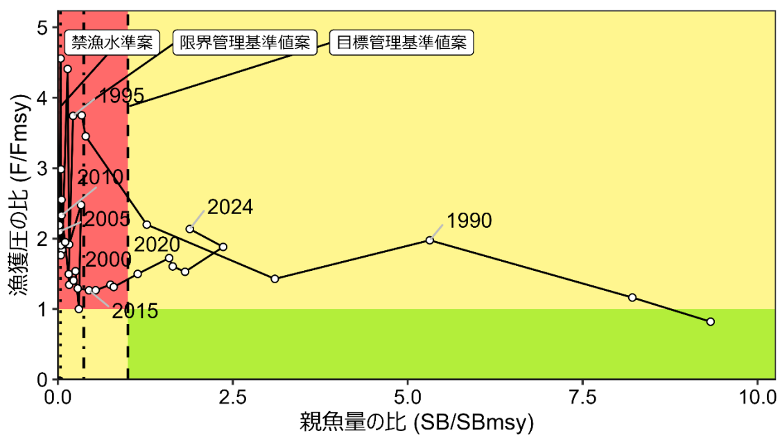
図4. 神戸プロット (SC 補足図 3-1)
