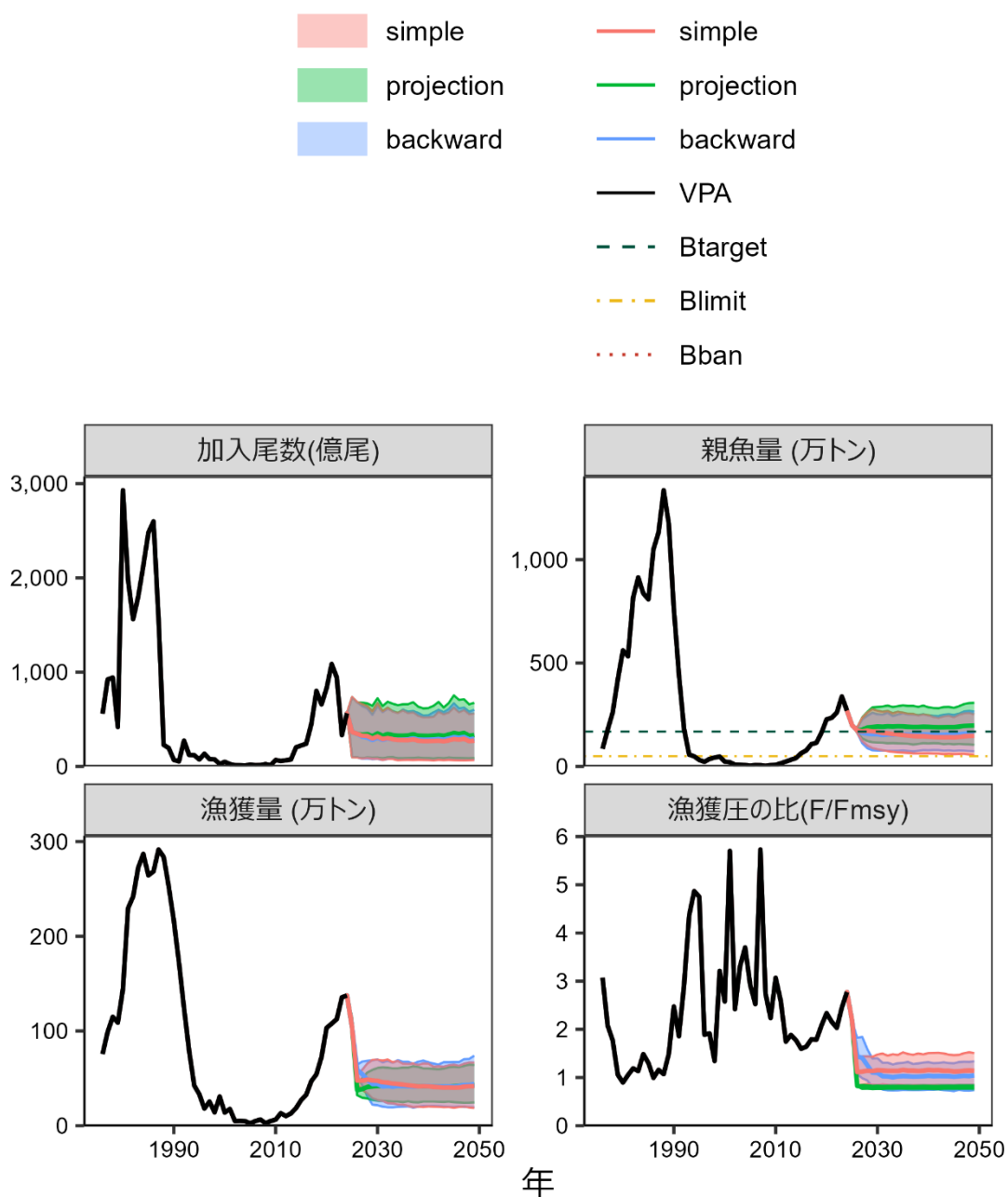
補足図 4-1. 通常加入期において真の再生産関係が RI 型であるときに、HS 型の再生産関係を適用した場合の加入尾数、親魚量、漁獲量、漁獲圧の比の将来予測 目標管理基準値案、限界管理基準値案は真の再生産関係である RI 型の管理基準値案を示す。 simple は真の再生産関係が RI 型であるときに、HS 型の再生産関係を適用した場合の将来予測、 projection は真の再生産関係が RI 型であるときに、RI 型の再生産関係を適用した場合の将来予測、 backward は simple と同じだが ABC 計算時に加入量の誤差に残差のバックワードリサンプリングを適用した場合の将来予測を示す。
