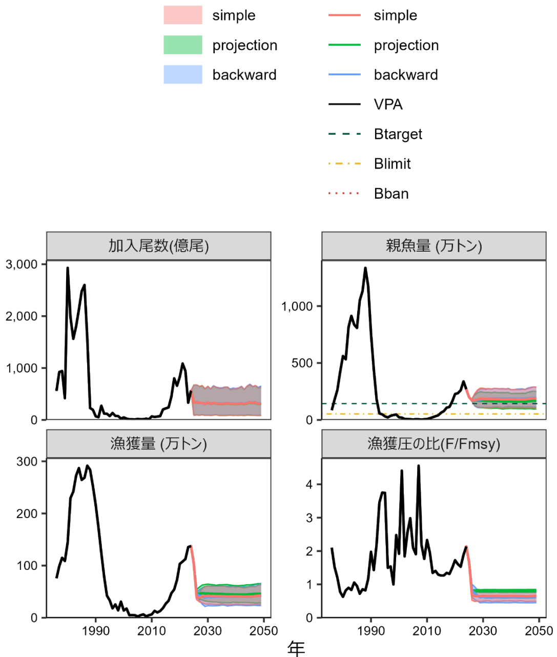
補足図 4-3. 通常加入期において真の再生産関係が HS 型であるときに、RI 型の再生産関係を適用した場合の加入尾数、親魚量、漁獲量、漁獲圧の比の将来予測 目標管理基準値案、限界管理基準値案は真の再生産関係である HS 型の管理基準値案を示す。simple は真の再生産関係が HS 型であるときに、RI 型の再生産関係を適用した場合の将来予測、projection は真の再生産関係が HS 型であるときに、HS 型の再生産関係を適用した場合の将来予測、backward は simple と同じだが ABC 計算時に加入量の誤差に残差のバックワードリサンプリングを適用した場合の将来予測を示す。
