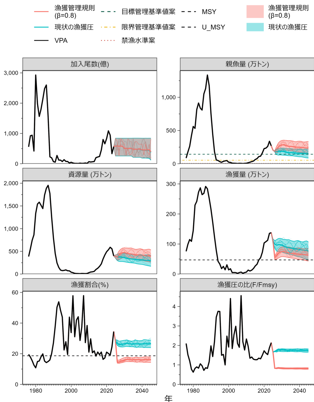
図 6. 管理基準値案に基づく漁獲管理規則案を用いた将来予測（赤色）と現状の漁獲圧（F2022-2024）で漁獲を続けた場合の将来予測（緑色）の比較
