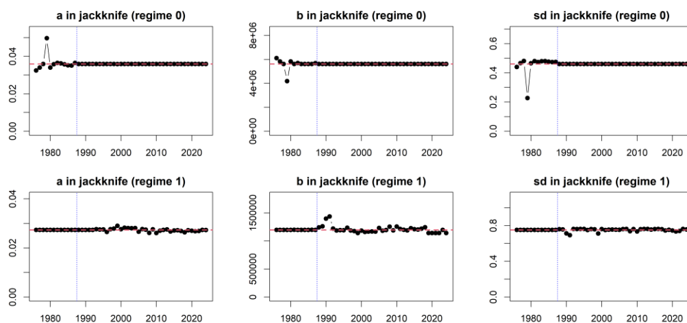
補足図 1-5. ホッケー・スティック型を仮定し再生産関係期間で分けたモデルを最小二乗法で当てはめた場合のジャックナイフ解析でのパラメータ別の影響 上段は高加入期（Regime0）、下段は通常加入期（Regime1）の結果を示す。青色の点線は再生産関係が切り替わる時点を表している。
