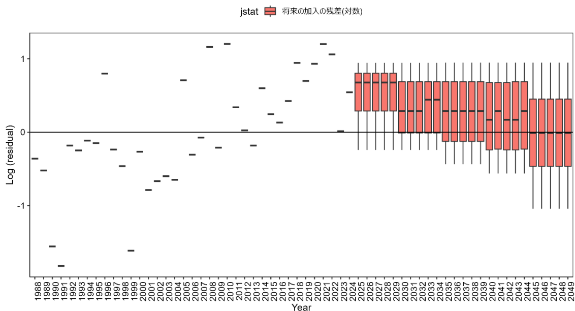
補足図 2-2. 加入量の予測値に対する観測値の残差（1988～2024 年）と将来予測において用いられた残差（SC 補足図 5-2）
