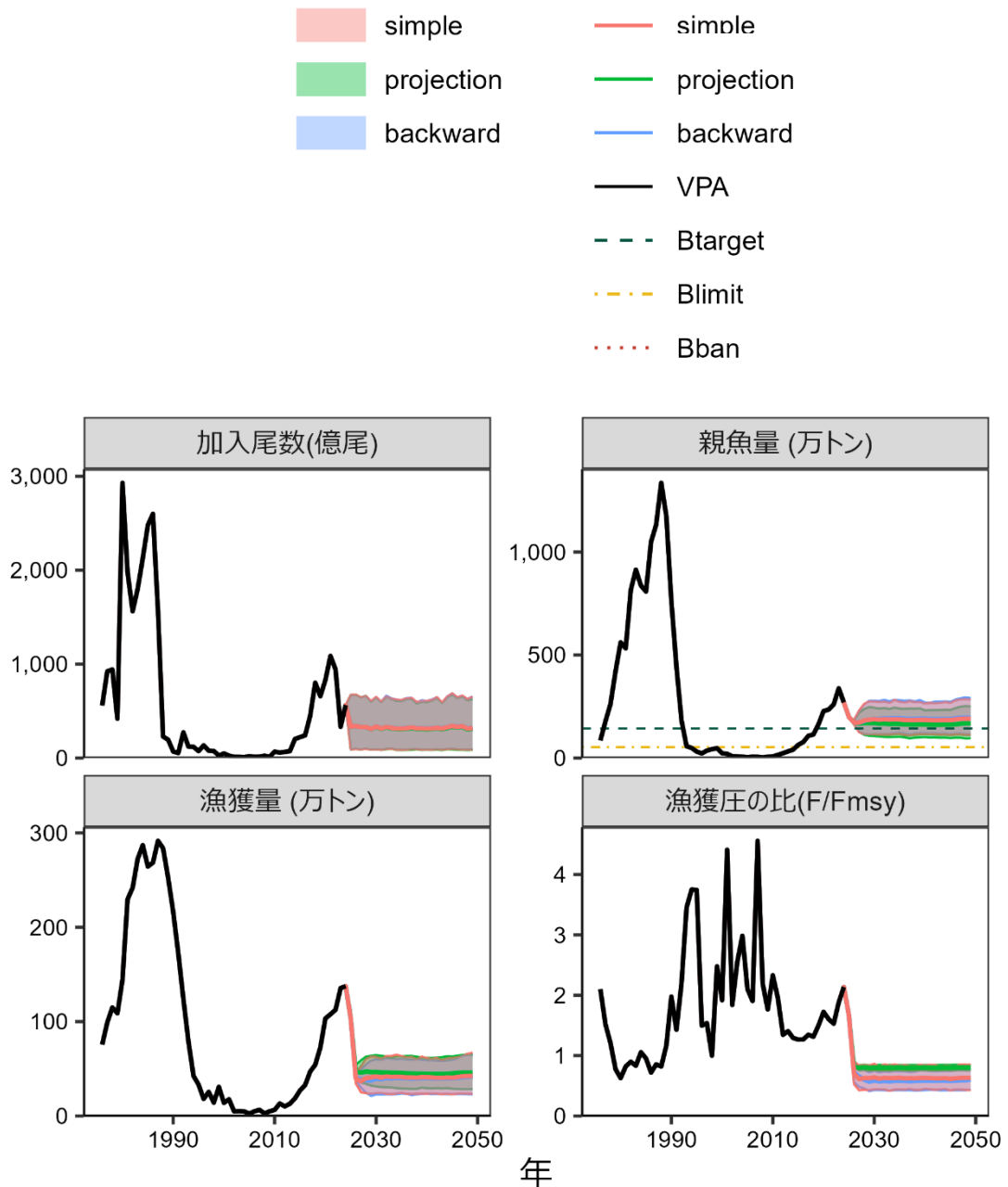
補足図 5-3. 真の再生産関係が通常加入期の HS 型であるときに、全期間の HS 型の再生産関係を適用した場合の加入尾数、親魚量、漁獲量、漁獲圧の比の将来予測 目標管理基準値案、限界管理基準値案は真の再生産関係である通常加入期の HS 型の管理基準値案を示す。simple は真の再生産関係が通常加入期の HS 型であるときに、全期間の HS 型の再生産関係を適用した場合の将来予測、projection は真の再生産関係が通常加入期の HS 型であるときに、通常加入期の HS 型の再生産関係を適用した場合の将来予測、backward は simple と同じだが ABC 計算時に加入量の誤差に残差のバックワードリサンプリングを適用した場合の将来予測を示す。
