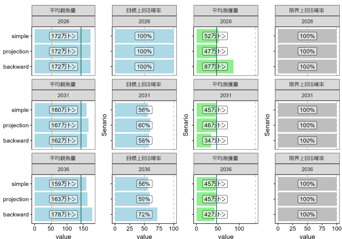
補足図 6-4. 真の再生産関係が通常加入期の HS 型であるときに、高加入期の HS 型の再生産関係を想定して管理を行った場合の 2026 年、2031 年、2036 年の平均親魚量、目標管理基準値案を上回る確率、平均漁獲量、限界管理基準値案を上回る確率。目標管理基準値案、限界管理基準値案は真の再生産関係である通常加入期の HS 型の管理基準値案を示す。simple は真の再生産関係が通常加入期の HS 型であるときに、高加入期の HS 型の再生産関係を適用した場合の将来予測、projection は真の再生産関係が通常加入期の HS 型であるときに、通常加入期の HS 型の再生産関係を適用した場合の将来予測、backward は simple と同じだが ABC 計算時に加入量の誤差に残差のバックワードリサンプリングを適用した場合の将来予測を示す。
