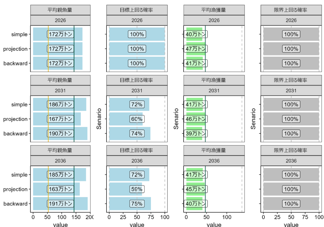
補足図 5-4. 真の再生産関係が通常加入期の HS 型であるときに、全期間の HS 型の再生産関係を適用した場合の 2026 年、2031 年、2036 年の平均親魚量、目標管理基準値案を上回る確率、平均漁獲量、限界管理基準値案を上回る確率
