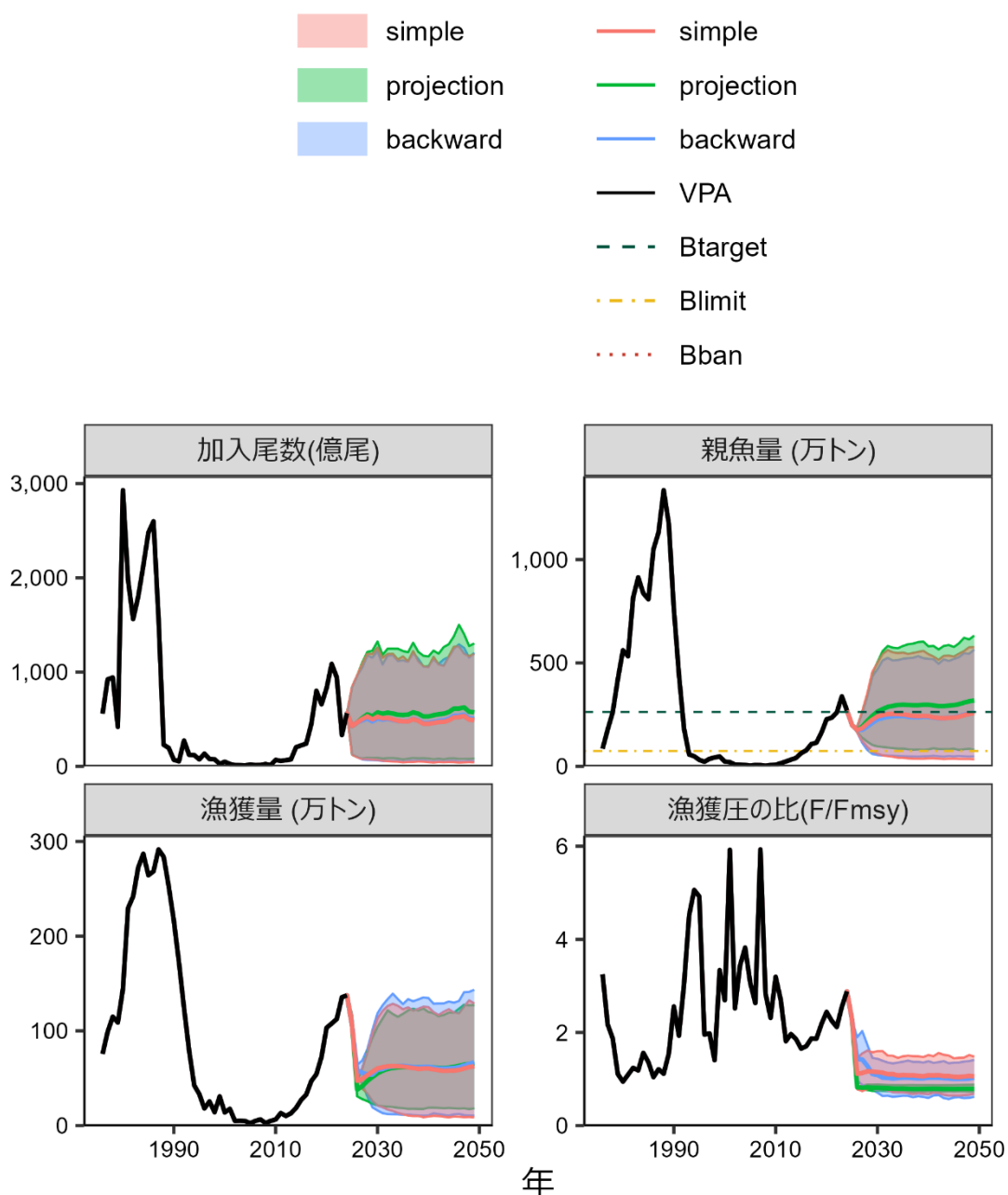
補足図 5-1. 真の再生産関係が全期間の HS 型であるときに、通常加入期の HS 型の再生産関係を適用した場合の加入尾数、親魚量、漁獲量、漁獲圧の比の将来予測 目標管理基準値案、限界管理基準値案は真の再生産関係である全期間の HS 型の管理基準値案を示す。simple は真の再生産関係が全期間の HS 型であるときに、通常加入期の HS 型の再生産関係を適用した場合の将来予測、projection は真の再生産関係が全期間の HS 型であるときに、全期間の HS 型の再生産関係を適用した場合の将来予測、backward は simple と同じだが ABC 計算時に加入量の誤差に残差のバックワードリサンプリングを適用した場合の将来予測を示す。
