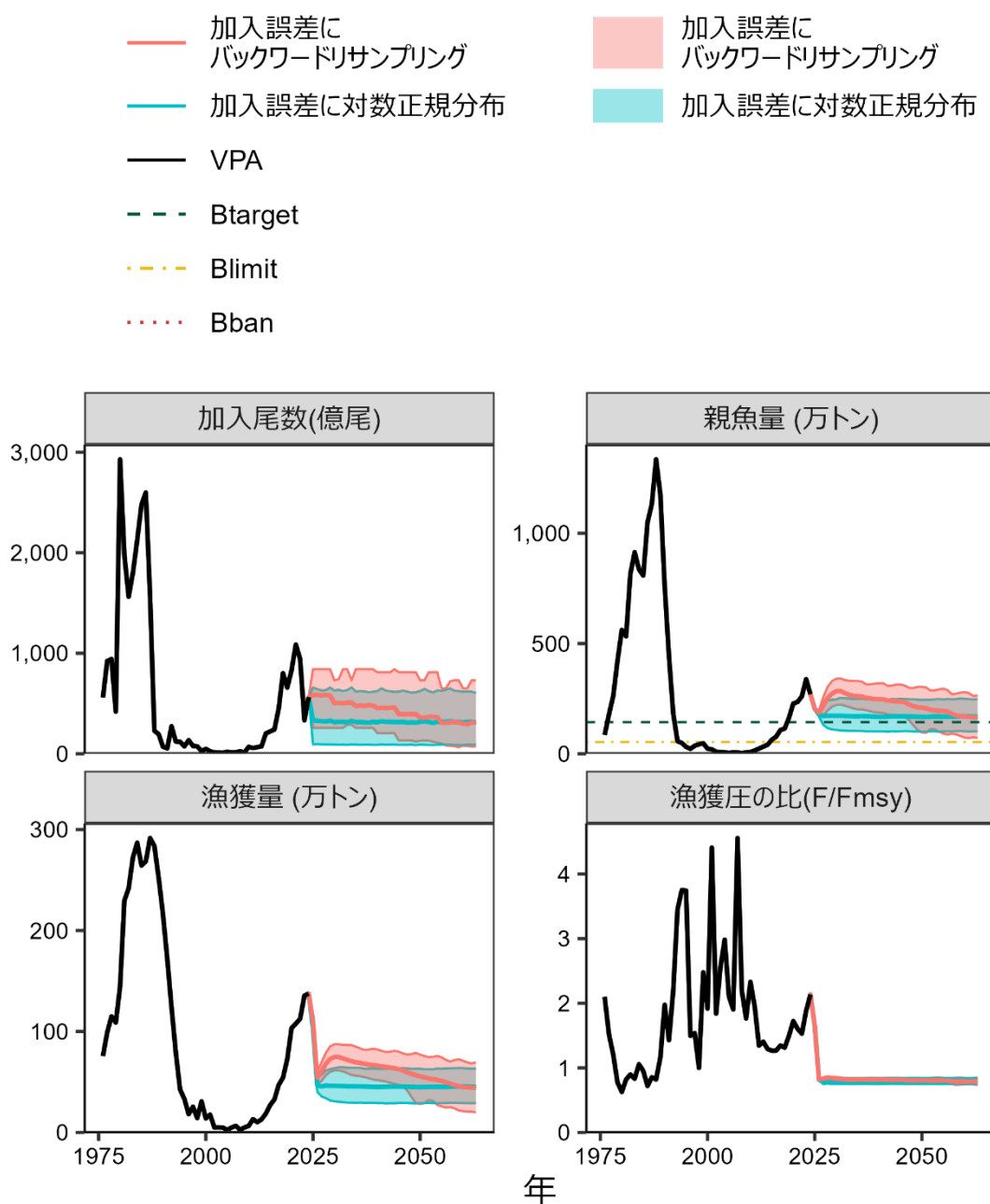
補足図 7-1. 加入量の誤差にバックワードリサンプリングを適用した将来予測と対数正規分布を適用した将来予測
