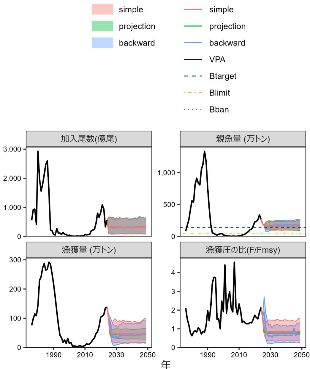
補足図 6-3. 真の再生産関係が通常加入期の HS 型であるときに、高加入期の HS 型の再生産関係を想定して管理を行った場合の加入尾数、親魚量、漁獲量、漁獲圧の比の将来予測
