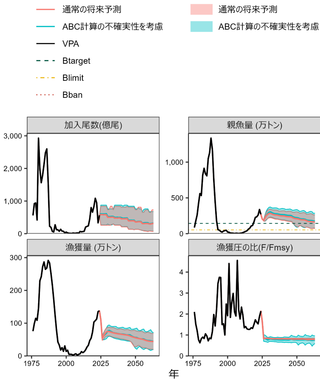
補足図 8-1. ABC 計算の不確実性を考慮した MSE に基づく将来予測
