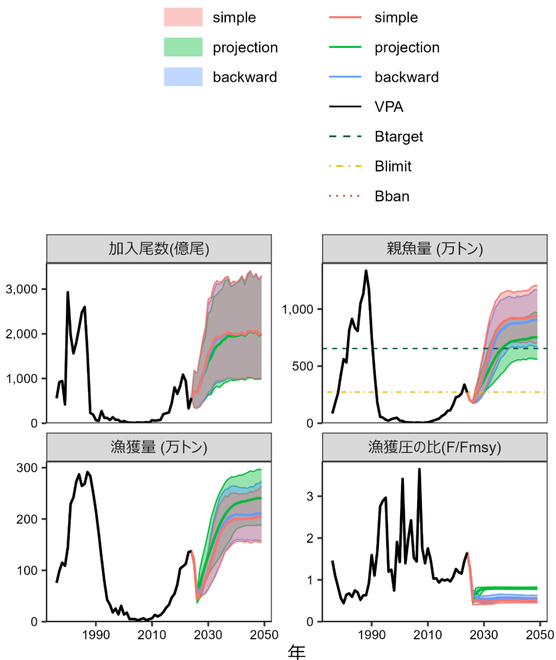
補足図 6-1. 真の再生産関係が高加入期の HS 型であるときに、通常加入期の HS 型の再生産関係を想定して管理を行った場合の加入尾数、親魚量、漁獲量、漁獲圧の比の将来予測
