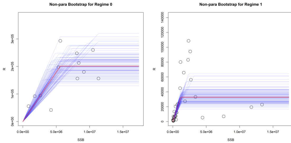
補足図 1-6. ホッケー・スティック型を仮定し再生産関係期間で分けたモデルを最小二乗法で当てはめた場合の残差ブートストラップ解析の結果 赤線は元データでの推定値、青線はノンパラメトリックブートストラップでの推定値である。分析に使用した親魚量・加入尾数を丸印で示す。左図は高加入期 (Regime0)、右図は通常加入期 (Regime1) の結果を示す。
