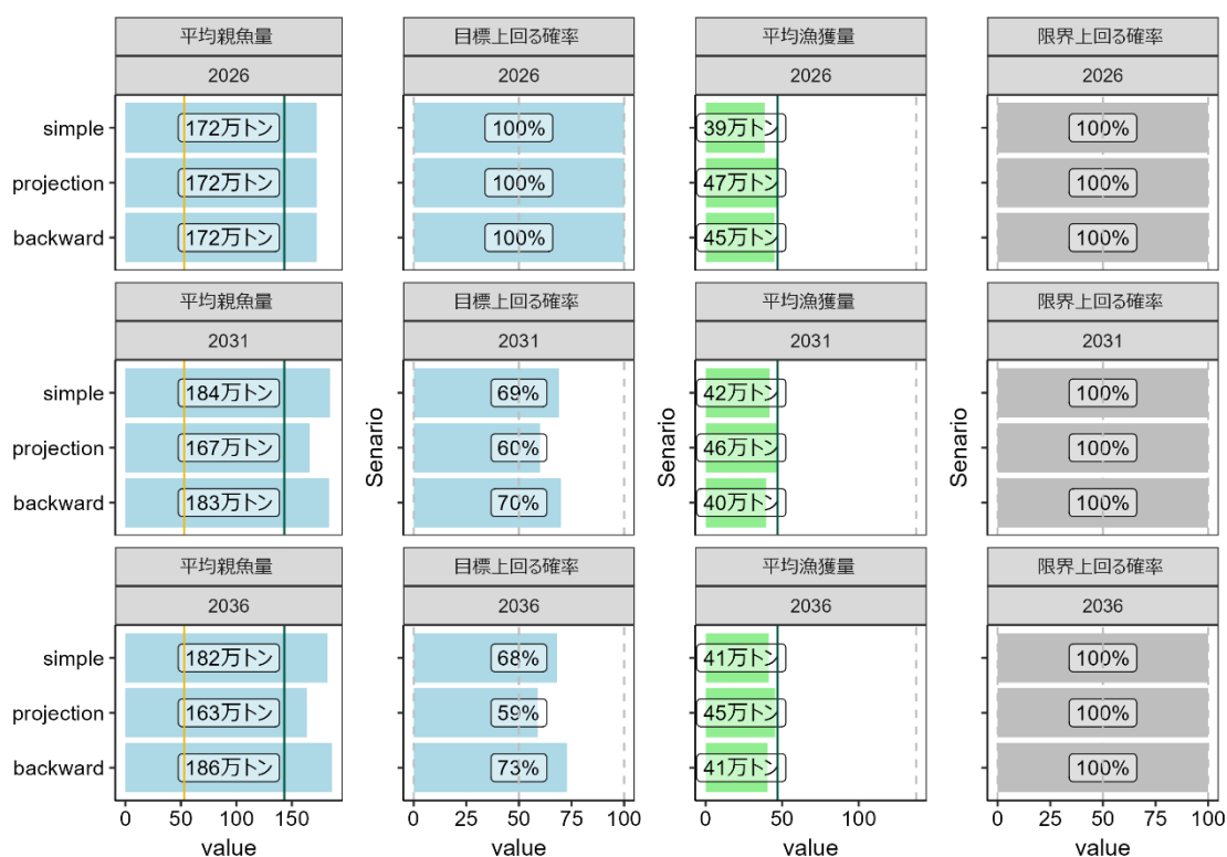
補足図 4-4. 通常加入期において真の再生産関係が HS 型であるときに、RI 型の再生産関係を適用した場合の 2026 年、2031 年、2036 年の平均親魚量、目標管理基準値案を上回る確率、平均漁獲量、限界管理基準値案を上回る確率 目標管理基準値案、限界管理基準値案は真の再生産関係である HS 型の管理基準値案を示す。simple は真の再生産関係が HS 型であるときに、RI 型の再生産関係を適用した場合の将来予測、projection は真の再生産関係が HS 型であるときに、HS 型の再生産関係を適用した場合の将来予測、backward は simple と同じだが ABC 計算時に加入量の誤差に残差のバックワードリサンプリングを適用した場合の将来予測を示す。
