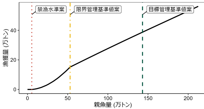
図 5. 漁獲管理規則案
