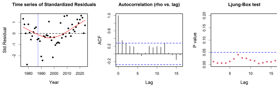
補足図 1-2. ホッケー・スティック型を仮定し再生産関係期間で分けたモデルを最小二乗法で当てはめた場合の残差トレンド（左図）、自己相関プロット（中央図）、および Ljung-Box 検定における P 値（右図）
