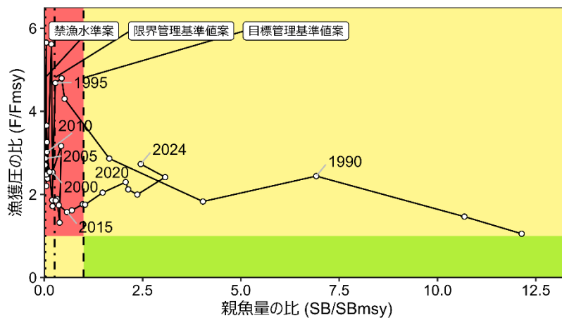
補足図 3-1. 通常加入期の管理基準値にもとづいた神戸プロット
