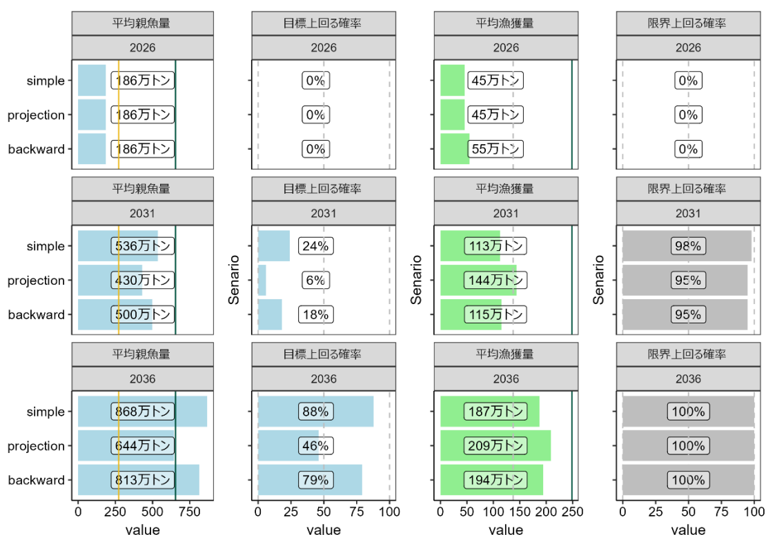
補足図 6-2. 真の再生産関係が高加入期の HS 型であるときに、通常加入期の HS 型の再生産関係を想定して管理を行った場合の 2026 年、2031 年、2036 年の平均親魚量、目標管理基準値案を上回る確率、平均漁獲量、限界管理基準値案を上回る確率。目標管理基準値案、限界管理基準値案は真の再生産関係である高加入期の HS 型の管理基準値案を示す。simple は真の再生産関係が高加入期の HS 型であるときに、通常加入期の HS 型の再生産関係を適用した場合の将来予測、projection は真の再生産関係が高加入期の HS 型であるときに、高加入期の HS 型の再生産関係を適用した場合の将来予測、backward は simple と同じだが ABC 計算時に加入量の誤差に残差のバックワードリサンプリングを適用した場合の将来予測を示す。
