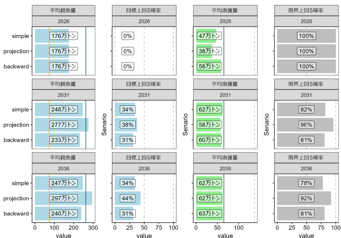
補足図 5-2. 真の再生産関係が全期間の HS 型であるときに、通常加入期の HS 型の再生産関係を適用した場合の 2026 年、2031 年、2036 年の平均親魚量、目標管理基準値案を上回る確率、平均漁獲量、限界管理基準値案を上回る確率
