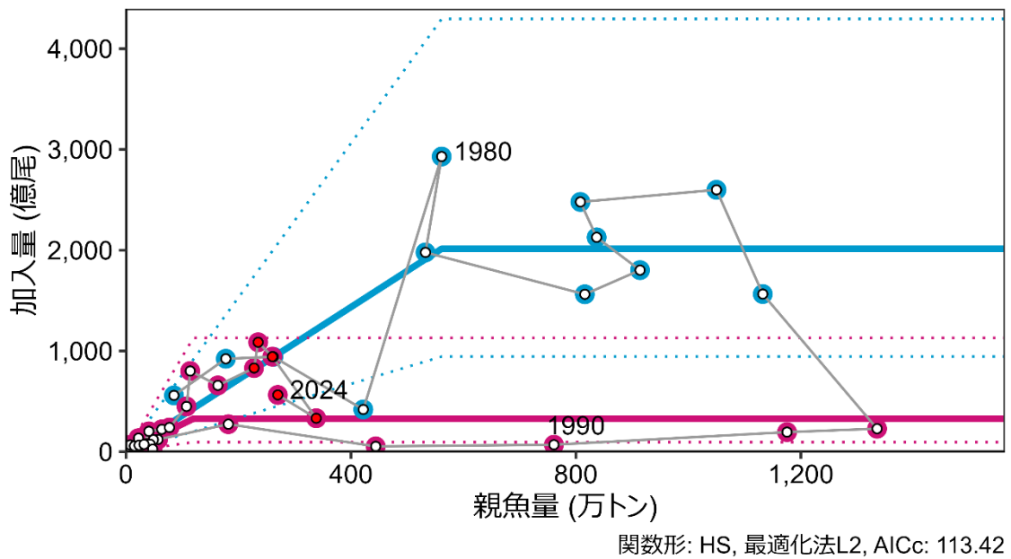
図 1. 再生産関係 (SC 図 4-9)
