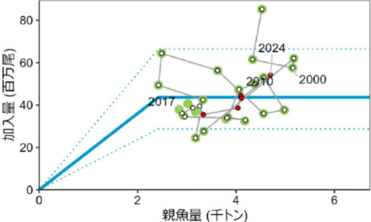
図6 再生産関係
