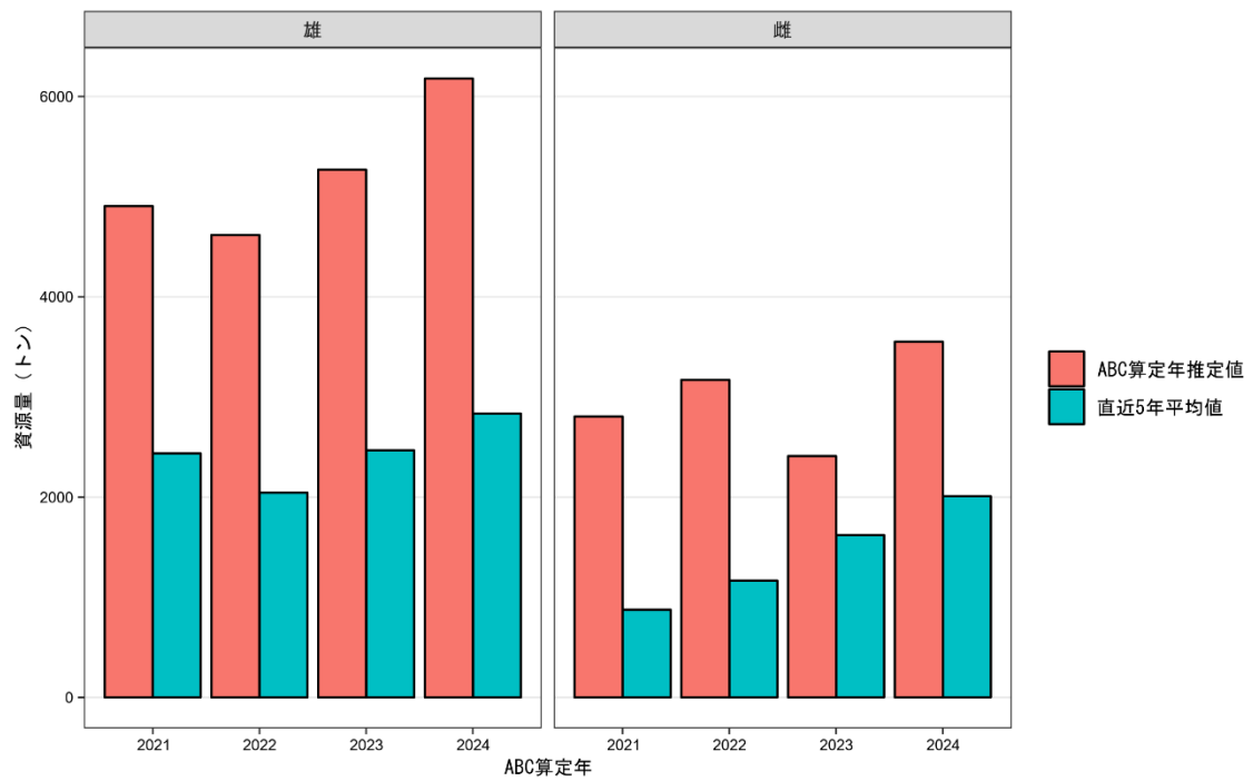
補足図 11-1. かご調査データで推定した ABC 算定年における資源量とそれに対応する直近 5 年間の資源量平均値の比較
