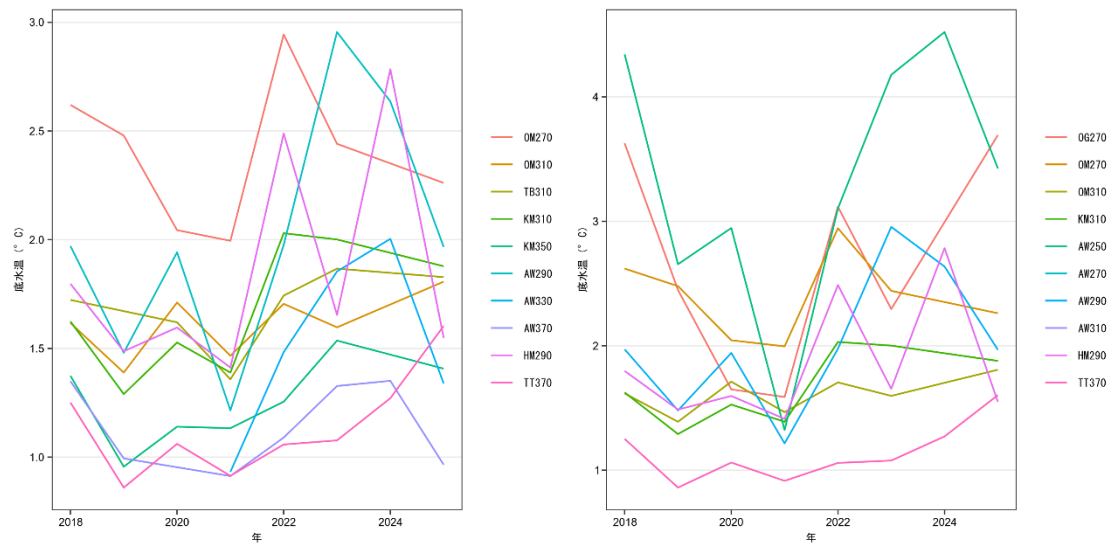
補足図 9-7. 出現密度上位 10 定点における底水温の推移（雄：左、雌：右） 定点位置は補足図 5-1 参照。雄：甲幅 90 mm 以上、雌：11 齢に関する密度。
