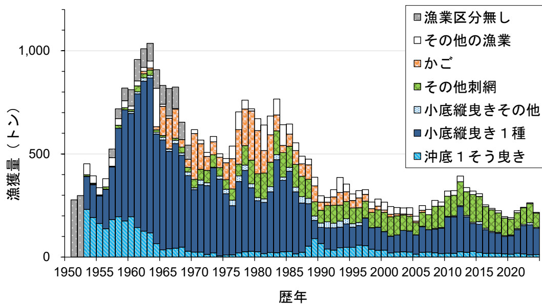
図 3-1. ズワイガニの漁業種類別漁獲量（暦年）
