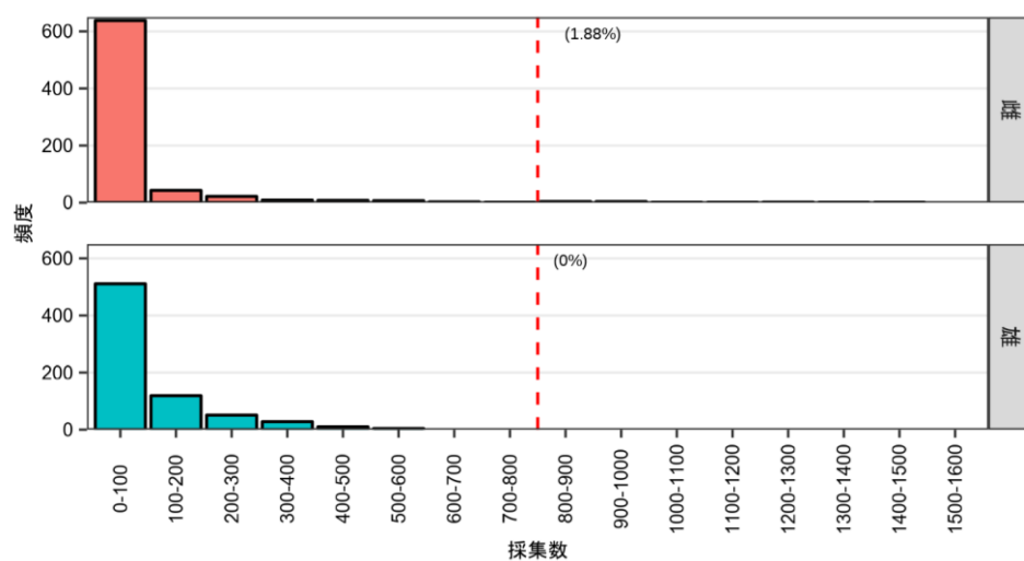
補足図 2-2. 定点別ズワイガニ採集個体数の頻度（1998～2025 年）
