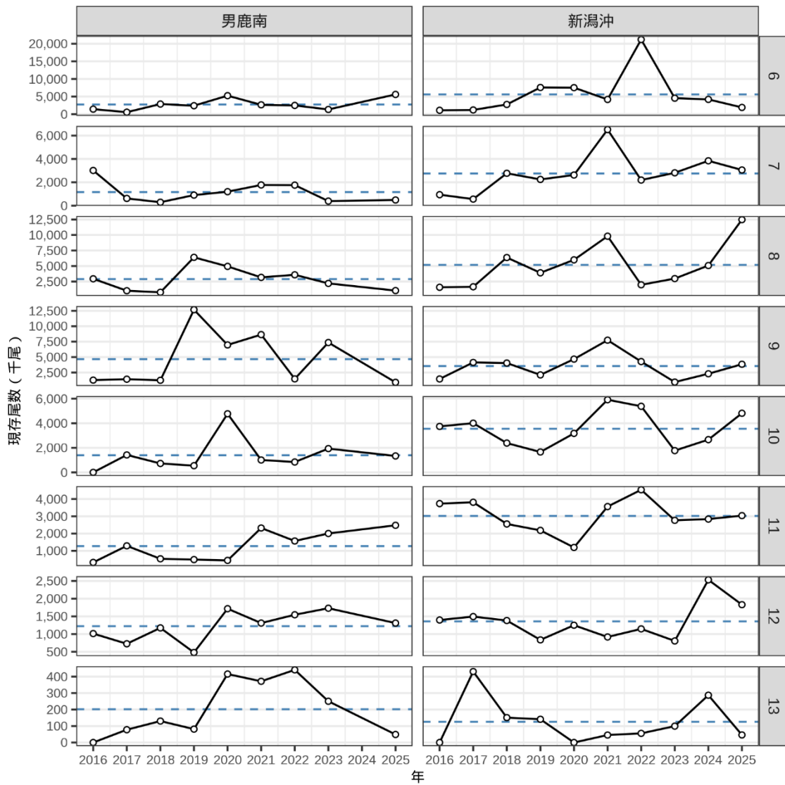
補足図 9-4. 桁網調査に基づく雄の齢期別現存尾数 (2016～2025 年)
