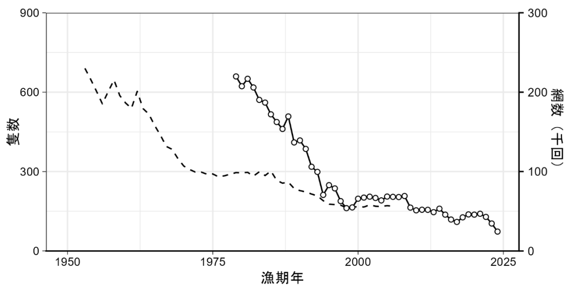
図 3-3. 沖底と小底の合計隻数（破線）および網数（白丸実線）
