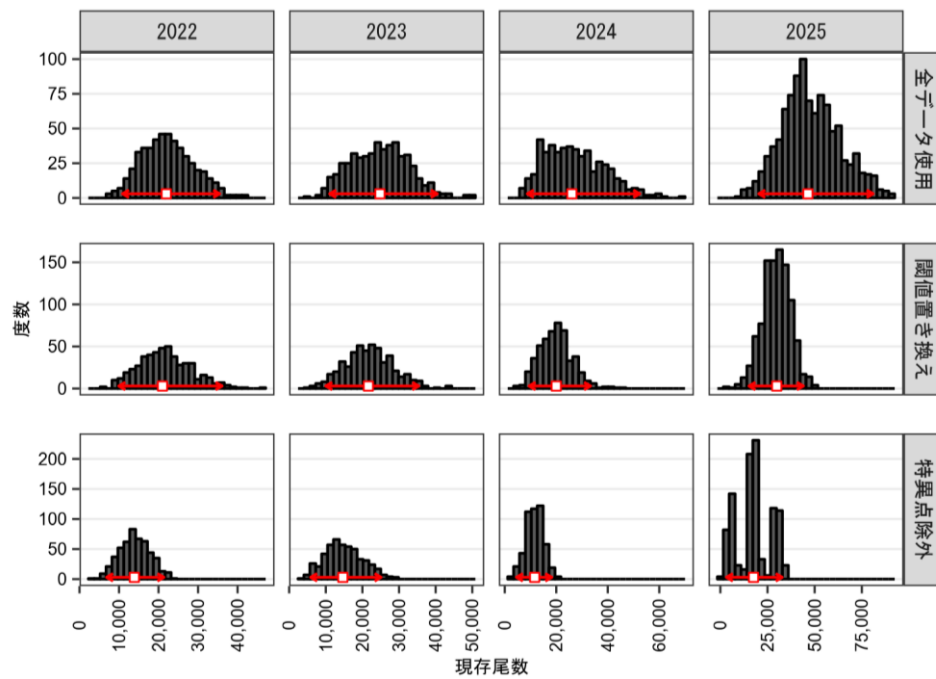
補足図 2-6. ブートストラップ法（500 回）に基づくズワイガニ雌の現存尾数推定値のヒストグラム、中央値（白四角）および 95%信頼区間（赤矢印）
