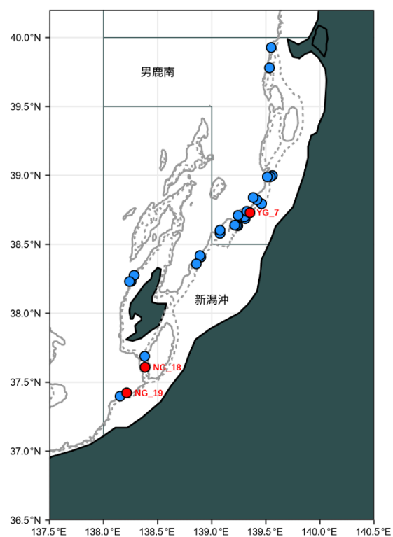
補足図 2-1. 2025 年かご調査の調査点
