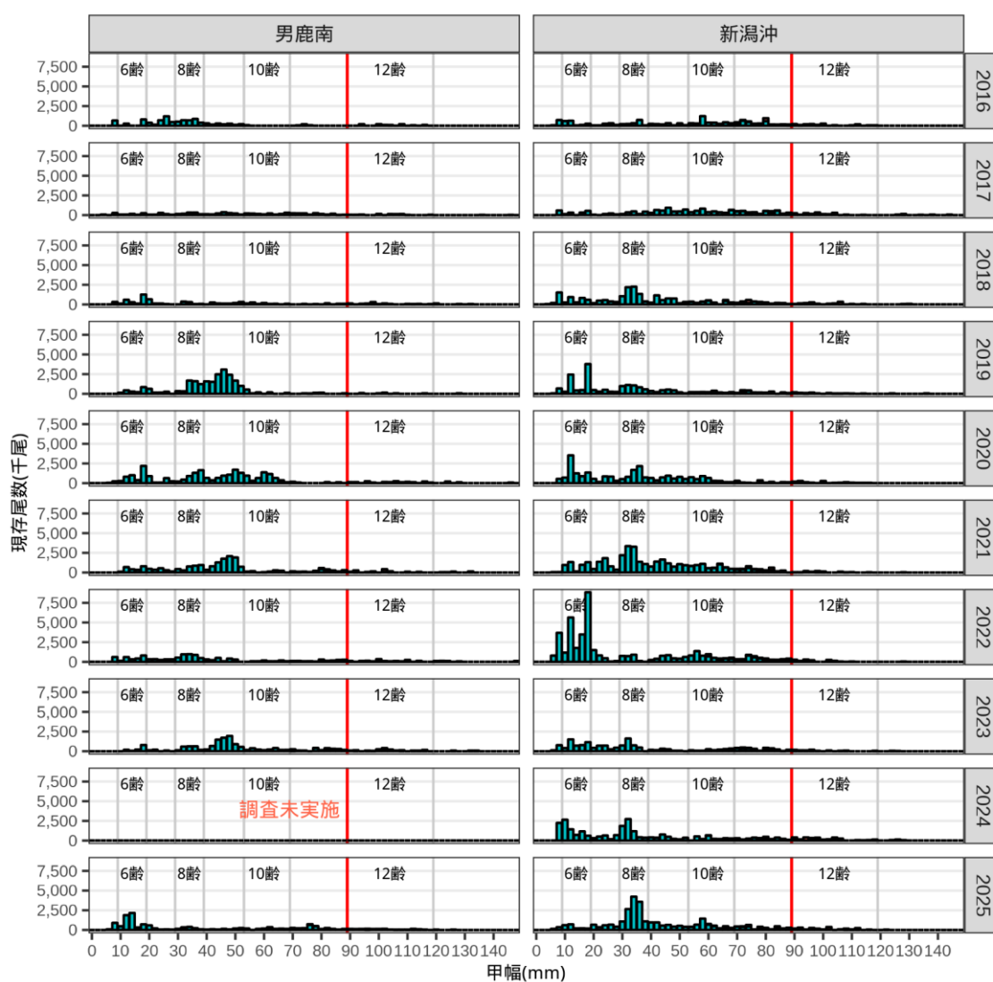
補足図 9-2. 桁網調査に基づく雄の甲幅組成 (2016～2025 年)
