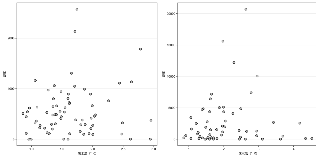
補足図 9-6. 採集密度上位 10 定点における出現密度と底水温の関係（雄：左、雌：右） 雄：甲幅 90 mm 以上、雌：11 齢に関する密度。当該上位 10 定点は補足図 9-7 を参照。
