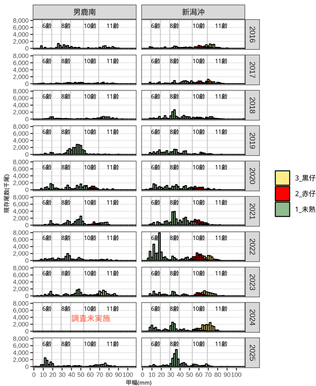
補足図 9-3. 桁網調査に基づく雌の甲幅組成 (2016~2025 年)
