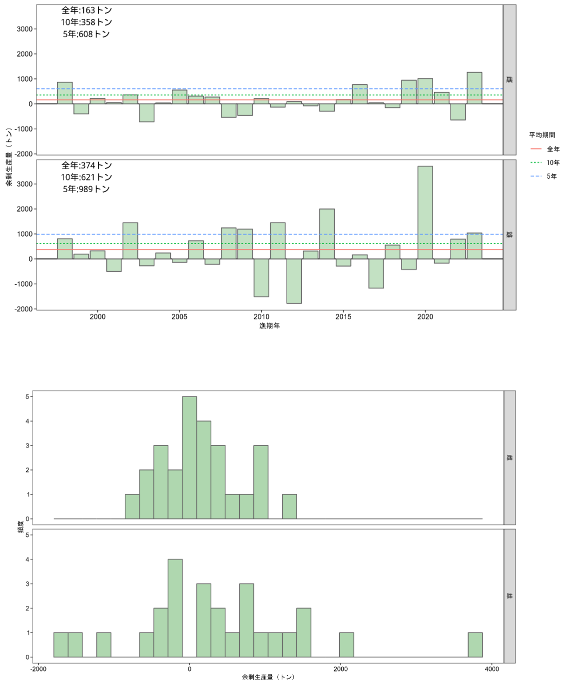
図 4-9 余剰生産量の時系列（上）と分布（下）
