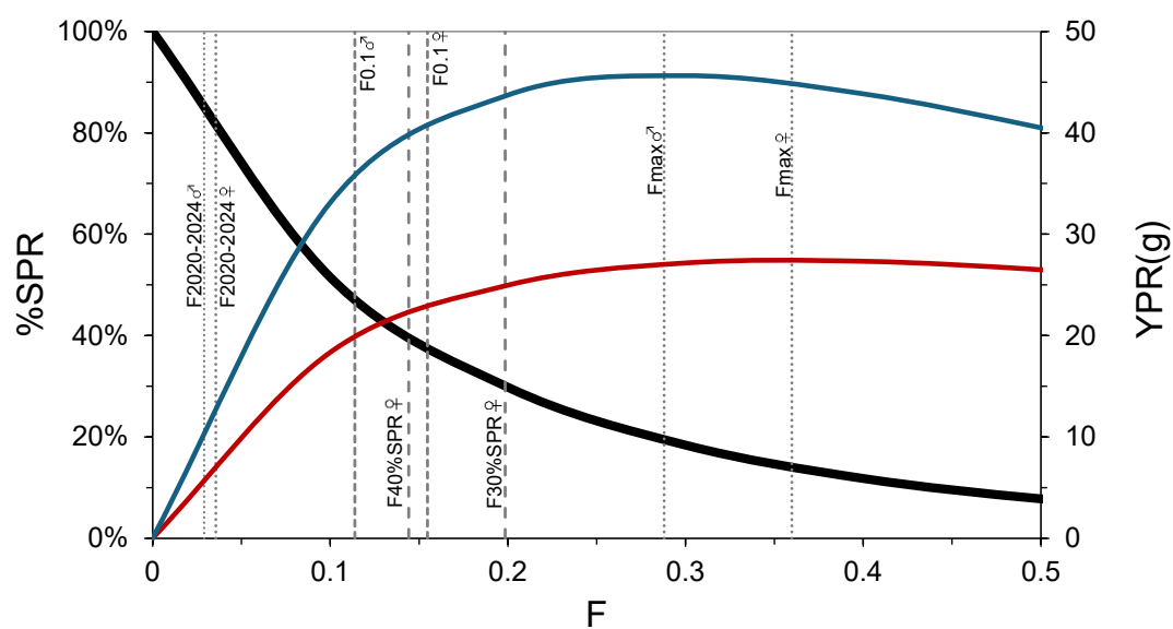
図 4-8. F と %SPR および YPR の関係
