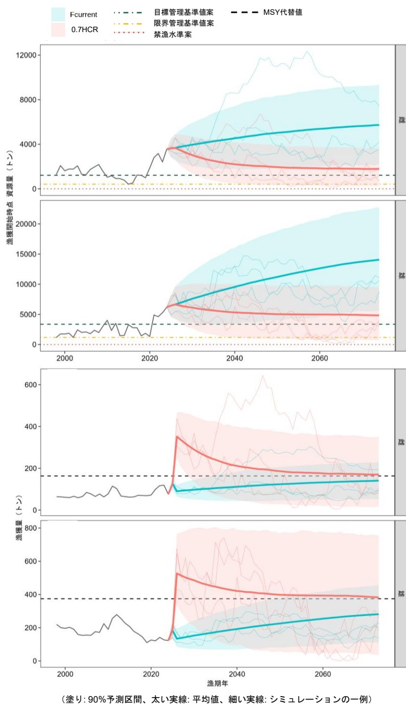
補足図 6-2. 管理基準値に基づく漁獲管理規則案を用いた将来予測（赤色）と現状の漁獲圧で漁獲を続けた場合の将来予測（青色）の比較
