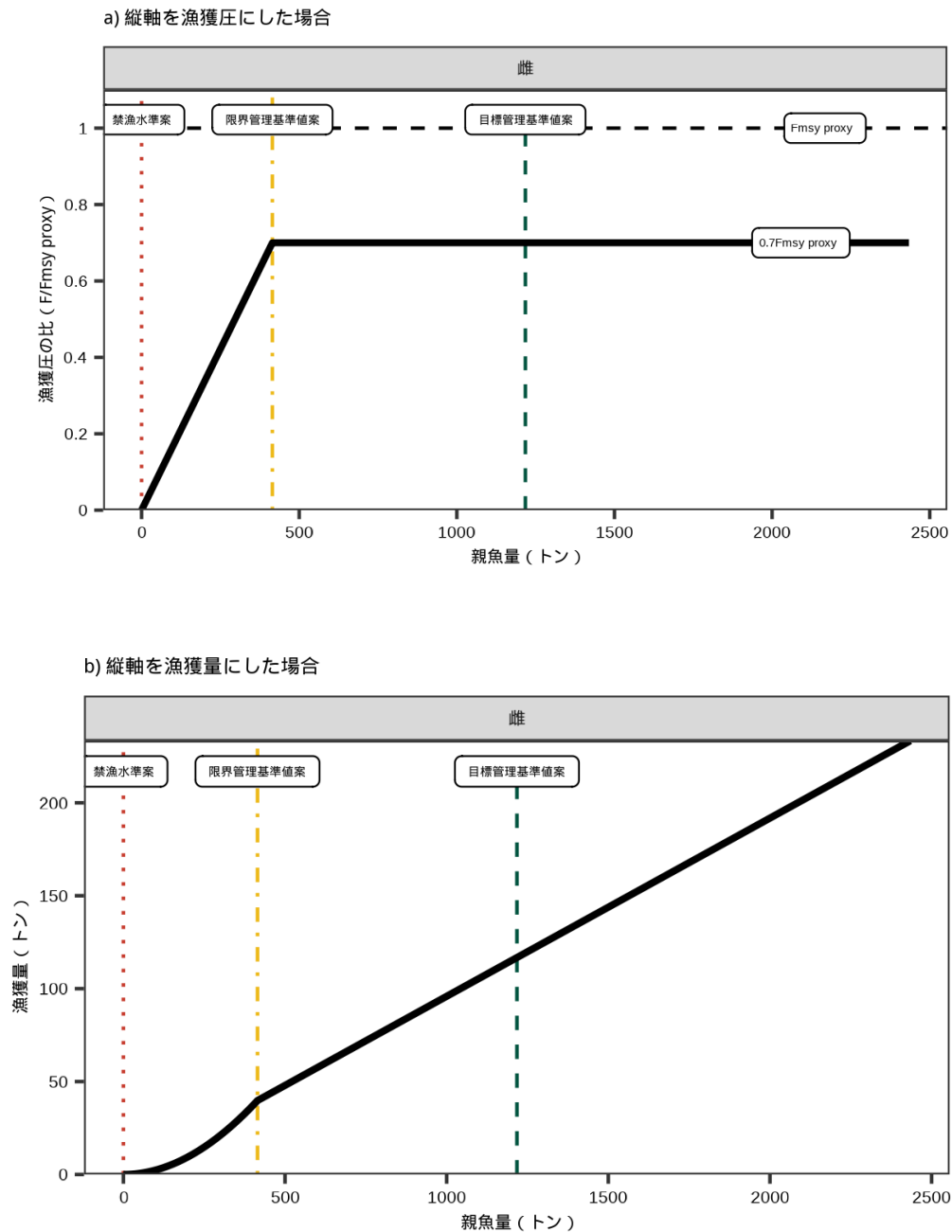
補足図 6-1. 漁獲管理規則案
