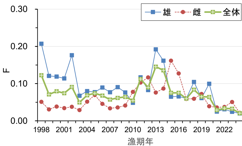
図 4-7. 漁獲係数 (F)
