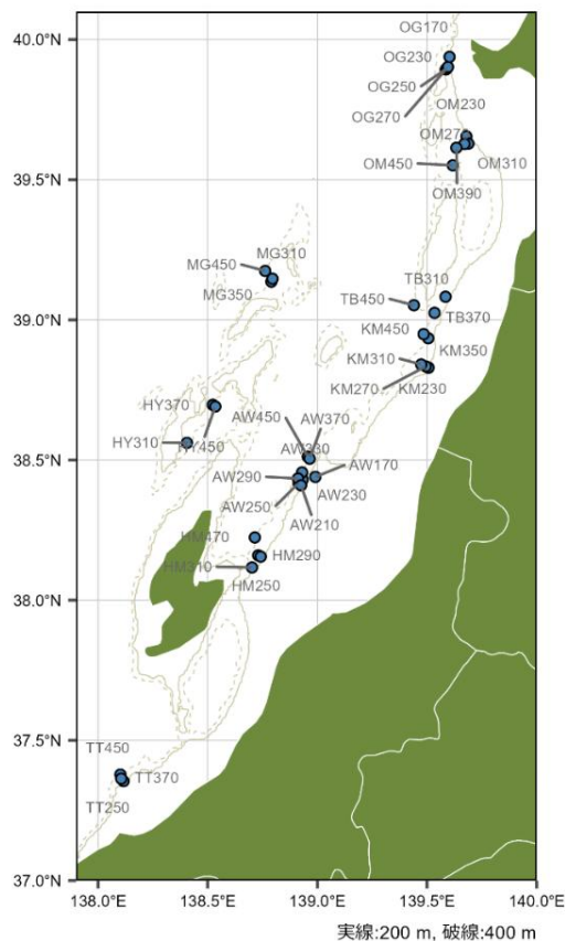
補足図 9-1. 桁網調査の調査海域図
