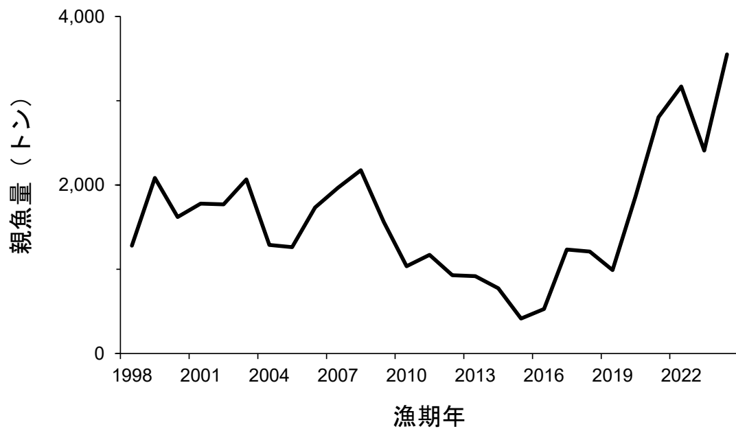
図 4-5. かご調査で推定した漁獲開始時点の親魚量 雌のアカコとクロコが含まれる。
