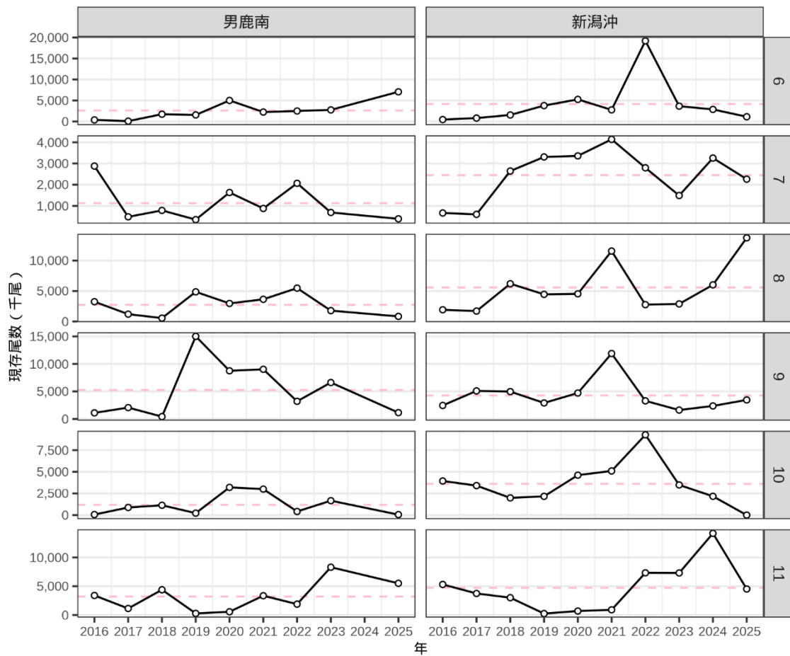
補足図 9-5. 桁網調査に基づく雌の齢期別現存尾数（2016～2025 年）
