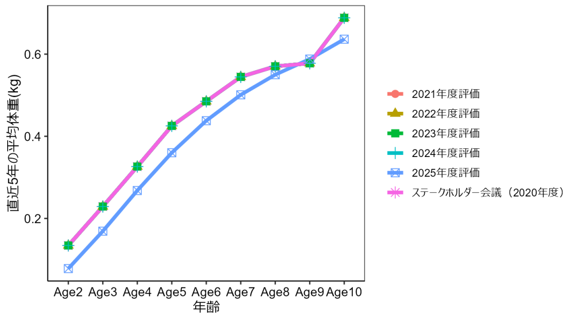
補足図 10-8. MSY 算定に用いた年齢別平均体重と、評価年度別の直近年の年齢別平均体重
