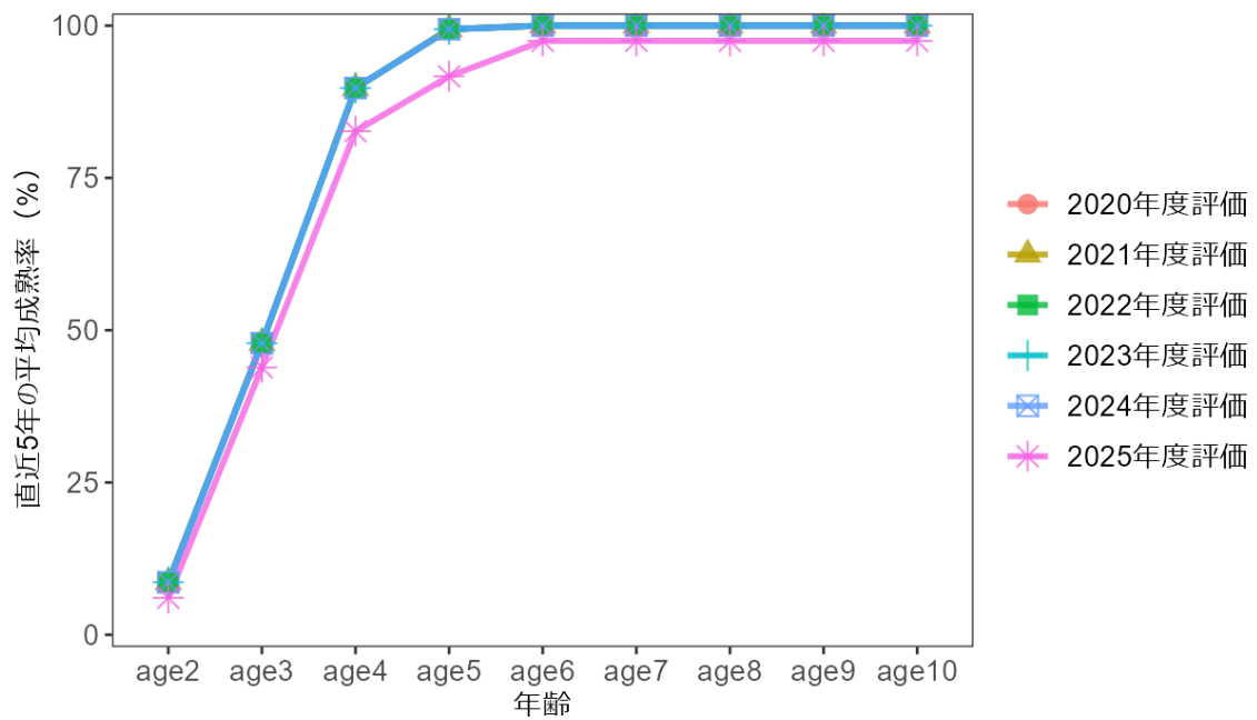
補足図 10-10. VPA における親魚量チューニングに用いた評価年度別の直近年の雌雄年齢別成熟率
