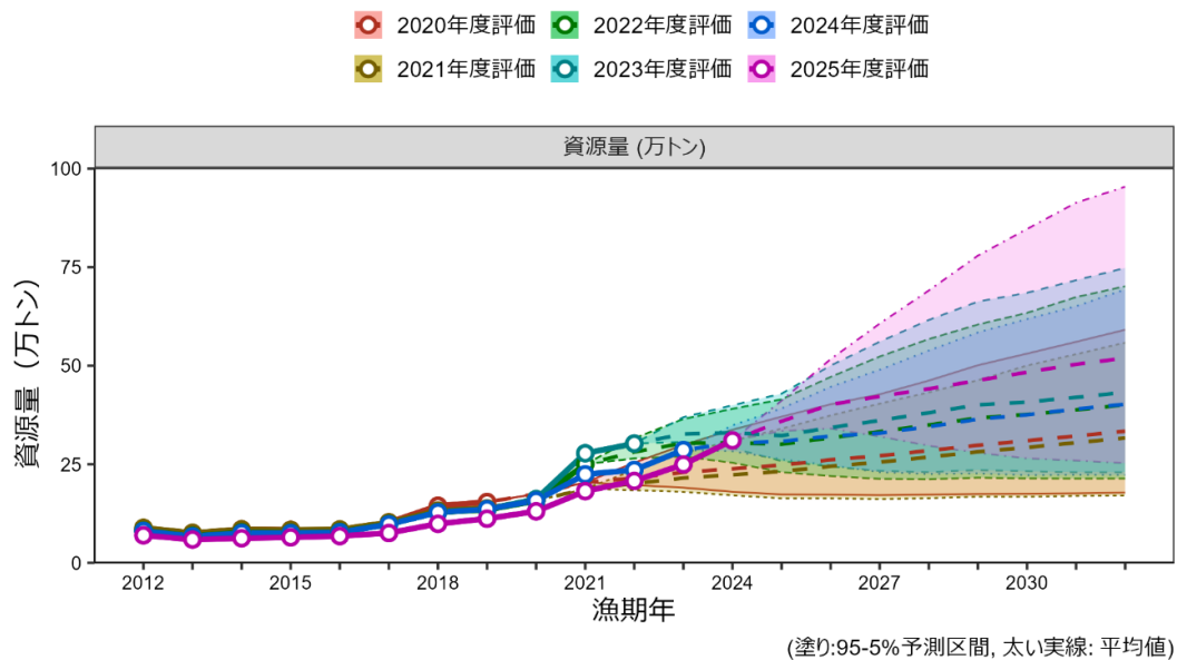
補足図 10-2. 評価年度別の資源量の比較
