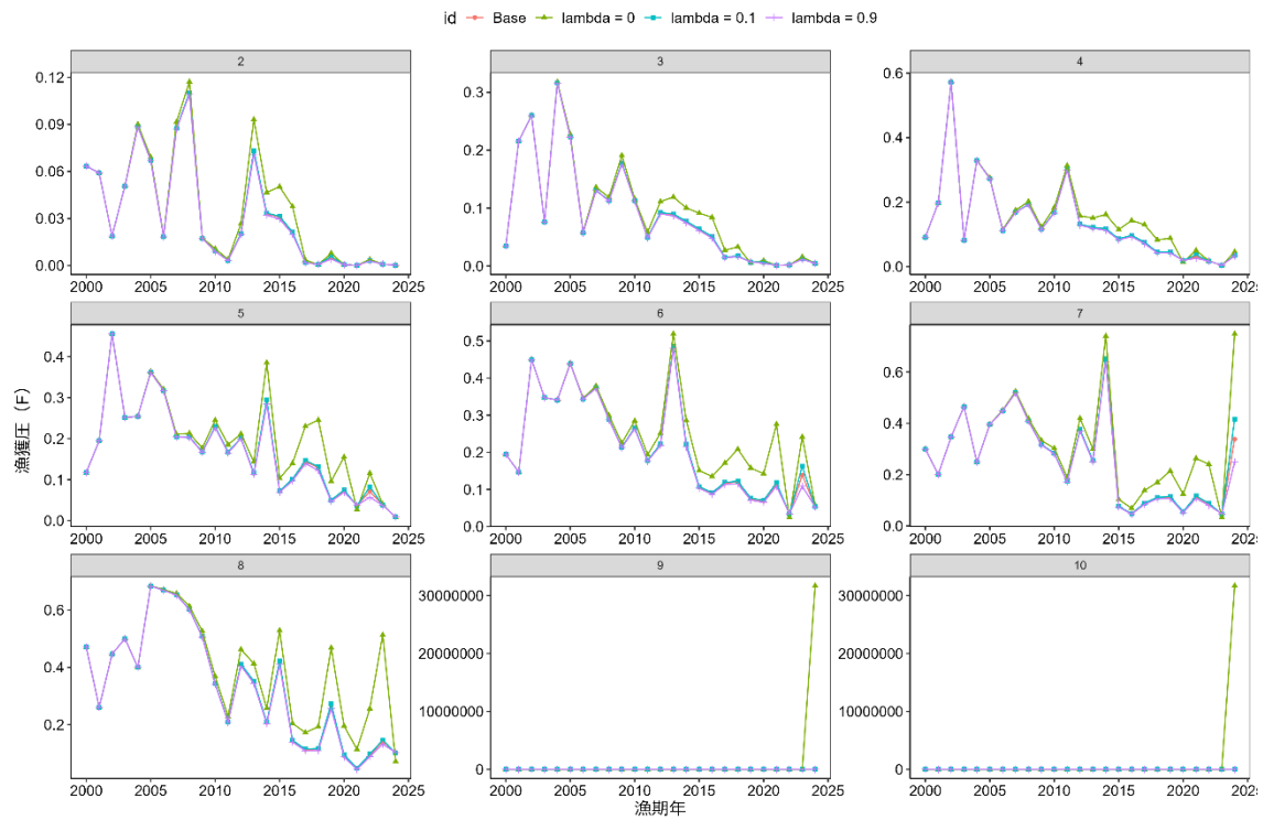
補足図 2-5. 年齢別 F に関する \lambda の感度分析結果
