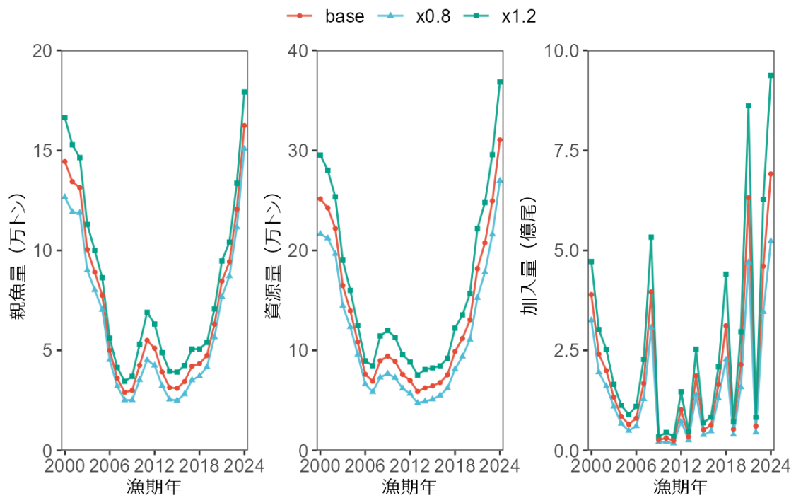
図 4-6. M の値を変化させた場合の感度分析の結果
