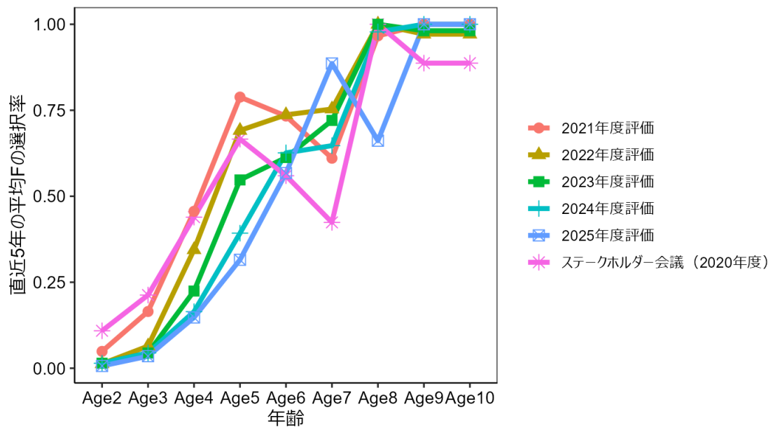
補足図 10-7. MSY 算定に用いた選択率と、評価年度別の直近年の選択率の比較
