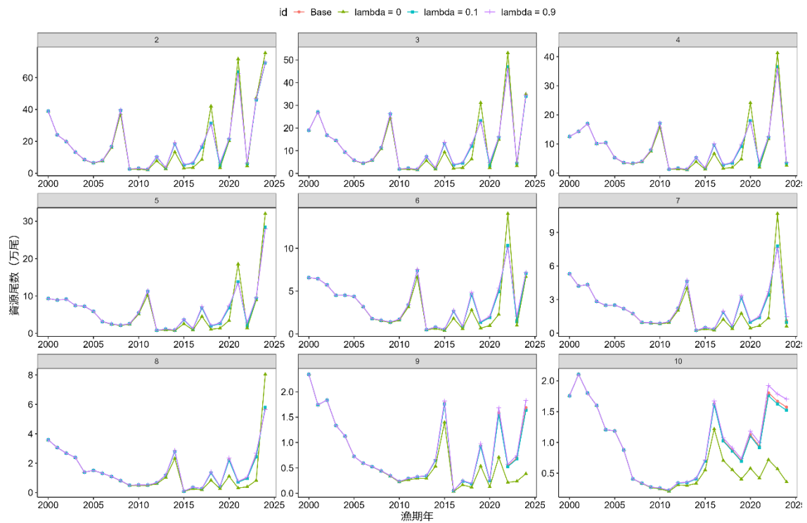
補足図 2-6. 年齢別資源尾数に関する \lambda の感度分析結果
