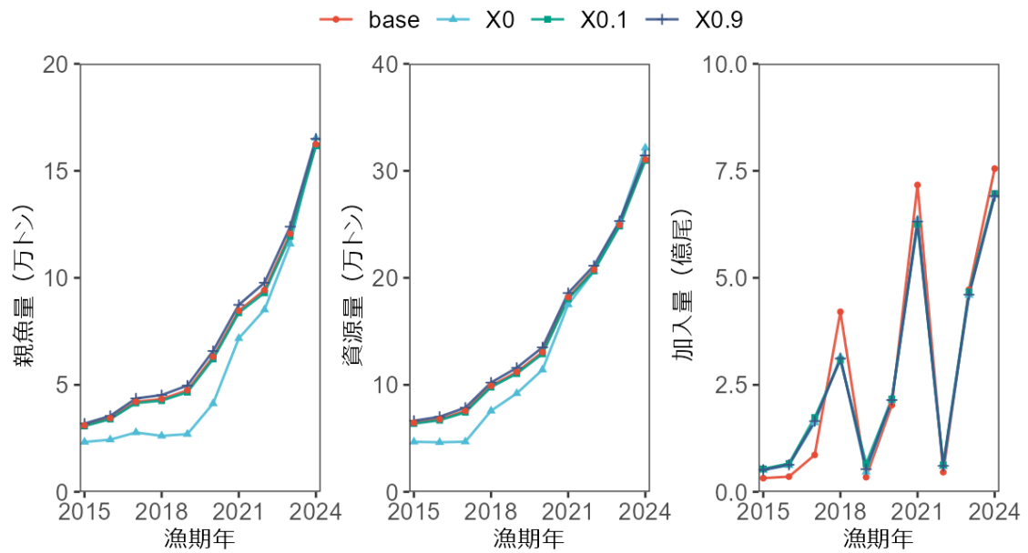
補足図 2-4. 親魚量 SSB、資源量 biomass、加入量 Recruitment に関する \lambda の感度分析結果
