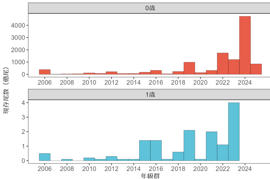
図 4-2. 加入量指標値の推移
