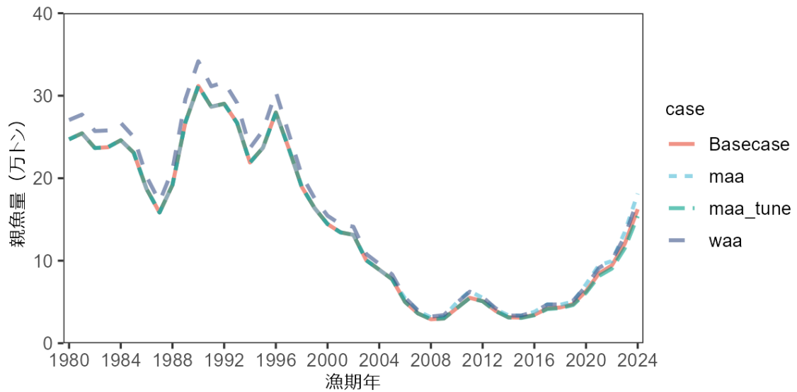
補足図 10-12. 2025 年度評価における生物パラメータの変更が親魚量推定値に及ぼす影響 Basecase は 2025 年度の資源評価モデルによる推定結果。maa、maa_tune、waa は 2025 年度の資源評価モデルから雌成熟率、雌雄成熟率、年齢別平均体重をそれぞれ従来の生物パラメータに戻して推定した結果。
