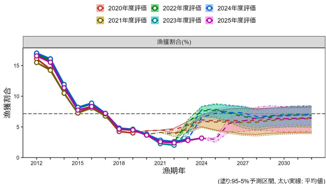
補足図 10-5. 評価年度別の漁獲割合（％）の比較
