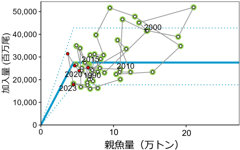
図6 再生産関係
