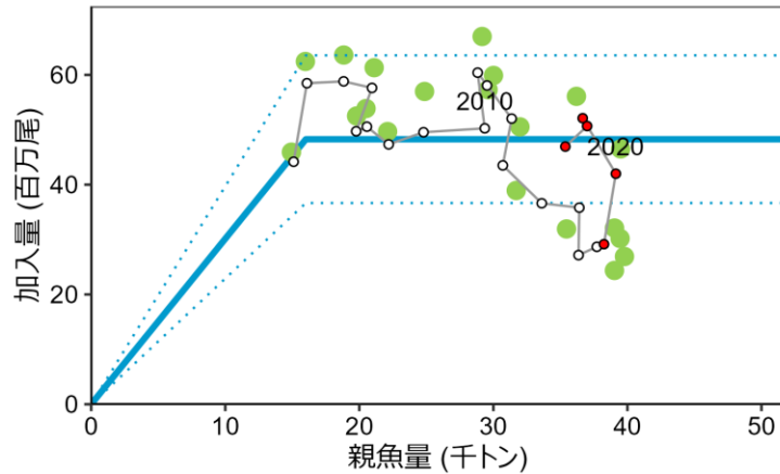
図6 再生産関係
