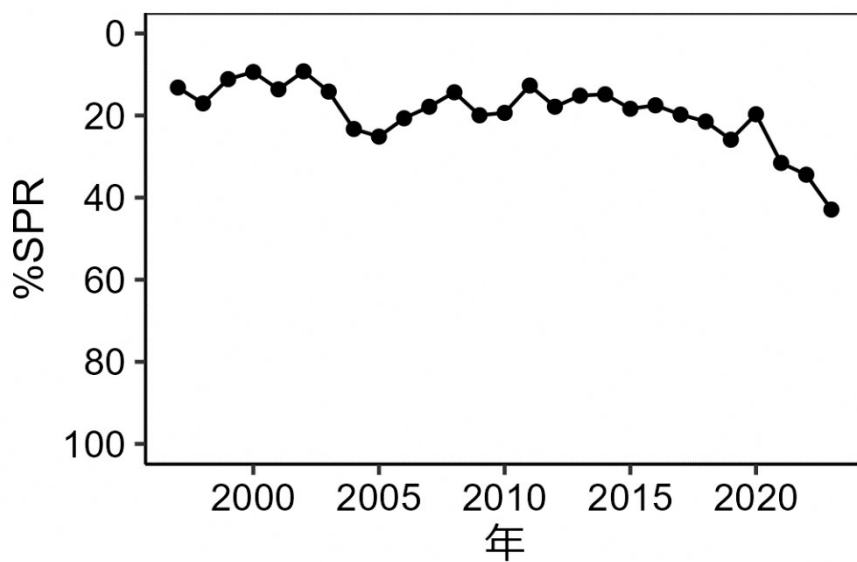
図 4-7. %SPR 値の推移
