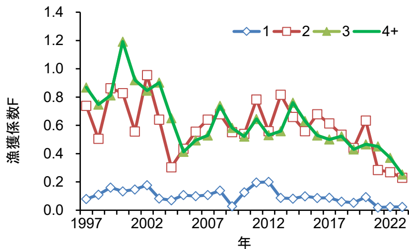
図 4-5. 年齢別漁獲係数 F の推移
