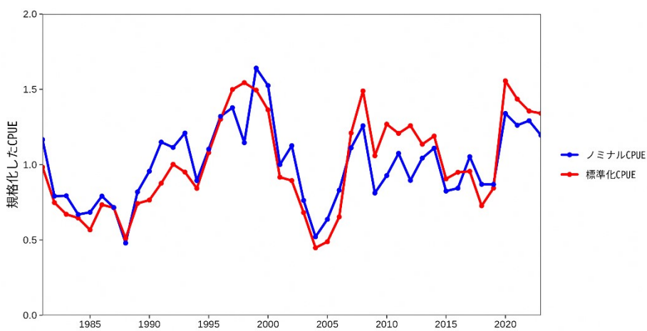
補足図 8-3. 平均で除して規格化したノミナル CPUE、標準化 CPUE
