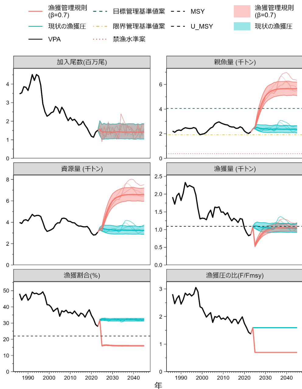
補足図 6-2. 将来の加入量として 2016~2020 年の加入に基づく加入のみを想定した場合の漁獲管理規則案を用いた場合（赤色）と現状の漁獲圧での将来予測（青色） 太実線は平均値、網掛けはシミュレーション結果の90%が含まれる90%予測区間、細線は3通りの将来予測の例示である。親魚量の図の緑破線は目標管理基準値案、黄一点鎖線は限界管理基準値案、赤点線は禁漁水準案を示す。漁獲割合の図の破線はUmsy proxyを示し、漁獲量の図の破線はMSY proxyを示す。2024年の漁獲は予測される資源量と現状の漁獲圧（F2020-2022）により仮定し、2025年以降の漁獲は漁獲管理規則案（補足図 6-1）に従うものとした。調整係数 \beta には 0.7 を用いた。
