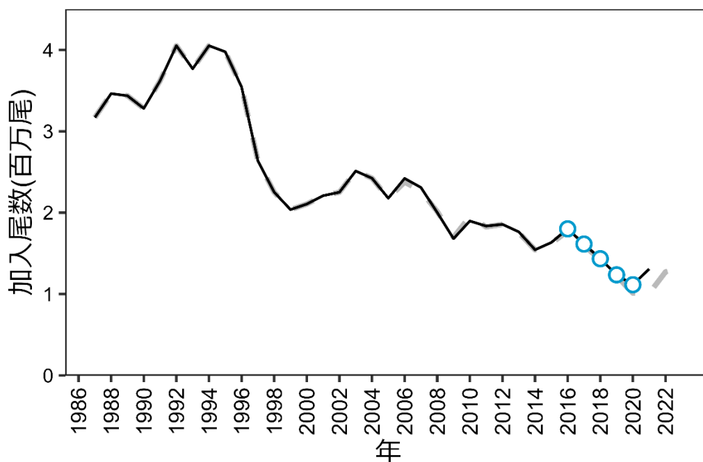
図 4-9. 加入量の推移と将来予測に用いた加入の仮定 令和 4 (2022) 年度ヒラメ日本海中西部・東シナ海系群の資源評価 (増渕ほか 2023) における天然由来加入尾数を用いて将来の加入を仮定する (実線)。青枠白塗りつぶ
