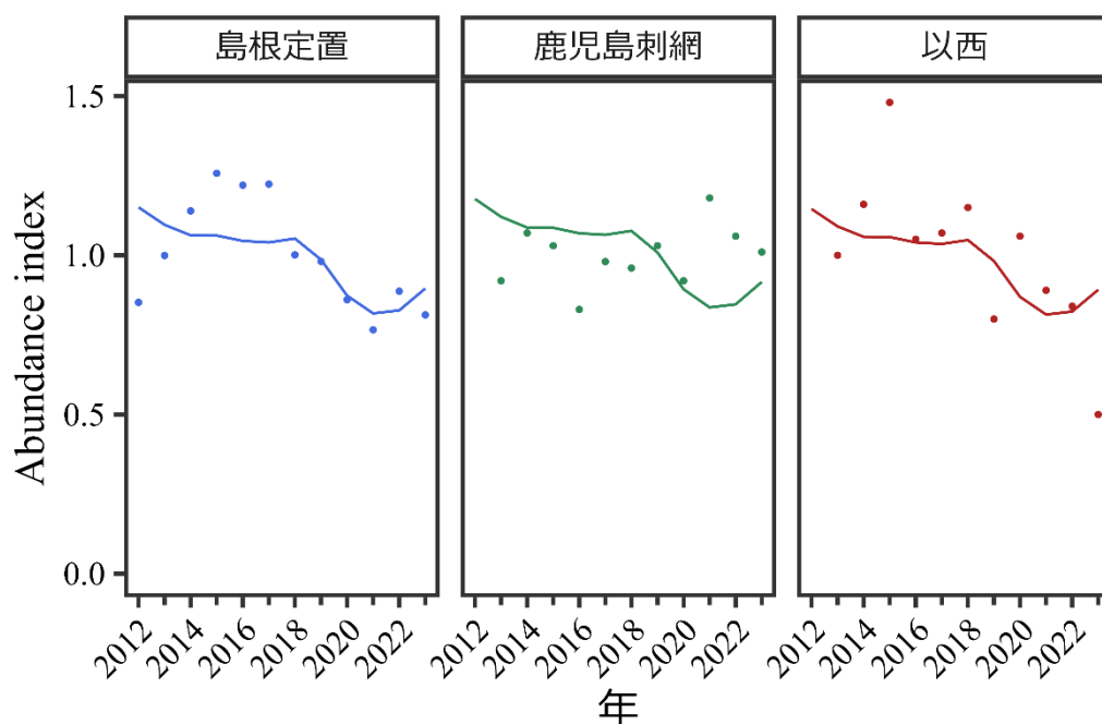
補足図 2-3. 指標値の観測値（丸印）とモデルの予測値（実線）の時系列プロット
