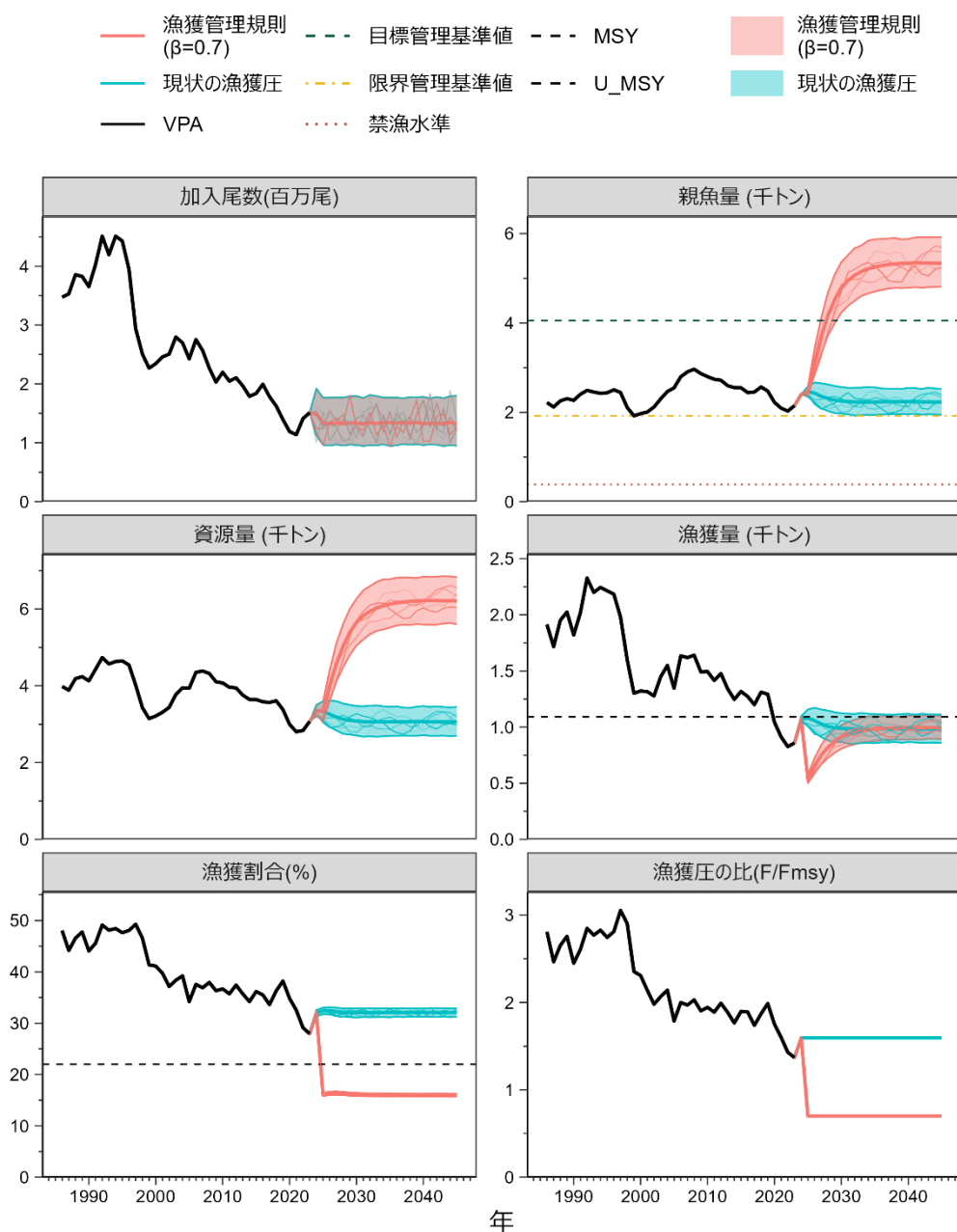
補足図 9-1. 将来の加入量として、今年度評価で更新された 2018～2022 年の天然由来の加入水準に基づく加入のみを想定した場合の漁獲管理規則案を用いた場合（赤色）と現状の漁獲圧での将来予測（青色）
