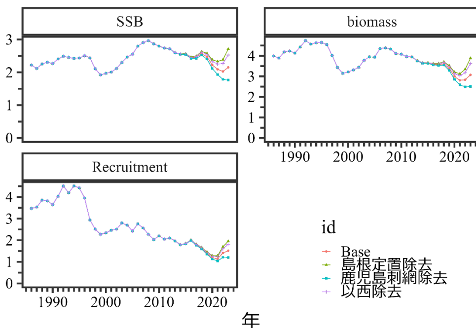
補足図 2-6. ジャックナイフ解析の結果 親魚量 (SSB)、資源量 (biomass) の単位は千トン、加入尾数 (Recruitment) の単位は百万尾。
