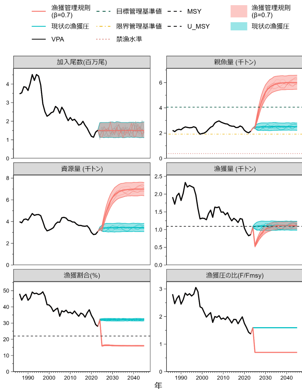
補足図 9-2. 加入参照年を 2018~2022 とし現状の放流を想定した場合の漁獲管理規則
