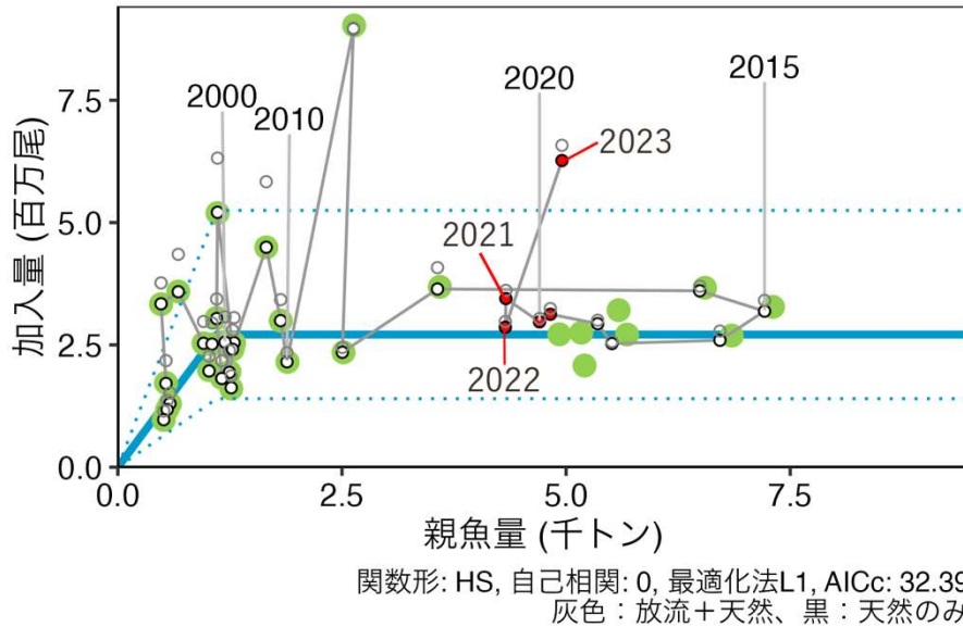
図 4-11. 親魚量と加入量の関係 青実線は本系群で適用した再生産関係式であり、上下の点線は、仮定されている再生産関係において観察データの 90%が含まれると推定される範囲である。再生産関係式のパラメータ（自己相関を考慮しないホッケー・スティック（HS）型再生産関係式を用い、最小絶対値法により推定）は令和 4 年 9 月に開催された「管理基準値等に関する研究機関会議」（富樫ほか 2022a）に示された値に基づく。塗りつぶしの黄緑丸印は、この再生産関係推定時の親魚量と加入量を示す。白抜丸印および赤丸印は本年度評価における 1990～2022 年の親魚量と 1991～2023 年の加入量を示し、黒色は天然のみ、灰色は種苗放流を加味した値である。図中の数字は加入群（1 歳魚）の加入年を示す。
