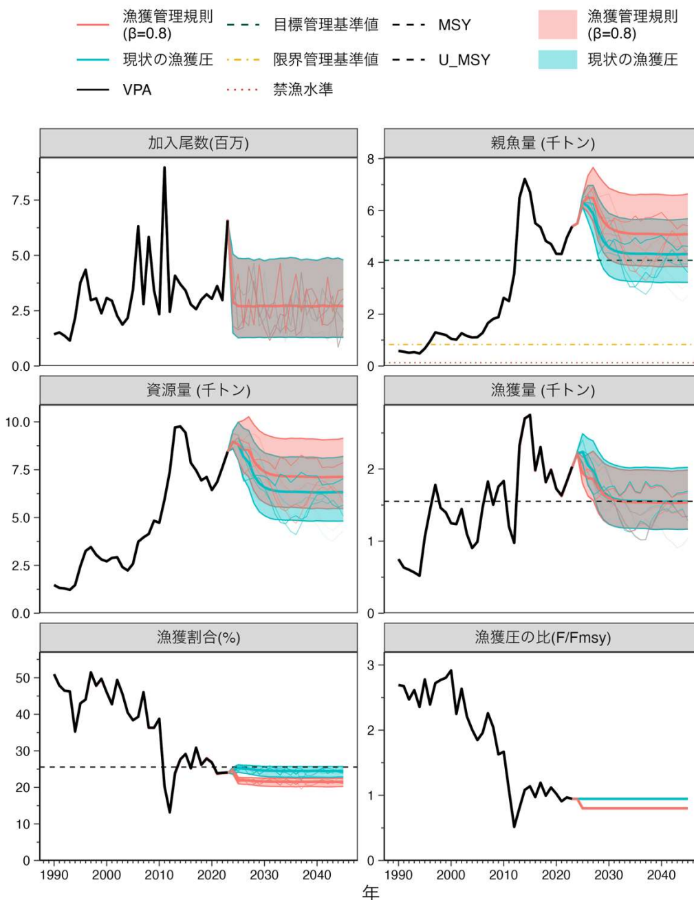
補足図 5-2. 再生産関係による加入のみを考慮した場合における漁獲管理規則案を用いた場合（赤色）と現状の漁獲圧（F2020-2022）での将来予測（青色） 太実線は平均値、網掛けはシミュレーション結果の90%が含まれる90%予測区間、細線は5通りの将来予測の例示である。親魚量の図の緑破線は目標管理基準値案、黄点線は限界管理基準値案、赤線は禁漁水準案を示す。漁獲量の図の破線はMSY、漁獲割合の図の破線はUmsyを示す。2024年の漁獲は予測される資源量と現状の漁獲圧(F2020-2022)により仮定し、2025年以降の漁獲は漁獲管理規則案（補足図 5-1）に従うものとした。調整係数 \beta には0.8を用いた。
