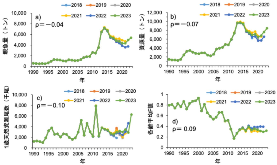
補足図 2-1. a) 親魚量、b) 資源量、c) 1歳天然資源尾数、d) 各齢平均 F 値のレトロスペクティブ解析結果 凡例の数字はコホート解析の最終年を示す。
