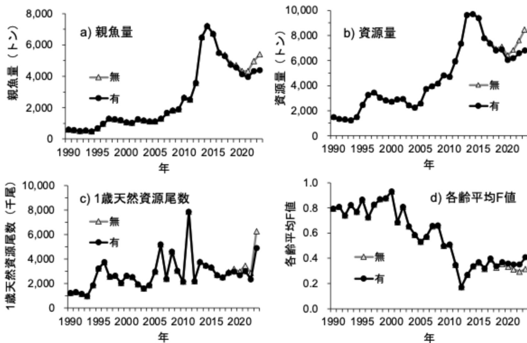
補足図 3-1. チューニング有無による a) 親魚量、b) 資源量、c) 1 歳天然資源尾数、d) 各 齢平均 F 値の比較
