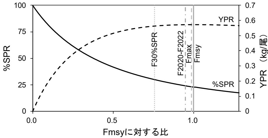
図 4-10. Fmsy に対する YPR と%SPR の関係
