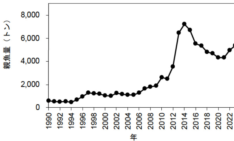
図 4-4. 親魚量の推移 雌雄込で 2 歳魚の 1/4、3 歳魚の 3/4、4 歳以上魚の資源量の合計値とした。
