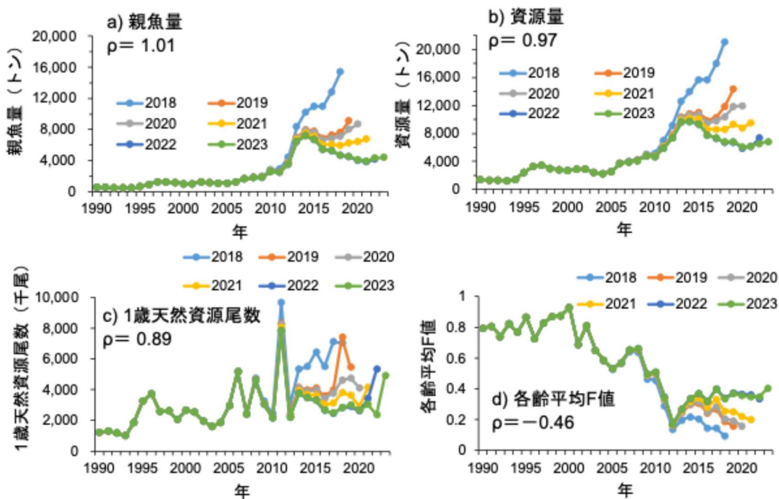
補足図 3-2. チューニングした場合の a) 親魚量、b) 資源量、c) 1 歳天然資源尾数、d) 各 齢平均 F 値のレトロスペクティブ解析結果
