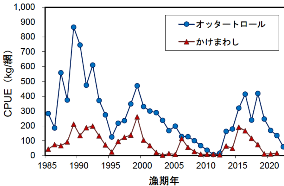
図 3-4. オホーツク海日本水域における沖底の CPUE の推移
