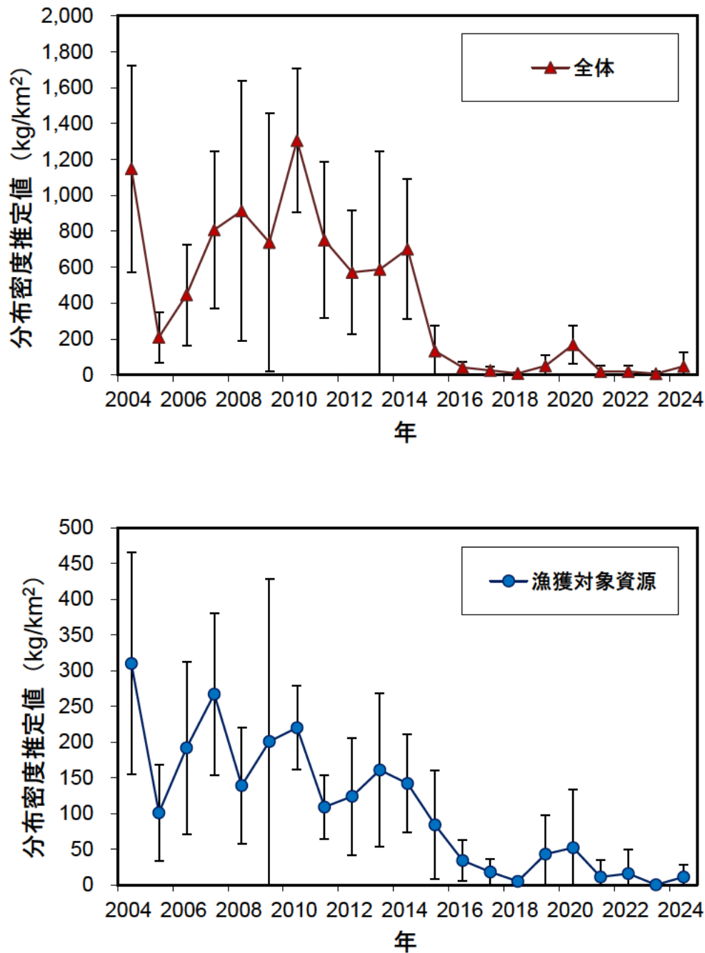
図 4-1. 2004～2024 年のオホーツク海におけるズワイガニの分布密度推定値の推移 縦棒は 95%信頼区間、ただし 2014 年の信頼区間は海氷の影響で十分な曳網数が確保できなかった水域を除いて算出した。
