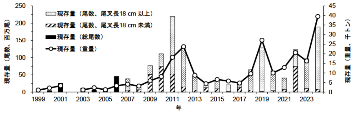
図 4-4. オホーツク海底魚資源調査により推定されたスケトウダラの現存量 2002 年は調査未実施のためデータ無し。
