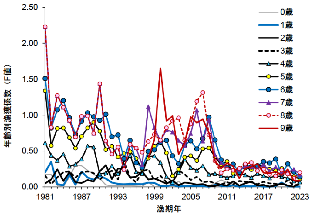
図 4-9. 各年齢の漁獲係数 (F 値) の推移 10 歳以上の F 値は 9 歳と同じである。
