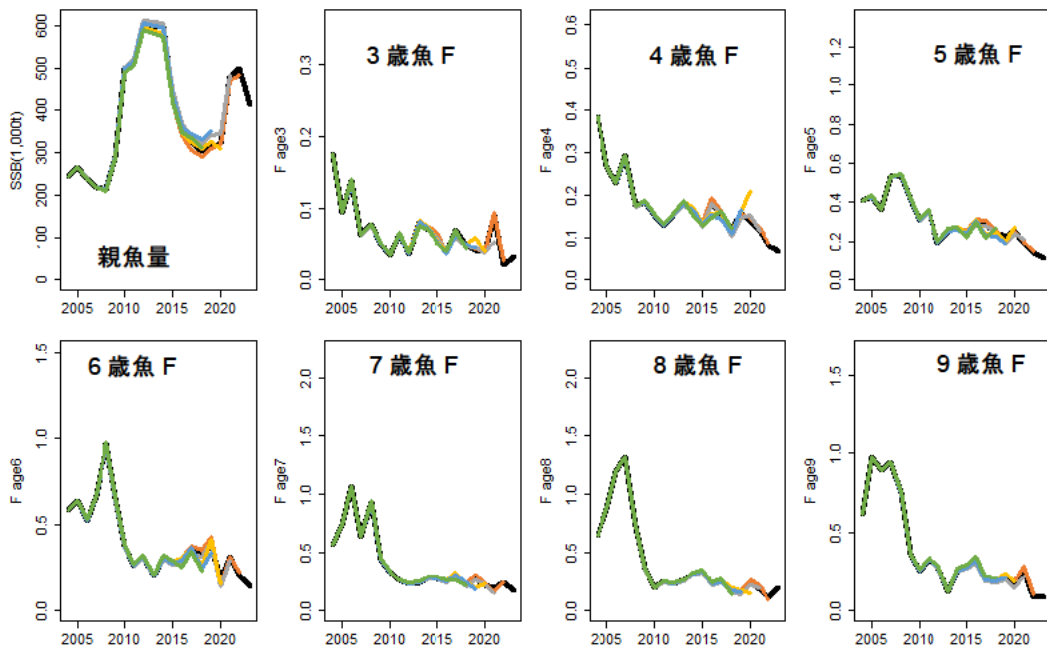
補足図 6-2. 評価で採用したリッジ VPA のペナルティのレトロスペクティブ解析結果 ペナルティ \lambda を 0.785、 \eta を 0.955 とした場合の結果を示す。
