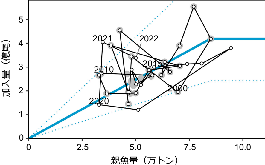
図6 再生産関係
