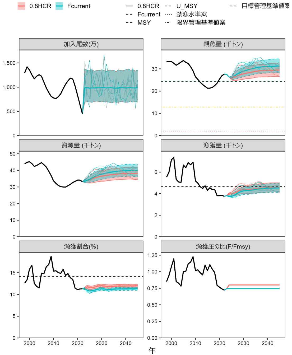
補足図 4-2. 漁獲管理規則案を用いた場合 (赤線) と現状の漁獲圧での将来予測 (青色) 太実線は平均値、網掛けはシミュレーション結果の 90%が含まれる予測区間、細線は 5 通りの将来予測の例示である。親魚量の図の緑破線は目標管理基準値案、黄鎖線は限界管理基準値案、赤点線は禁漁水準案を示す。漁獲割合の図の破線は最大持続生産量 MSY を達成する漁獲割合 (Umsy) を示す。漁獲管理規則案での調整係数 \beta には 0.8 を用いた。
