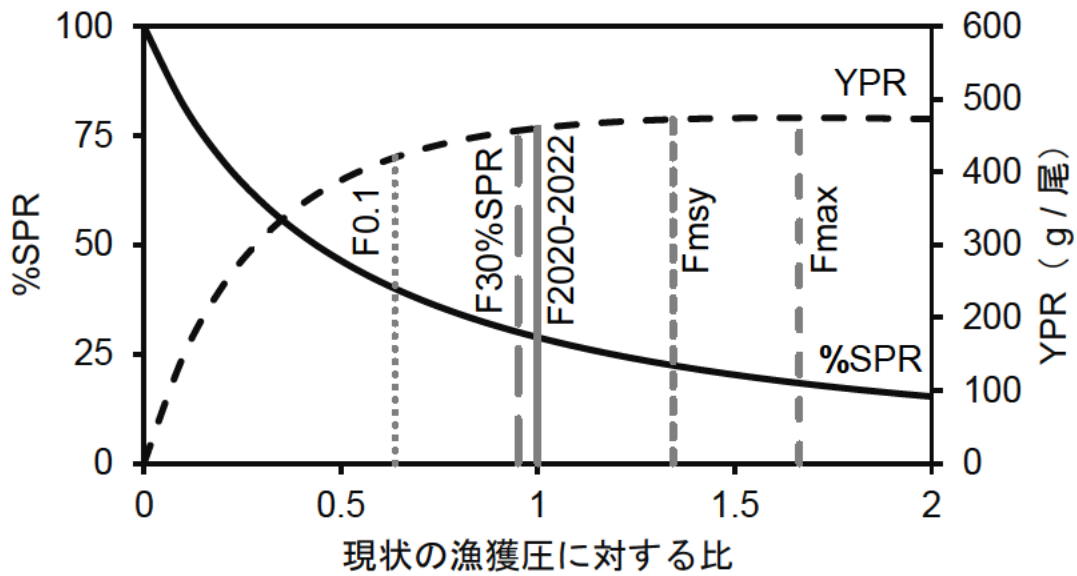
図 4-9. 現状の漁獲圧 (F2020-2022) に対する YPR と%SPR の関係
