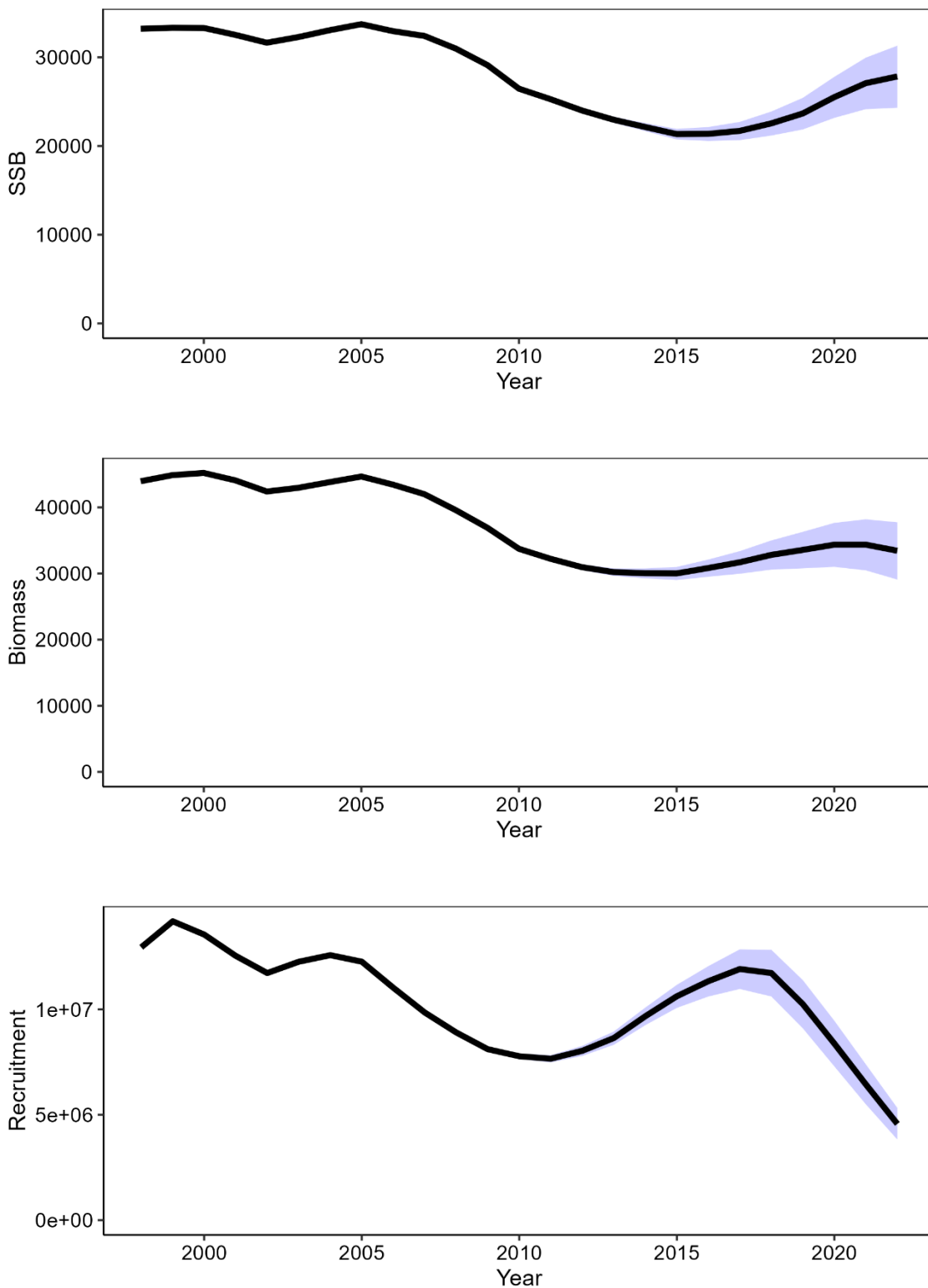
補足図 2-5. 親魚量 (SSB)、資源量 (Biomass)、加入量 (Recruitment) のブートストラップ解析、推定値 (黒実線) と 95%信頼区間 (青色) を表す。
