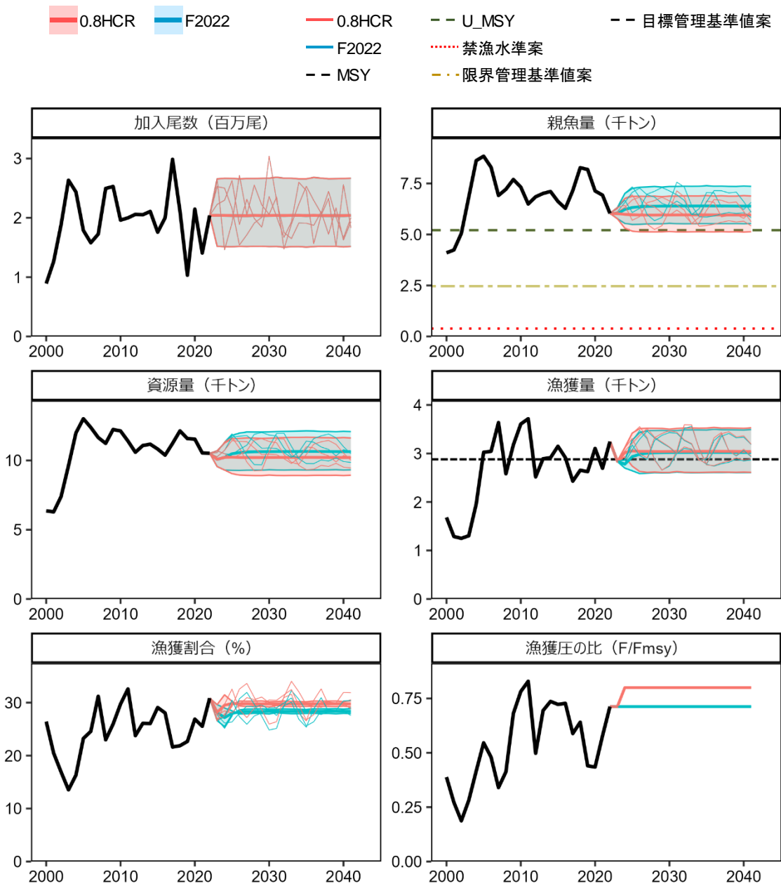
補足図 4-2. 漁獲管理規則案および現状の漁獲圧による将来予測の比較
