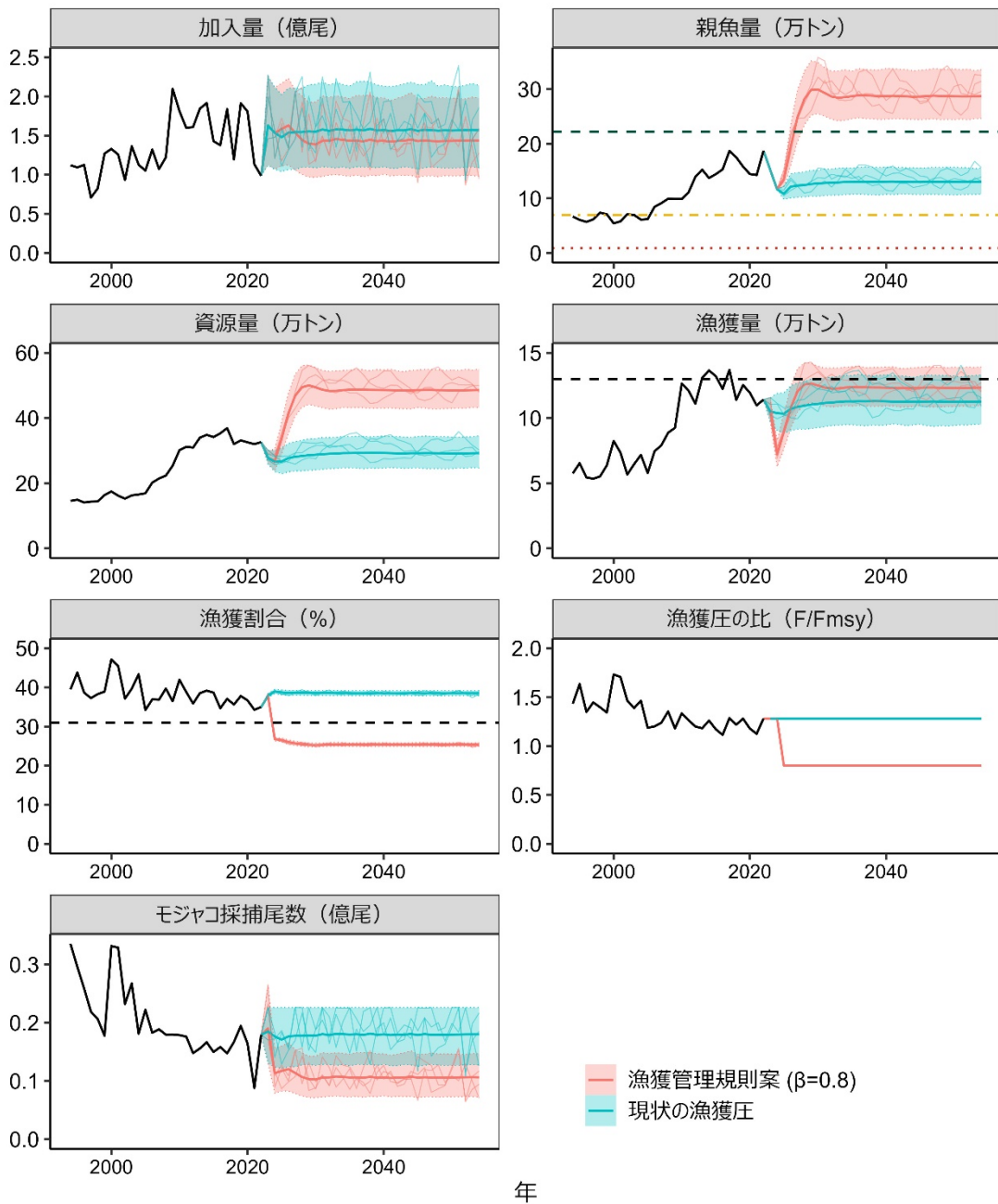
補足図 4-2. 漁獲管理規則案を用いた場合（赤線）と現状の漁獲圧での将来予測（青色） 太実線は平均値、網掛けはシミュレーション結果の90%が含まれる90%予測区間、細線は3通りの将来予測の例示である。親魚量の図の緑破線は目標管理基準値案、黄一点鎖線は限界管理基準値案、赤点線は禁漁水準案を示す。漁獲割合の図の破線は U_{msy} を示す。2023年の漁獲量は予測される資源量と現状の漁獲圧（ F_{2023} ）により仮定し、2024年以降の漁獲は漁獲管理規則案（補足図 4-1）に従うものとした。現状の漁獲圧でのモジャコ採捕尾数の将来予測では、最近10年間の採捕計画尾数の平均値をモジャコ採捕尾数の上限とした。調整係数 \beta には 0.8 を用いた。
