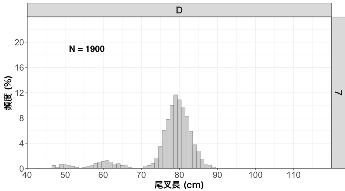
図 7b 大型竿釣り船の月別・海区別のビンナガ体長組成 (図上のアルファベットは海区, 図右の数字は漁獲月を示す).
