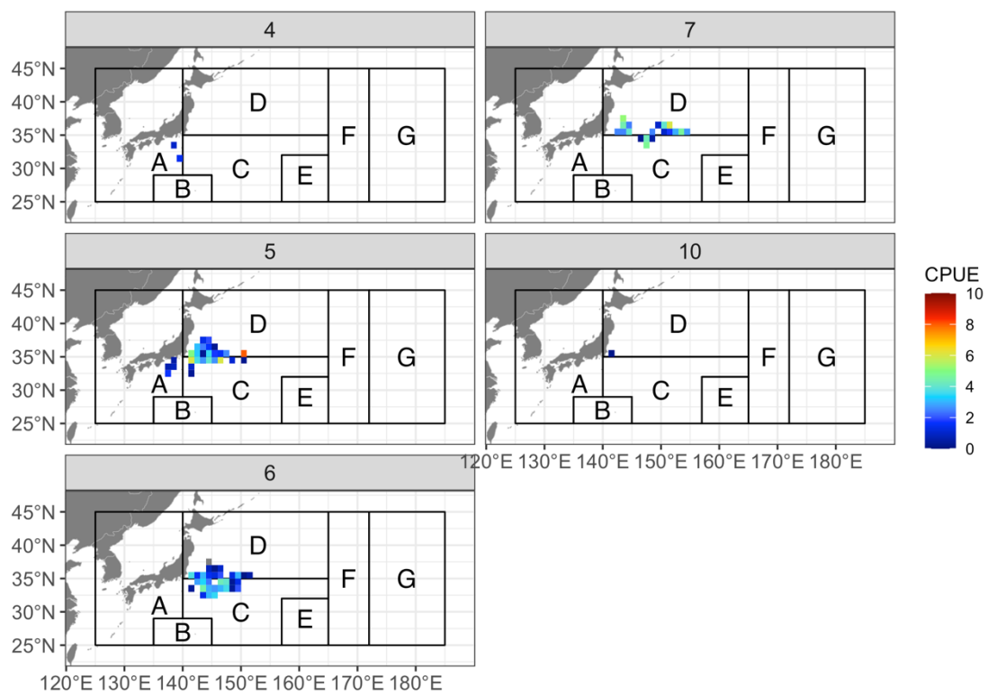
図3 中型竿釣り船の月別ピンナガ CPUE(トン/日・隻)の分布. 図の上の数字は漁獲月を示す.
