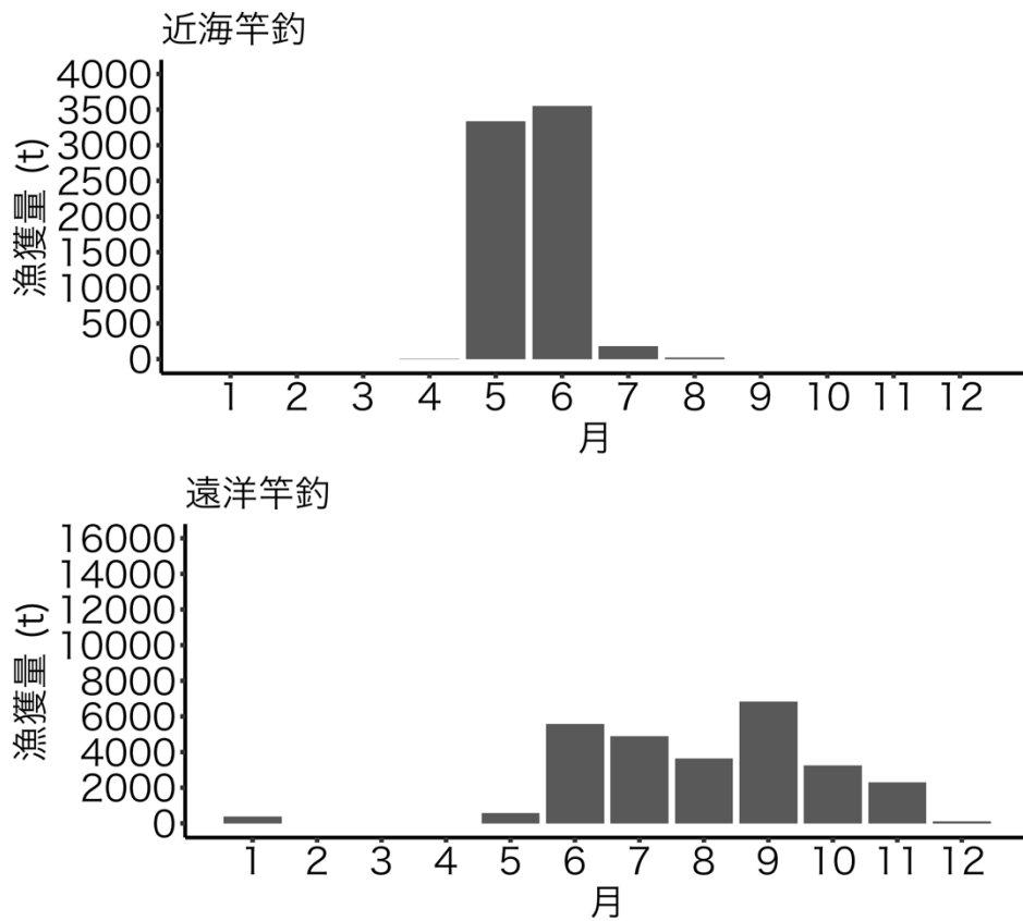
図 2 月別・漁法別(中型竿釣り船(上), 大型竿釣り船(下))のビンナガの水揚げ量の推移.
