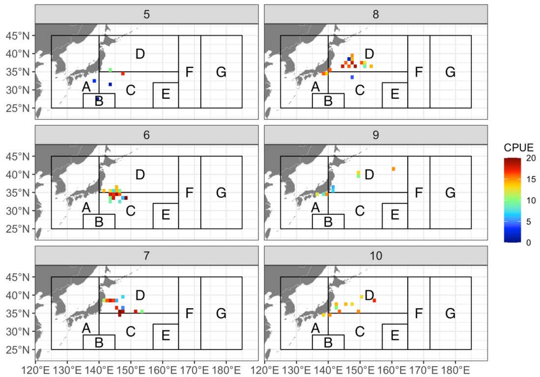
図 5 大型竿釣り船の月別ビンナガ CPUE(トン/日・隻)の分布. 図の上の数字は漁獲月を示す. 1-4,11,12 月は当該海域内での漁獲は無かった.
