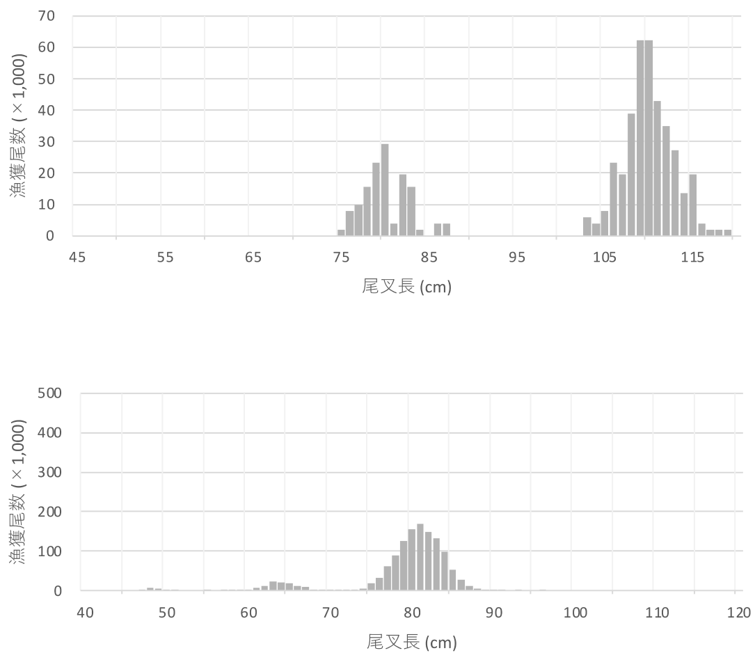
図 8 中型竿釣り船（上）および大型竿釣り船（下）によって漁獲されたビンナガの体長別漁獲個体数.
