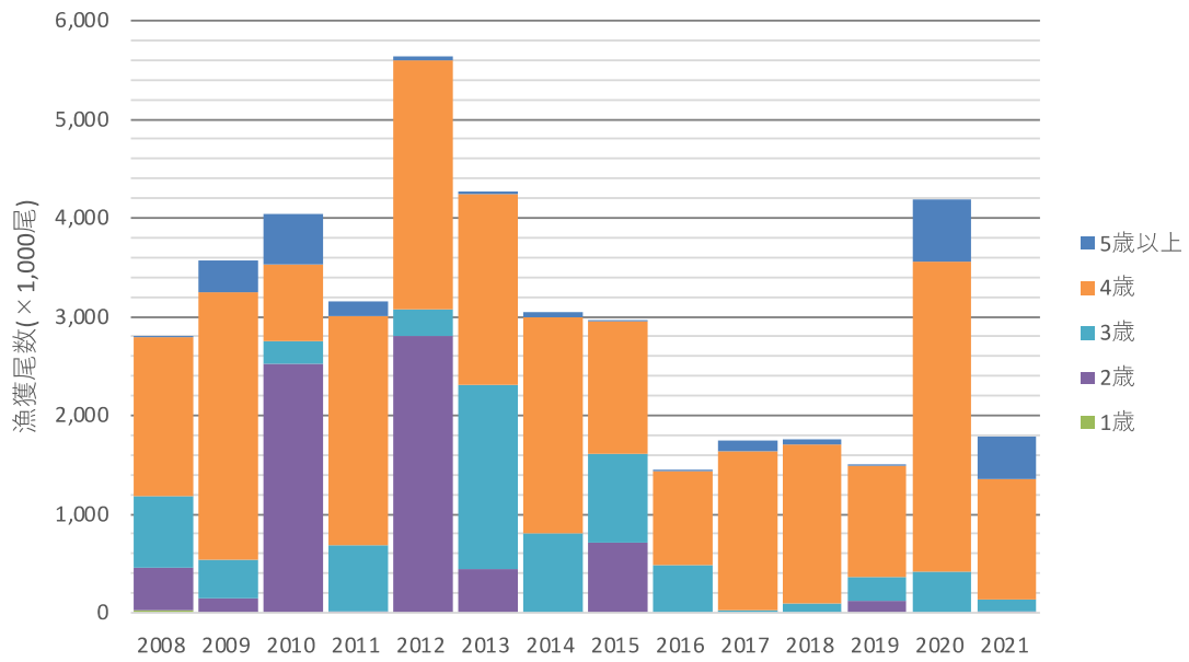
図 9 竿釣りによるビンナガの年齢別漁獲個体数の経年変化.
