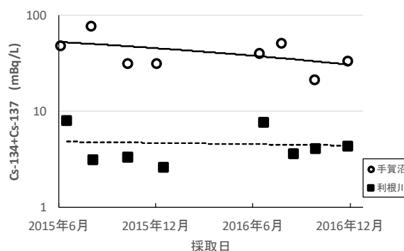
図 2 環境水の放射性セシウム濃度 (2015-2016)
