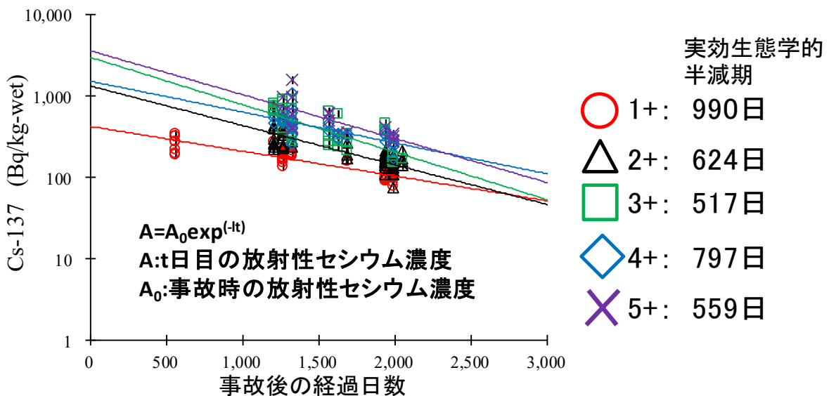
図6 コクチバスの年級群ごとの放射性セシウム濃度の推移
