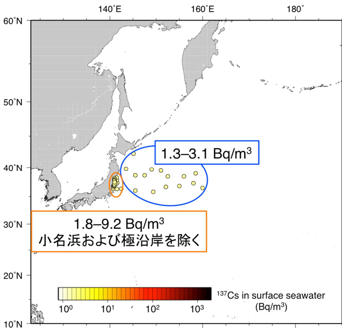
図 4. 2016 年に採取した表面海水の Cs-137 濃度
