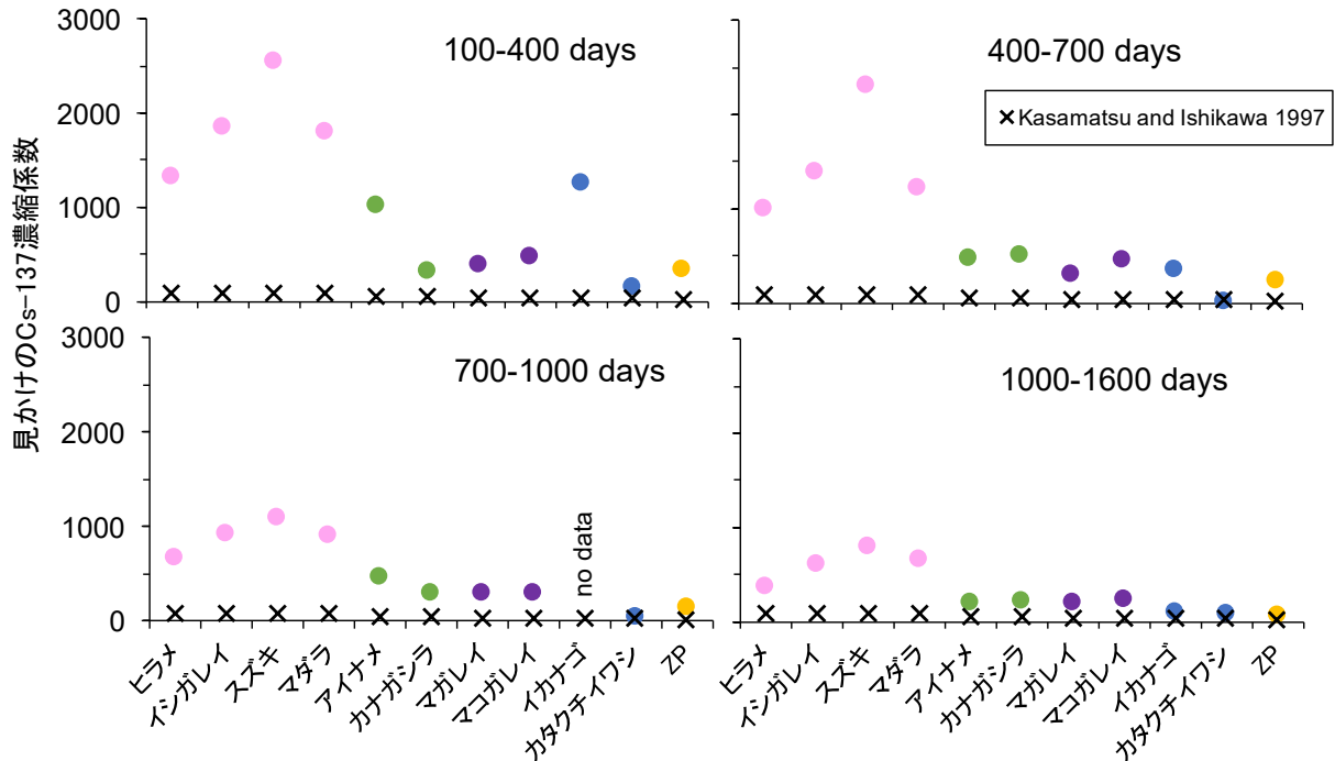
図3 事故後各期間における主要魚類および動物プランクトン (ZP) の見かけの Cs-137 濃縮係数。図内シンボル (X) は、Kasamatsu and Ishikawa (1997) により食性別に算出された事故前の濃縮係数である。シンボルの色は胃内容物観察より区別し、ピンク色は魚食性、緑色は甲殻類食性、紫色はベントス食性および青色はプランクトン食性をそれぞれ表す。また黄色は動物プランクトン (ZP) である。
