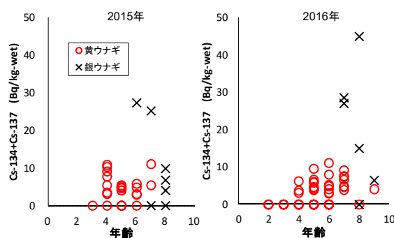
図 4 ウナギの放射性セシウム濃度 (2015-2016 利根川)
