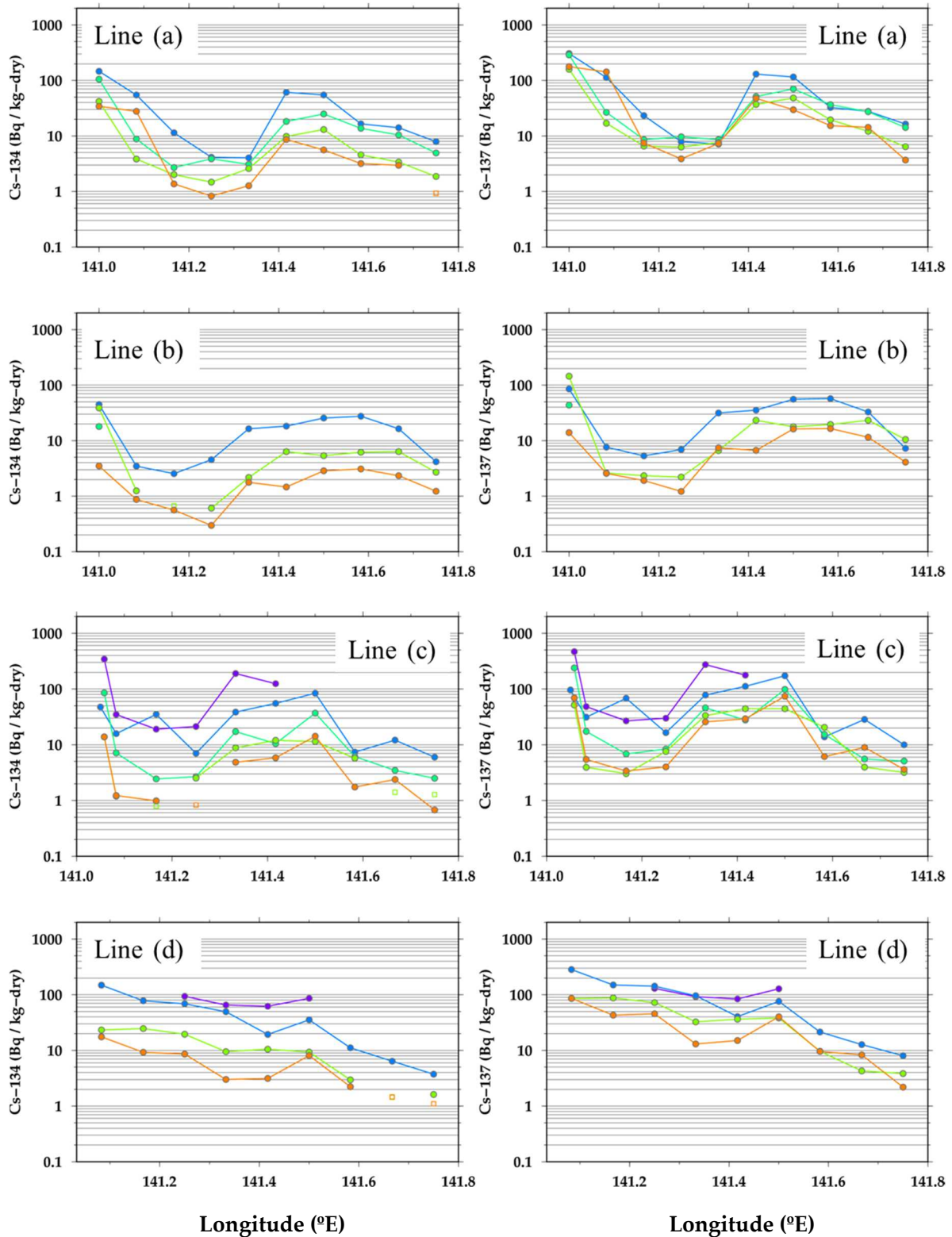
図3. 図1に示したa~hのそれぞれの東西定線における、調査年（右凡例のカラーを参照）ごとの表層海底土中のCs-134（左段）とCs-137（右段）濃度分布。中抜きのプロットの調査点において、海底土中の放射性核種濃度は検出下限値未満であった（プロット値はその検出下限値を示す）。
