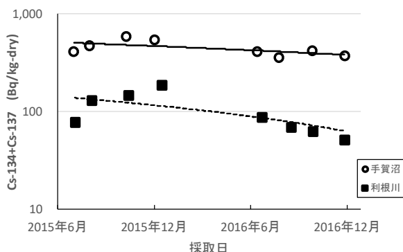
図 3 底泥の放射性セシウム濃度 (2015-2016)
