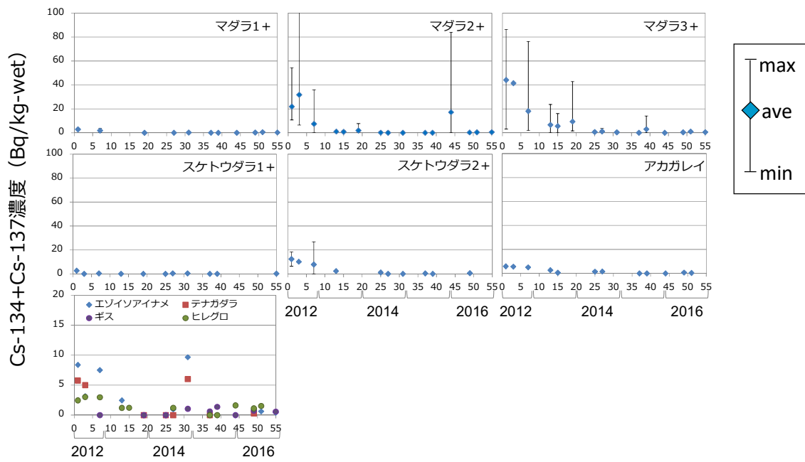
図 3. 大陸棚斜面上部における主要底魚類の放射性セシウム濃度の時系列変化
