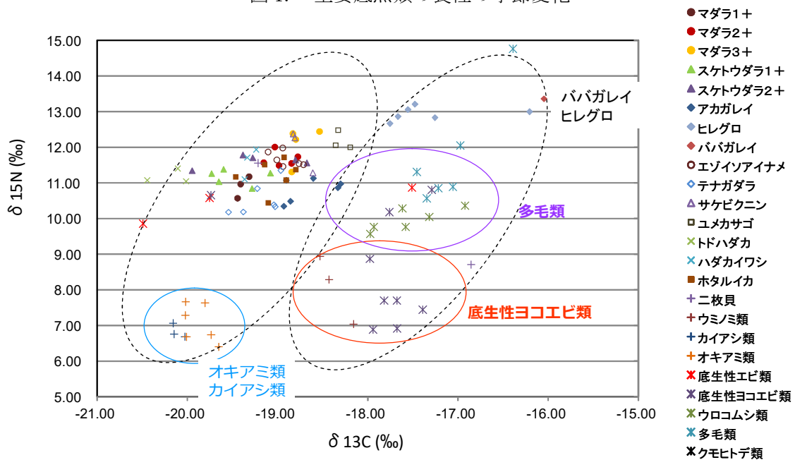
図1. 主要底魚類の食性の季節変化
