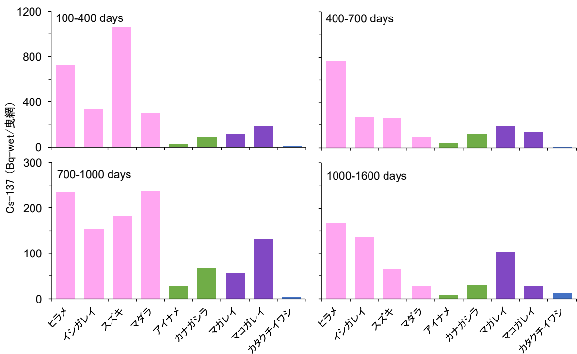
図 5 事故後各期間における曳網あたりのバイオマスで重み付けした Cs-137 量。上段と下段の縦軸は、スケールが異なっている。シンボルの色は胃内容物観察より区別し、ピンク色は魚食性、緑色は甲殻類食性、紫色はベントス食性および青色はプランクトン食性をそれぞれ表す。
