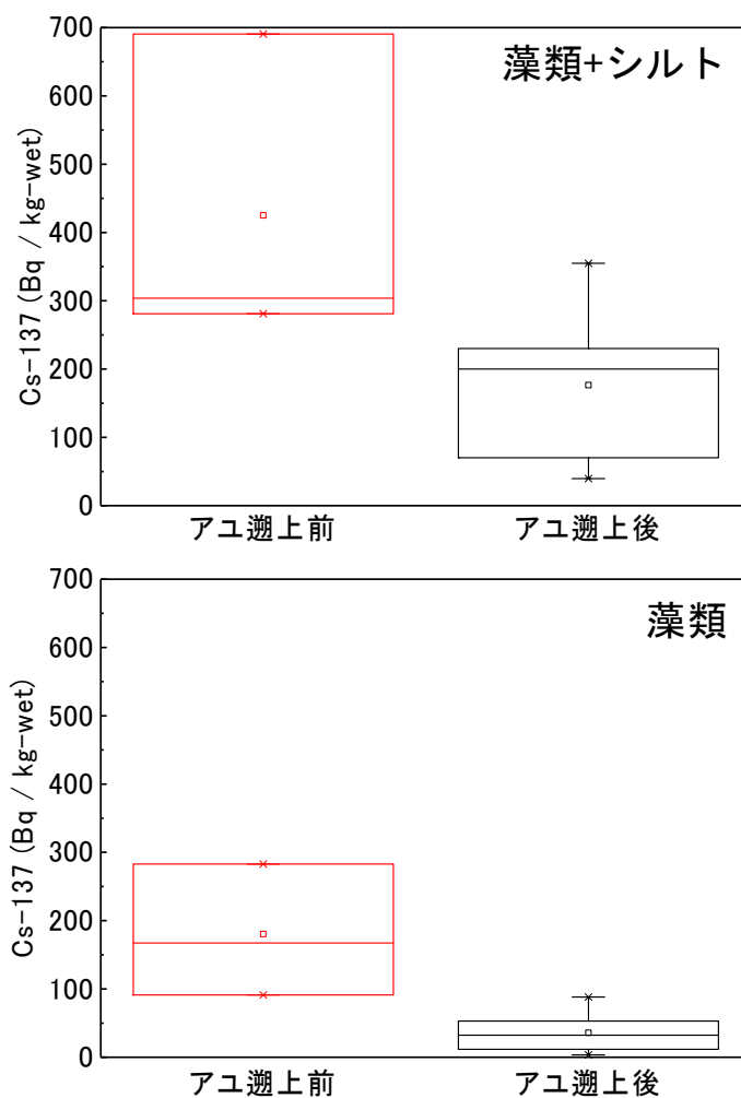
図6 2016年4月（アユ遡上前）、および5, 7, 9月（アユ遡上後）に新田川、木戸川、阿武隈川で採取された底質の付着物（藻類およびシルト、グラフ上段）と付着物からシルトを取り除いた藻類分画（グラフ下段）のCs-137の濃度。エラーバーは95%信頼区間であるが、アユ遡上前は3河川のデータであるため、エラーバーは箱と重複する。
