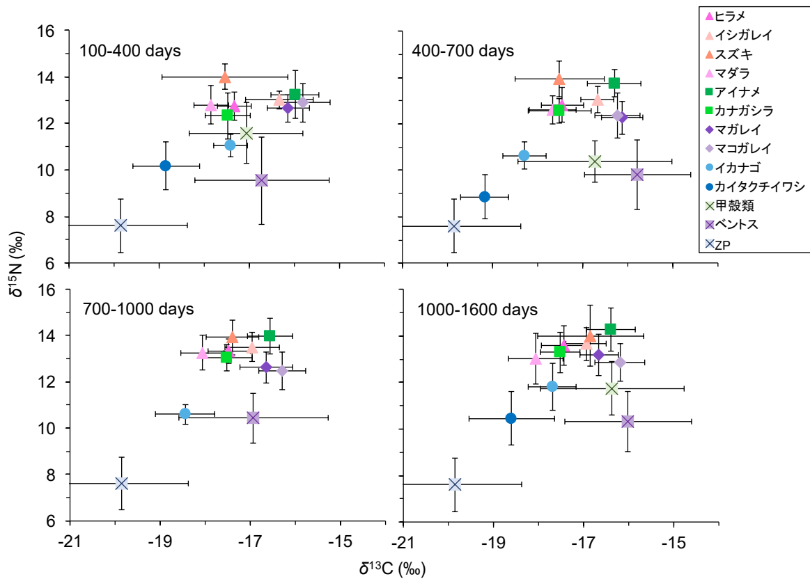
図 4 事故後各期間における炭素・窒素安定同位体比の 2 次元マップ。動物プランクトン (ZP) は、調査期間全体の算術平均値±SD をプロットした。その他生物は、各期間の算術平均値±SD である。
