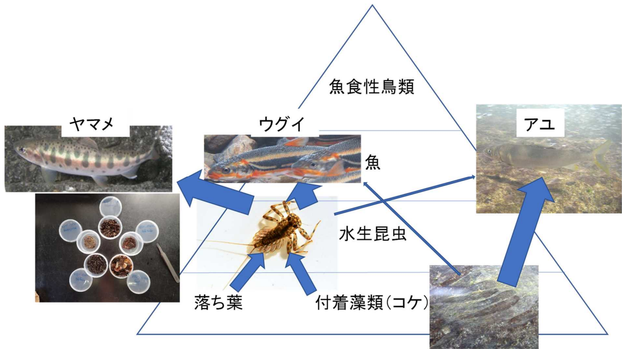
図7 木戸川に生息するアユ、ヤマメ、ウグイの食性調査から明らかになった食物網
