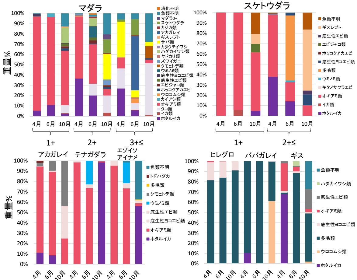
図1. 主要底魚類の食性の季節変化
