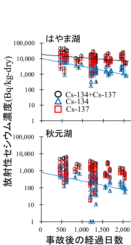
図3 底泥の放射性セシウム濃度の変化
