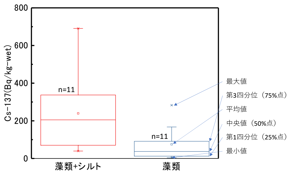
図5 2015年から2016年にかけて新田川、木戸川、阿武隈川、鮫川で採取された底質の付着物（藻類およびシルト）と付着物からシルトを取り除いた藻類分画のCs-137の濃度. エラーバーは95%信頼区間.
