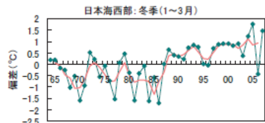
図 2 日本海西部の冬季水温の変化
