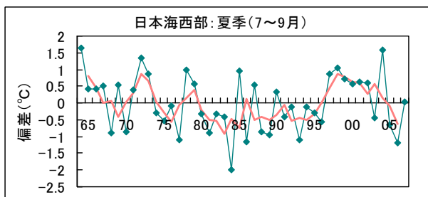
図 日本海西部（ほぼ福井県以西）の冬季と夏季の50m層水温（資料：加藤（日水研））
