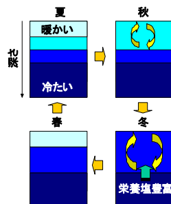
図2. 季節に伴う海洋の上下層の混合と栄養塩取り込みの様子。
