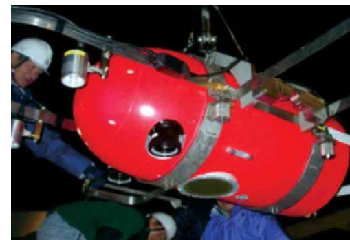
図3 音響・光学複合生物観測システム（J-QUEST）
