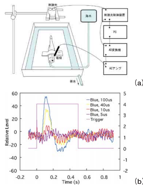
図5 網膜電位測定のための装置の模式図(a)と点灯時間が5、10、40、100 μ秒と異なる青色光の刺激により発生した電気信号(b)
