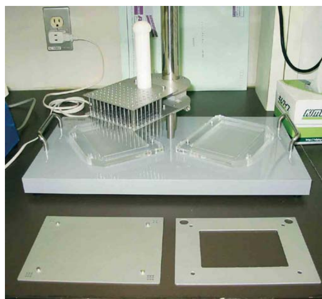
図2 魚介類疾病診断用DNAチップの作製のためのスポッター 手前の鉄板にナイロン膜を挟み、スポッター（奥の台座上）の針をDNAがはいった96穴のマイクロプレート中に浸してから膜に押し付け、DNAをスポットする。
