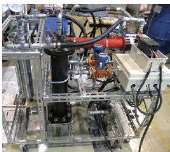
動植物性燃料製造装置
