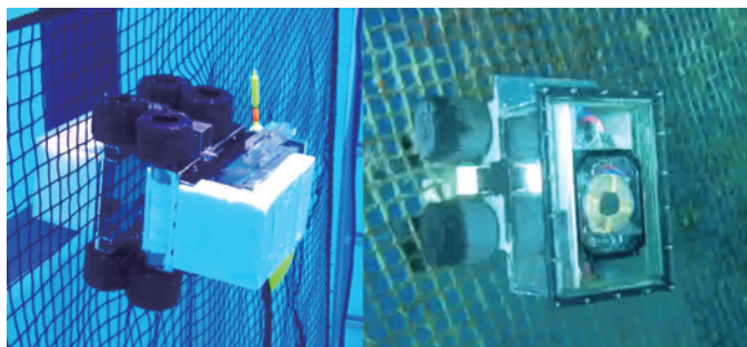
開発中のロボット1号機(左)と2号機(右)
