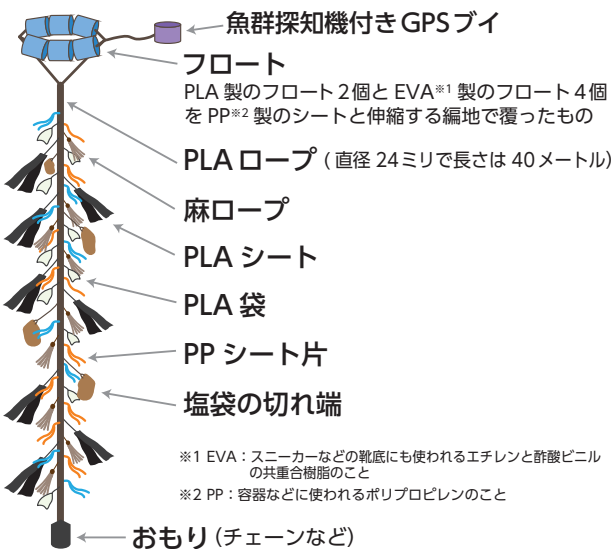
図3 2022年度調査で放流したエコFADs
