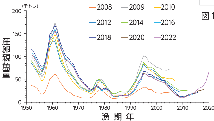
図2 ISCによる過去の太平洋クロマグロ資源評価の比較 凡例の年は資源評価が実施された年で、過去2年前までの資源動態が評価されたもの。
