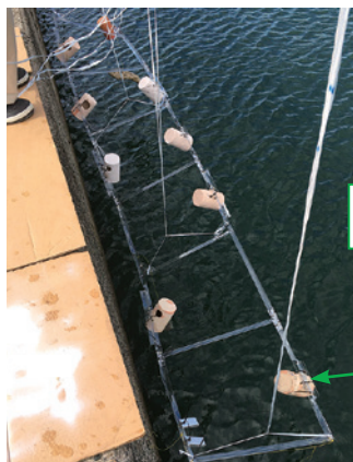
海中への焼成試験体の設置作業のようす
