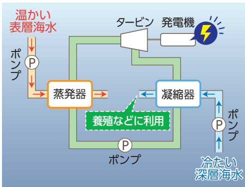
海洋温度差発電システムのイメージ
