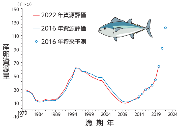
図3 2016年のISCによる将来予測結果と2022年の資源評価結果との比較
