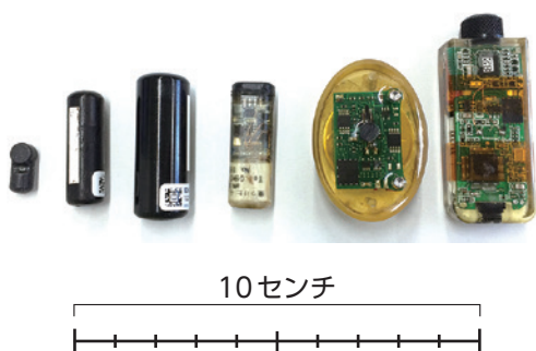
写真 さまざまな発信器・記録計 左3つが超音波発信器（発信型）。 左から4つ目は深度・水温記録計、 5つ目は三軸加速度・深度・水温記録計、6つ目は映像記録計
