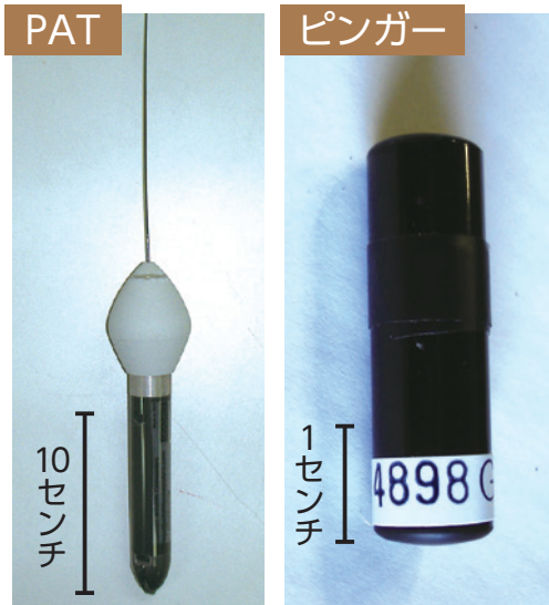
写真3 PATとピンガー
