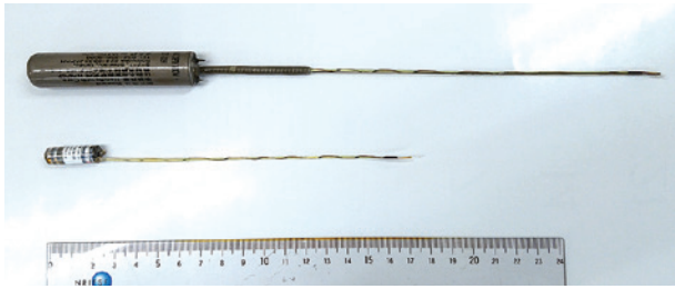
写真1 0歳魚に装着するデータ記録型電子標識（下）と大型魚に装着するデータ記録型電子標識（上）
