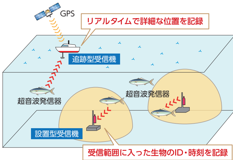
図2 発信型の概念図 受信範囲は追跡型、設置型ともに数百メートルです
