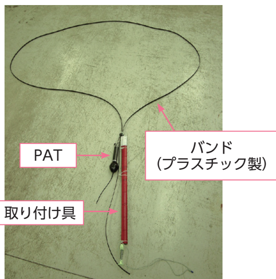
写真4 自作の取り付けバンド
