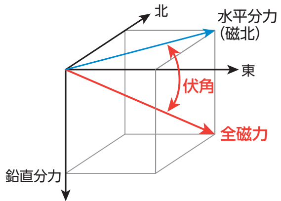
図2 全磁力と伏角の関係
