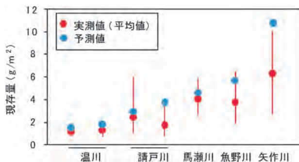
図2. 河川における付着藻類現存量の実測値とモデル予測値の比較。縦線(赤線)の上下端はそれぞれ実測値(n=10)の最大値および最小値を示す。
