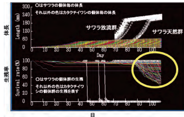
図2 燧灘低次生産モデル+IBM結果例
