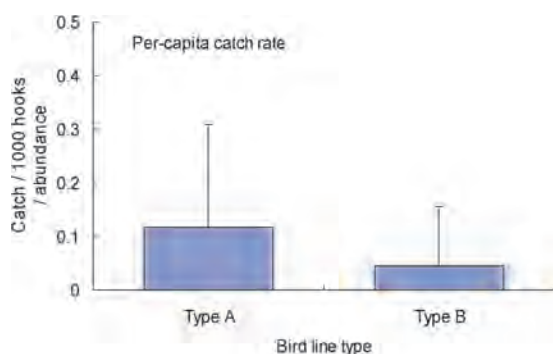
図1. 従来型海鳥混獲回避装置（Type A）と軽量型海鳥混獲回避装置（Type B）の海鳥釣獲率の比較。データの解析は、漁船間の釣獲率の違いを变量効果として取り込んだ、ポアソンGLMMで行った。
