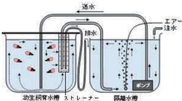
図1. 新たに開発した水流装置
