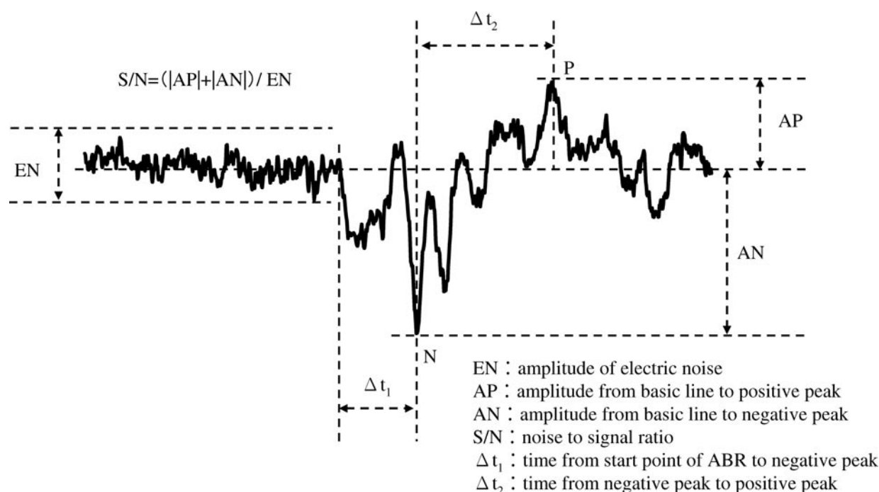
Fig. 3-5. Definition of ABR wave.
