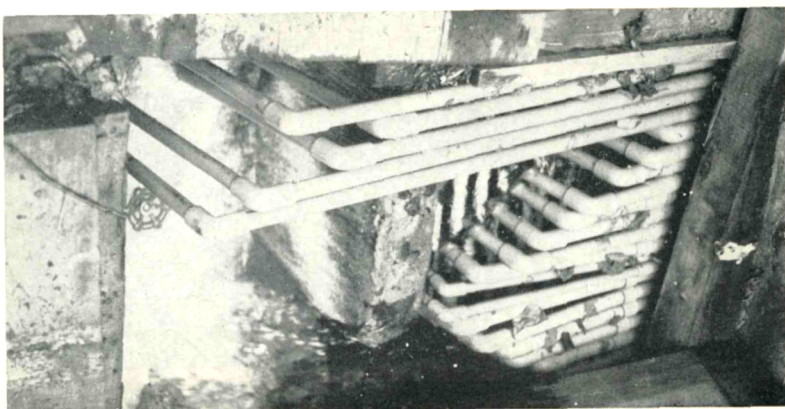
ふ化用水配管 (VP \phi 200mm)
