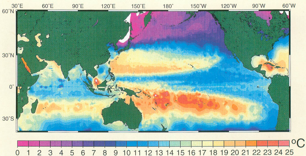
遠洋水産研究所の水温データベース(1964-97年)を用いて描いた太平洋、インド洋の年平均200m深水温図。水温と生息域が密接な関係を持つまぐろ、いか類等の分布域の推定に役立っている。 The distribution of annual mean temperature of 200m depth over the Pacific and Indian Oceans by using NRIFS temperature database (1964-97). It is useful to estimate the habitat of tunas and squids that are widely distributed in these areas and have a close connection with sub-surface temperature.
