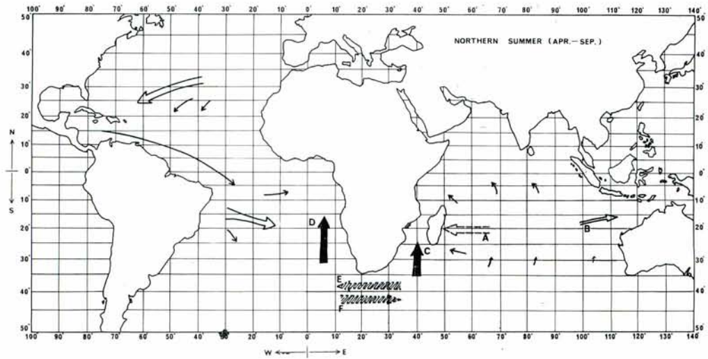
Fig. 4—1 Northern summer
