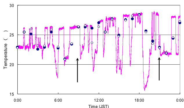
図 MTタグにより記録された水温(紺丸)とタグの記録方式から期待される水温(白抜丸)との比較。
