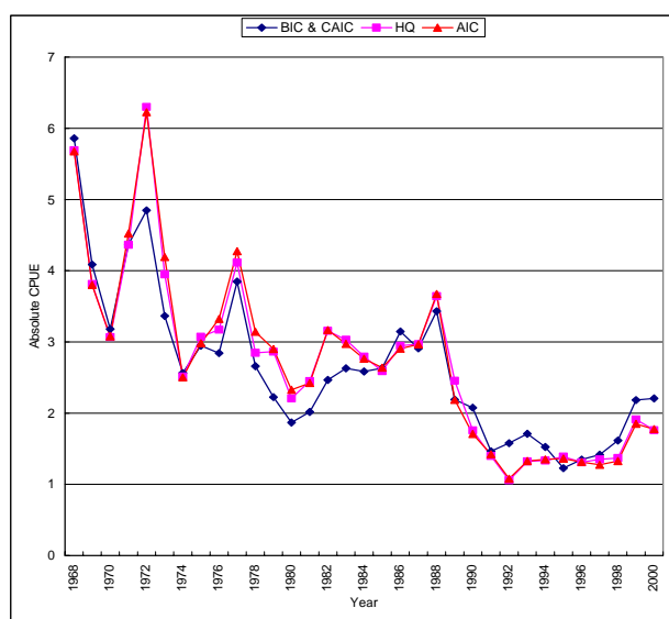
図1 各々の情報量規準(AIC, BIC, CAIC, HQ)により選択されたインド洋におけるキダ資源の標準化 CPUE 年トレンド (Shono,印刷中)
