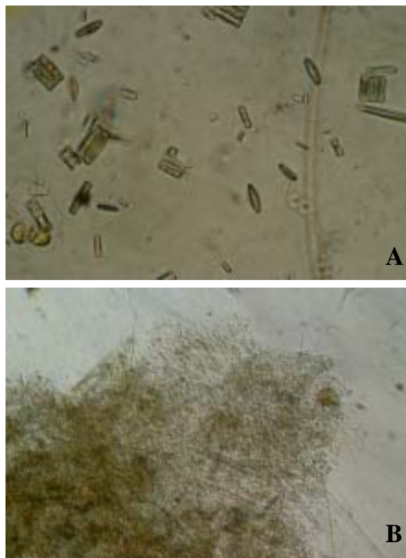
図 2. A: サルパの糞をほぐしたもの。植物プランクトンは破碎されていない。B: オキアミの糞。内容物は破碎され原形をとどめていない。
