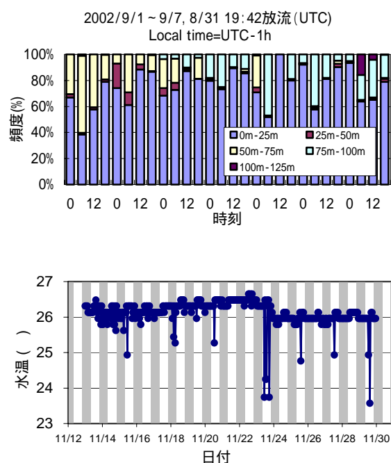
図2. ポップアップタグで得られたニシクロカジキの遊泳水深がWC社、下がMT社製のタグで得られたもの。
