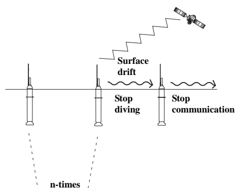
図4. 観測終了時のフロートの制御。一定の回数の観測(4年程度)後に海面に浮上して電波を発信して位置を通報。電池消耗後は海面に漂流する。
