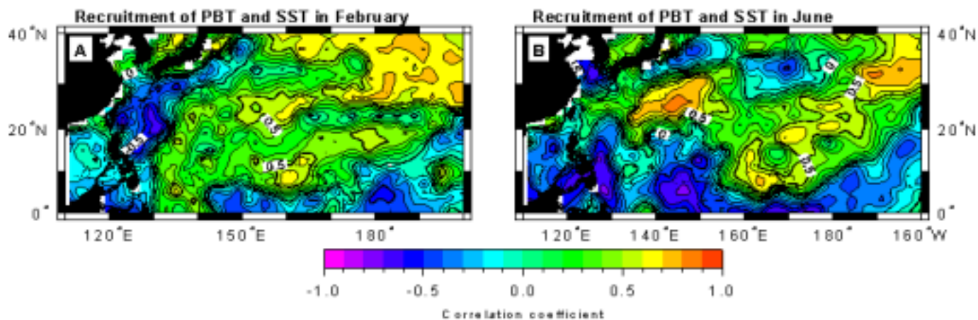
図 4. 太平洋クロマグロ加入量と海面水温 (緯経度 2 度目ごとの時系列データ) との相関係数の水平分布。 A : 2 月, B : 6 月 (主産卵期後期)。琉球列島沖の主産卵場の冬季海面水温と負相関 (青色)、産卵後期 (6 月) には正相関 (黄緑) となる (産卵場が冬季に冷たく、産卵後期に暖かくなる年に加入量が増大する)。越冬場である亜熱帯循環北部域 (北緯 30 度付近) で正相関となる (越冬場が高温であるほど加入量が増大する)。
