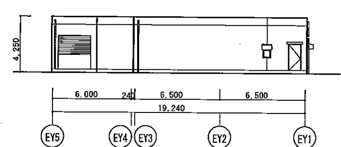
西面立面図
