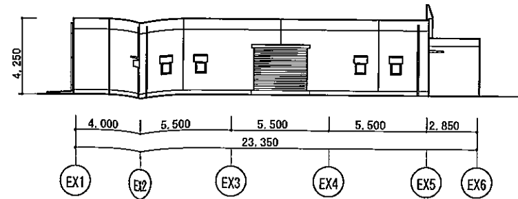
南面立面図
