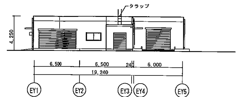
東面立面図
