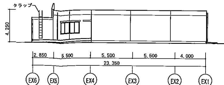
北面立面図
